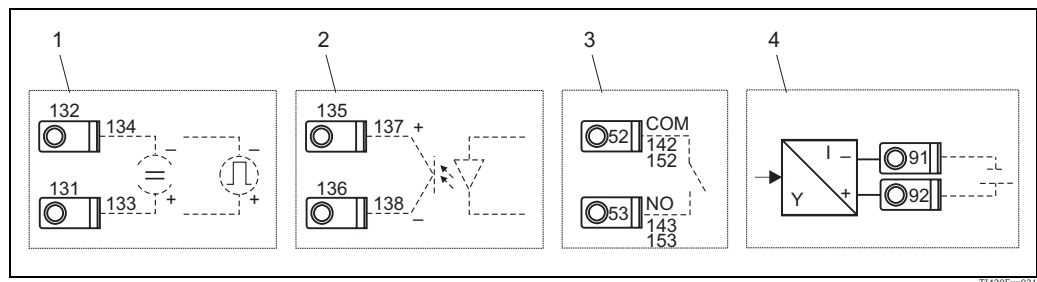
Abb. 17: Anschluss Ausgänge
