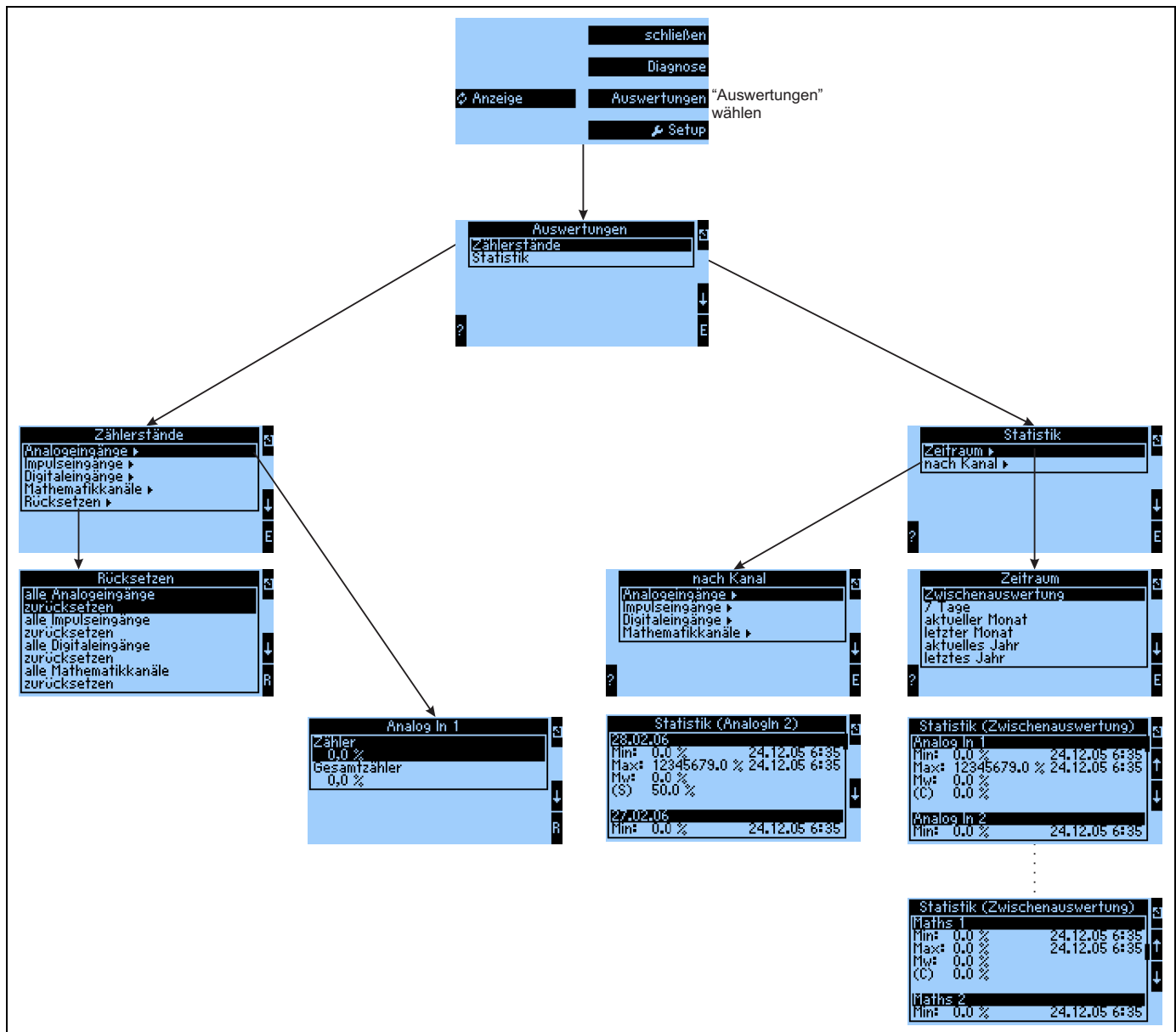
Abb. 35: Parametrierung der Statistik FML621
