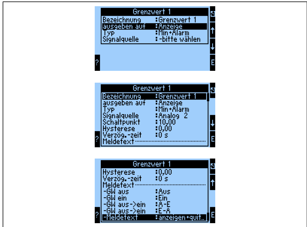
Abb. 49: Parametrierung der Grenzwerte
