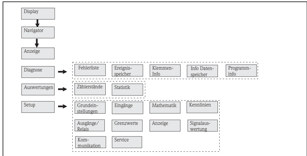
Abb. 33: Funktionsmatrix (Auszug) für die Vor-Ort-Parametrierung des Dichterechners. Eine ausführliche Funktionsmatrix ist im Anhang zu finden.
