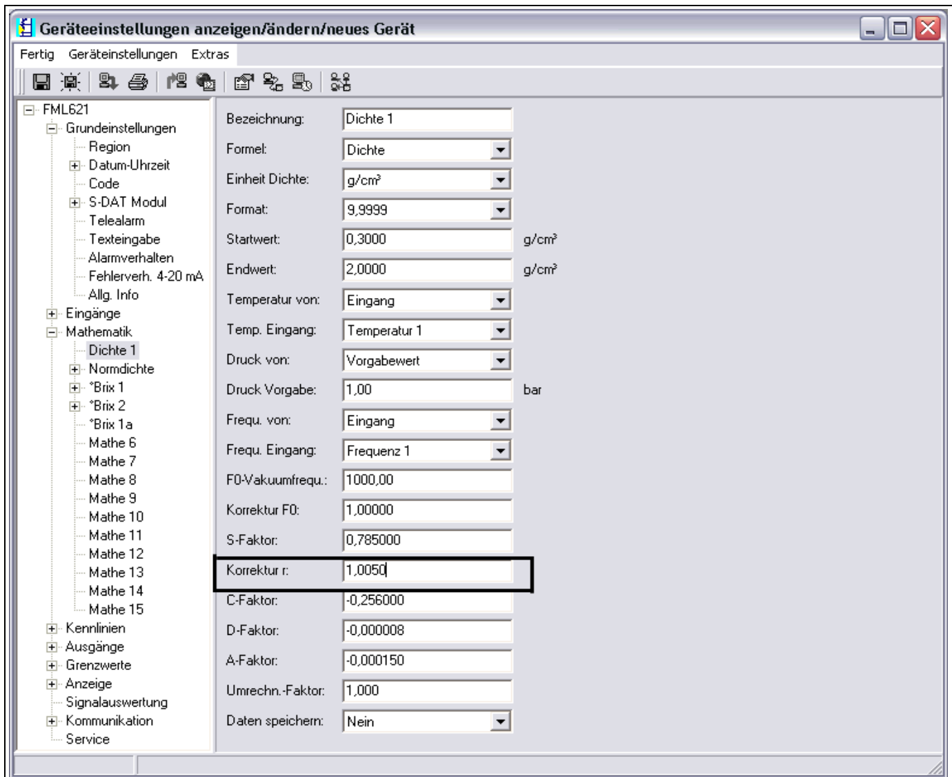
Abb. 12: Eingabefeld für den Korrekturfaktor (Korrektur r)
