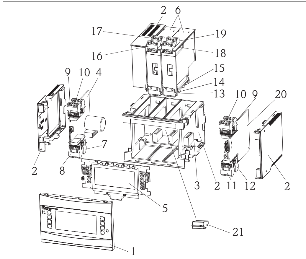
Abb. 70: Ersatzteile FML621
