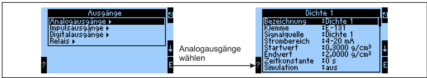
Abb. 45: Parametrierung des Analogausgangs
