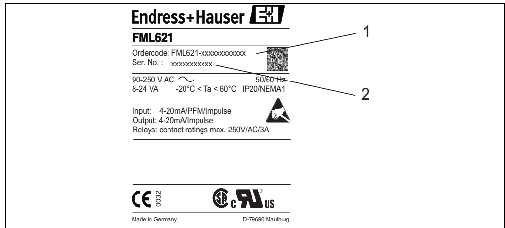
Abb. 1: Typenschild FML621
