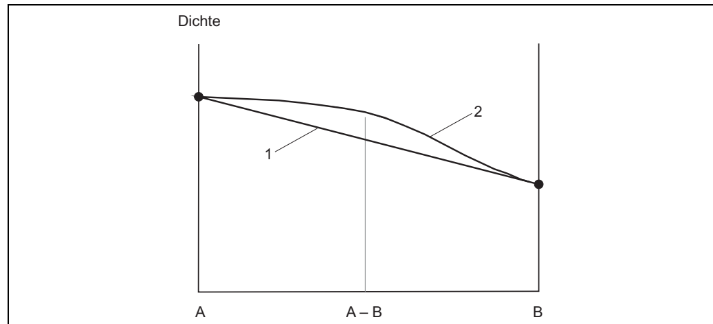
Abb. 65: Zwei Flüssigkeiten A und B bilden ein Assoziat A-B (Kurve 2)
