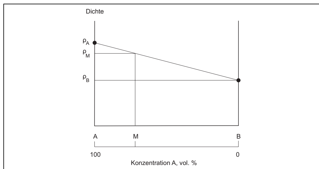
Abb. 66: Bestimmung der vol. Konzentration mittels der Dichte
