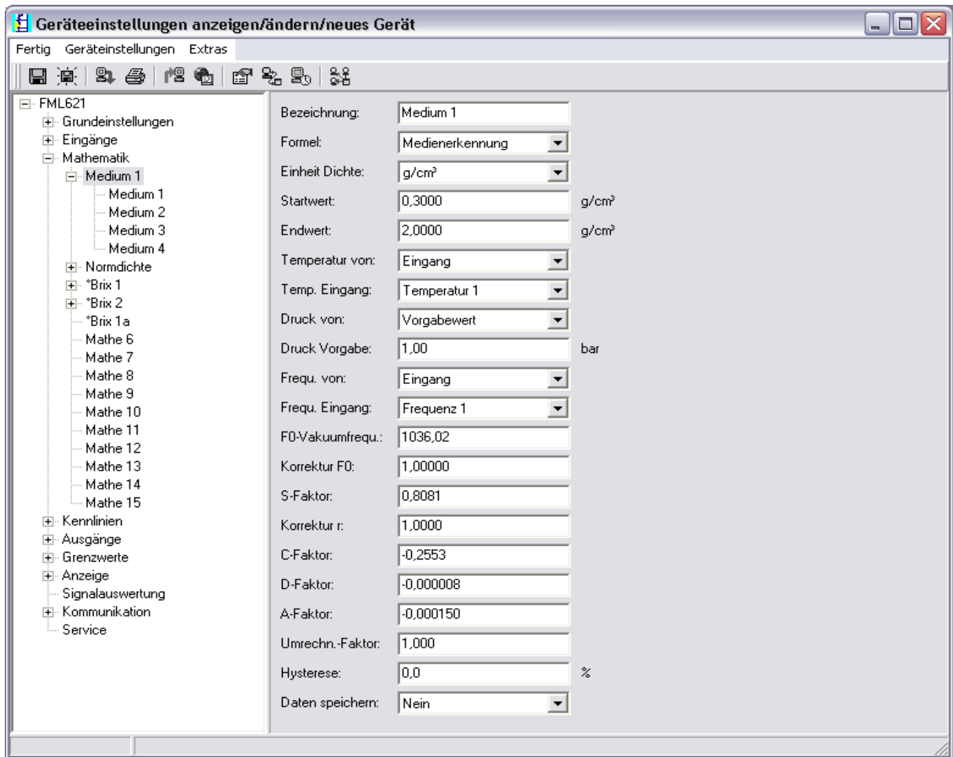
Abb. 69: Mathematik, Formel: Medienerkennung
