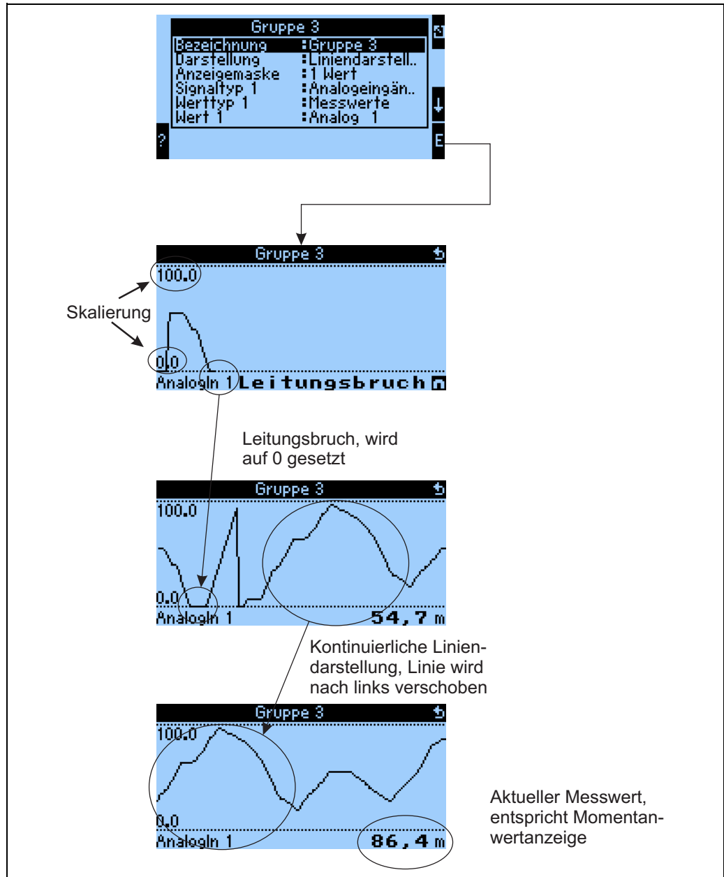
Abb. 39: Liniendarstellung eines Messwertes
