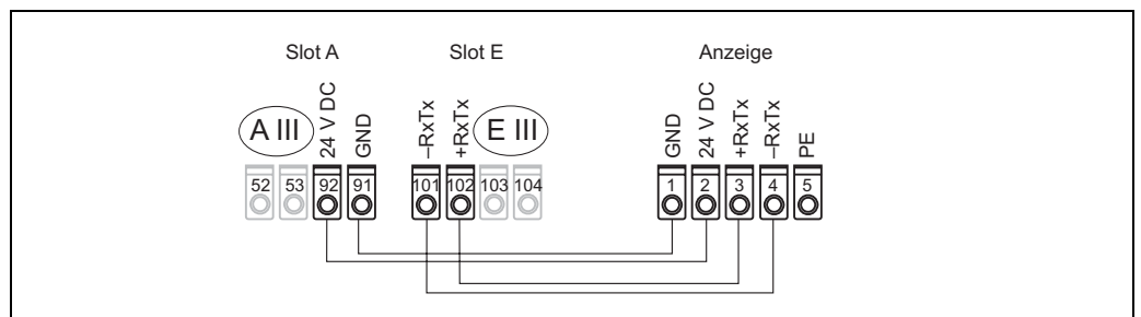
Abb. 23: Klemmenplan abgesetzte Anzeige-/Bedieneinheit
