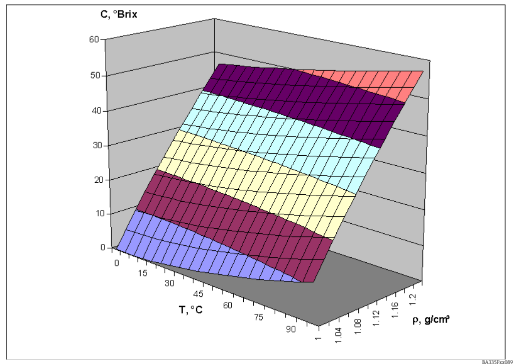
Abb. 67: Konzentration in °Brix als Funktion der Temperatur und der Dichte
