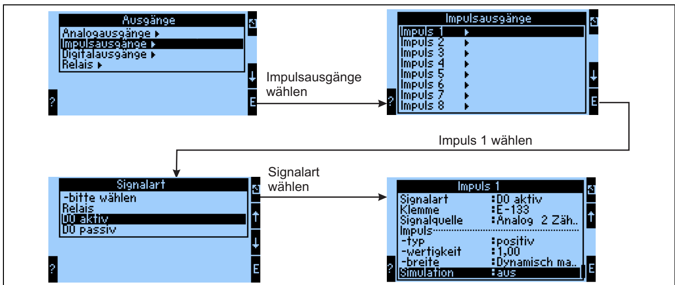
Abb. 46: Parametrierung der Impulsausgänge
