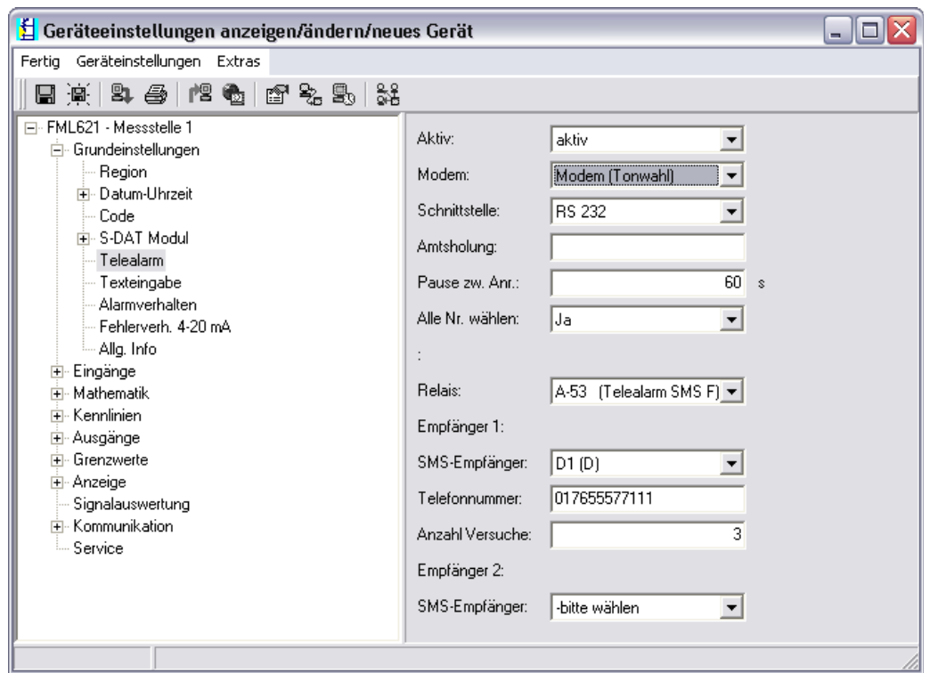
Abb. 52: Parametrierung Telealarm für Modem mit Tonwahl in ReadWin® 2000
