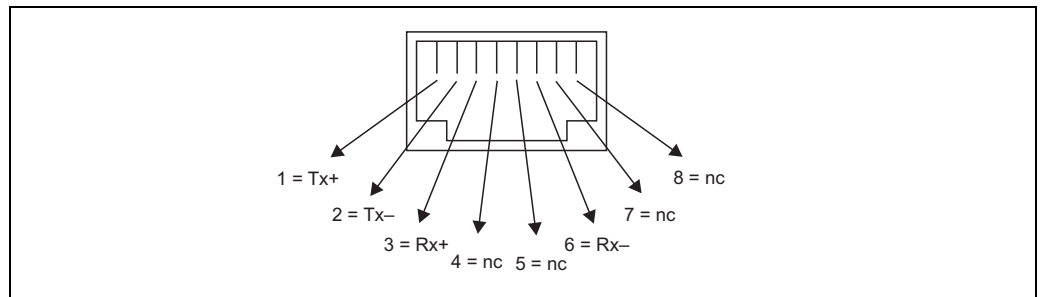
Abb. 19: RJ45-Buchse (Belegung AT&amp;T256)
