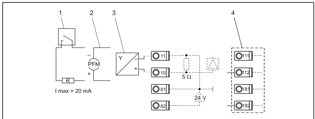
Abb. 16: Anschluss eines aktiven Sensors, z.B. am Eingang 1 (Slot A I).
