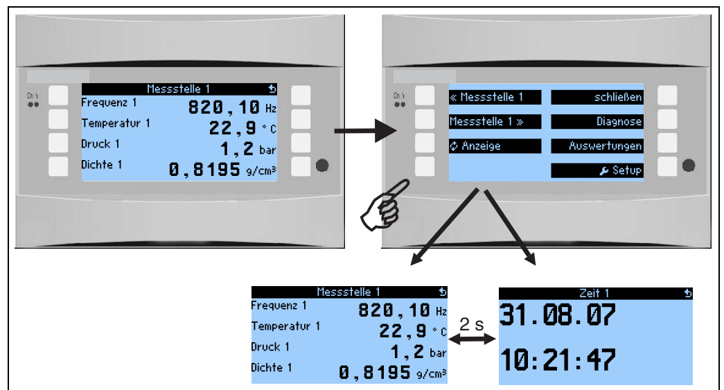
Abb. 37: Automatischer Wechsel verschiedener Anzeigegruppen (alternierende Anzeige)
