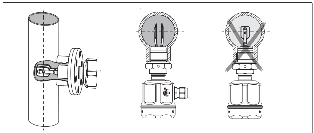
Abb. 8: Ausrichtung der Gabelzinken
