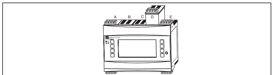
Abb. 72: Gerät mit Erweiterungskarten (optional oder als Zubehör erhältlich) – Steckplätze A und E sind Bestandteile des Grundgerätes – Steckplätze B, C und D sind mit Erweiterungskarten ausbaufähig
