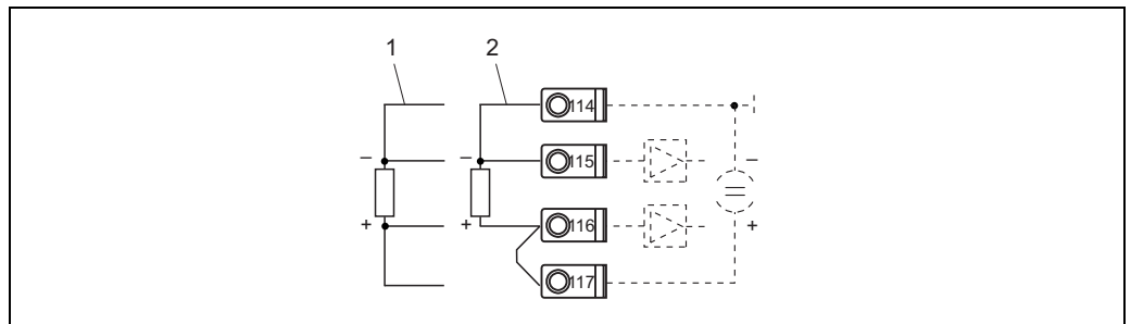
Abb. 21: Anschluss Temperatursensor, optionale Erweiterungskarte Temperatur z.B. in Slot B (Slot B I)
