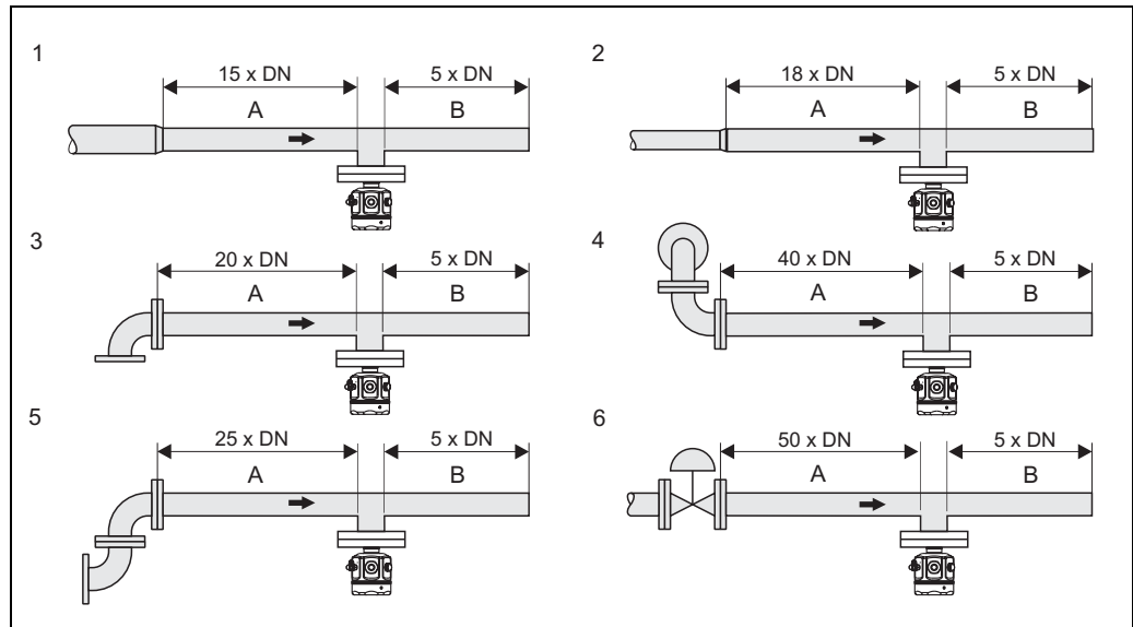
Abb. 5: Minimale Ein- und Auslaufstrecken bei verschiedenen Strömungshindernissen
