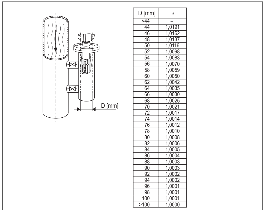
Abb. 10: * Korrekturfaktor (Korrektur r) bei Rohrinnweiten zwischen DN50 und DN100. Eine Korrektur bei Rohrinnweiten > DN100 ist nicht erforderlich.
