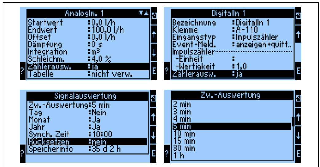
Abb. 50: Parametrierung der Signalauswertung
