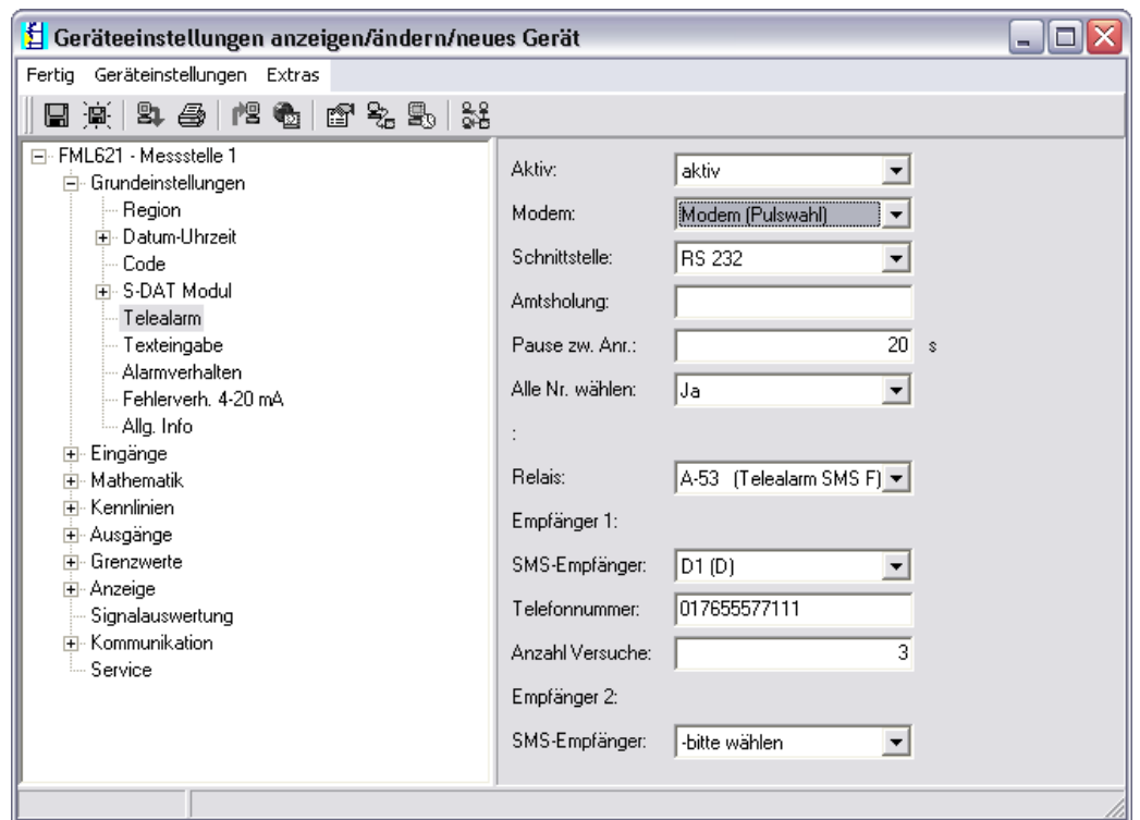
Abb. 53: Parametrierung Telealarm für Modem mit Pulswahl in ReadWin® 2000
