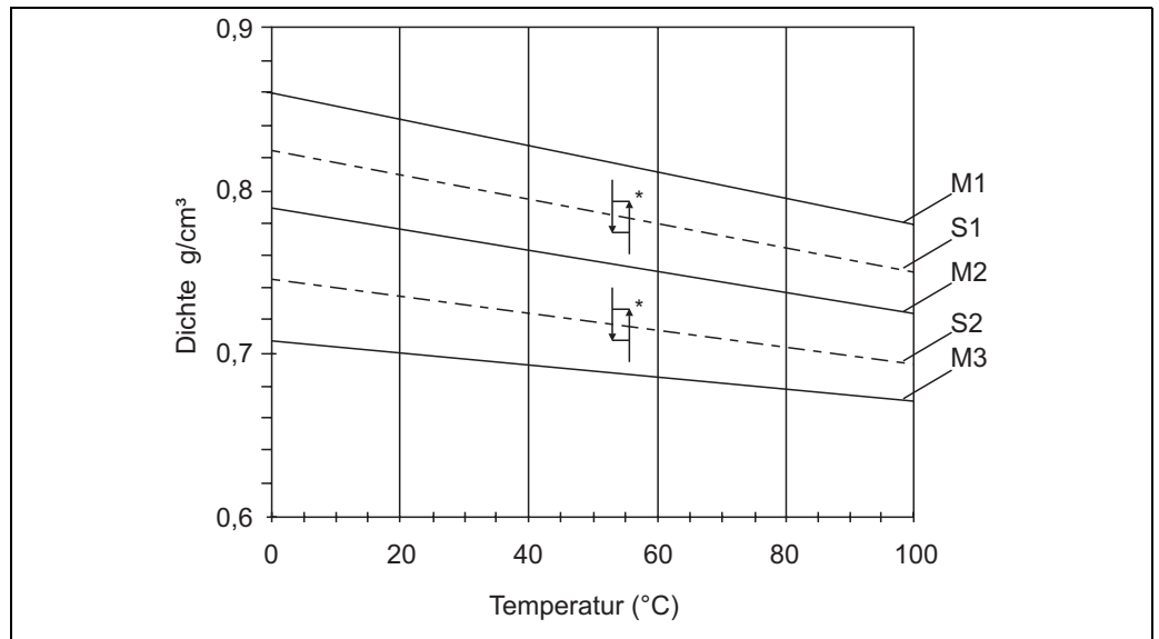
Abb. 68: M1 = Medium1; M2 = Medium2; M3 = Medium3; S1 = Schaltschwelle1; S2 = Schaltschwelle2 * Hysterese in %. Die Hysterese kann z. B. in ReadWin eingegeben werden.
