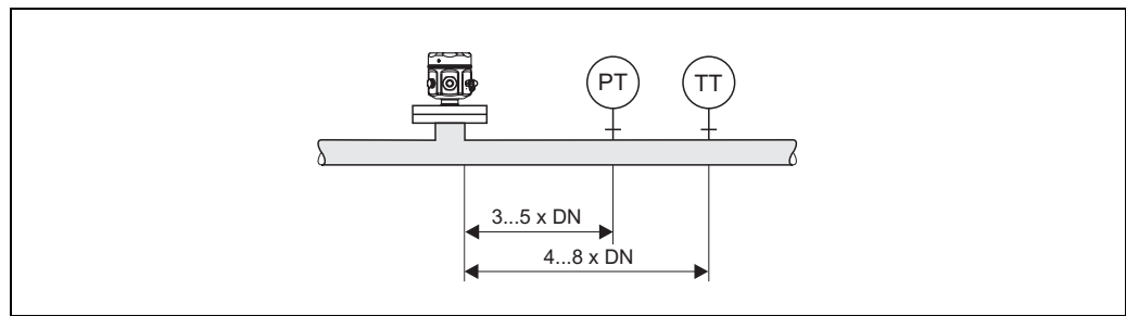
Abb. 6: PT = Druckmessstelle TT = Temperaturmessstelle
