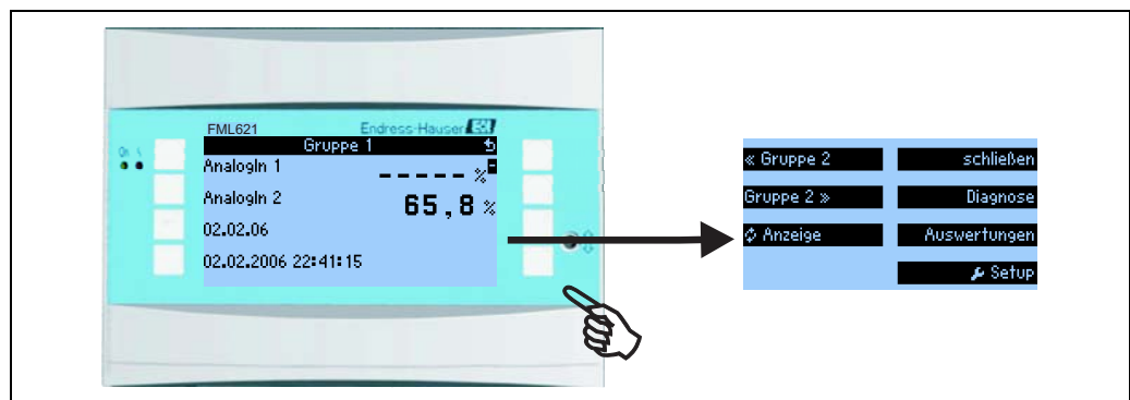
Abb. 34: Schnelleinstieg in die Konfiguration über das Navigatormenü des Dichterechners.
