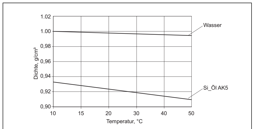
Abb. 62: Temperaturabhängigkeit der Dichte für Wasser und Silikonöl AK5
