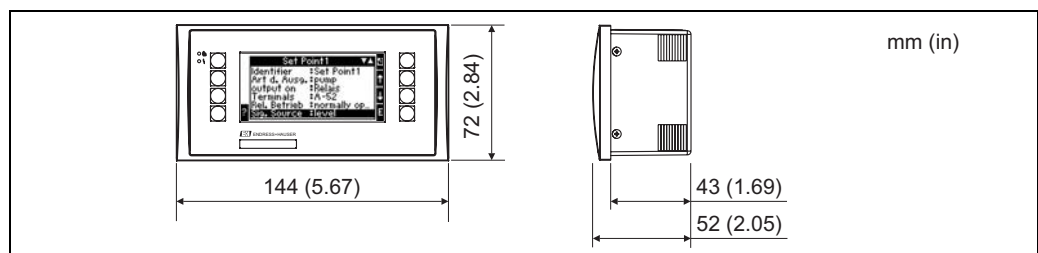
Abb. 73: Bedien-Anzeige-Einheit für Schalttafeleinbau (optional oder als Zubehör erhältlich)
