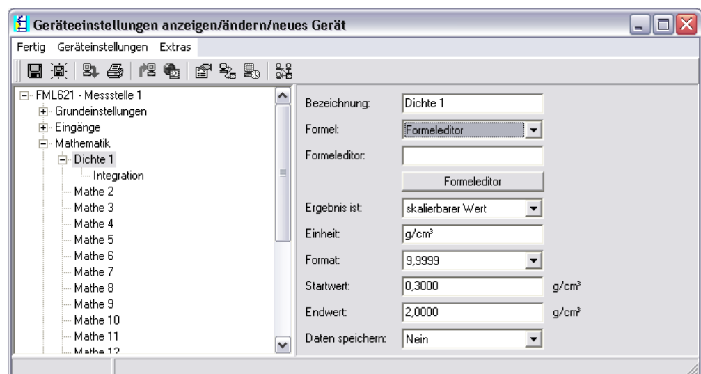
Abb. 60: Formeleditor in der PC-Bediensoftware aufrufen
