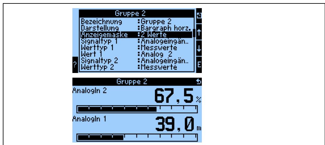
Abb. 40: Zahlenwert + horizontale Balkendarstellung
