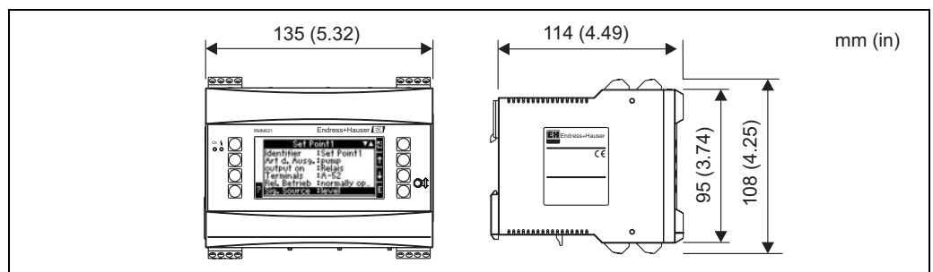
Abb. 71: Gehäuse für Hutschiene nach IEC 60715
