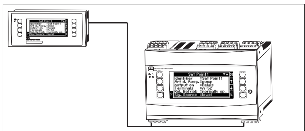
Abb. 74: Bedien-Anzeige-Einheit im Schalttafeleinbaugeschäuse
