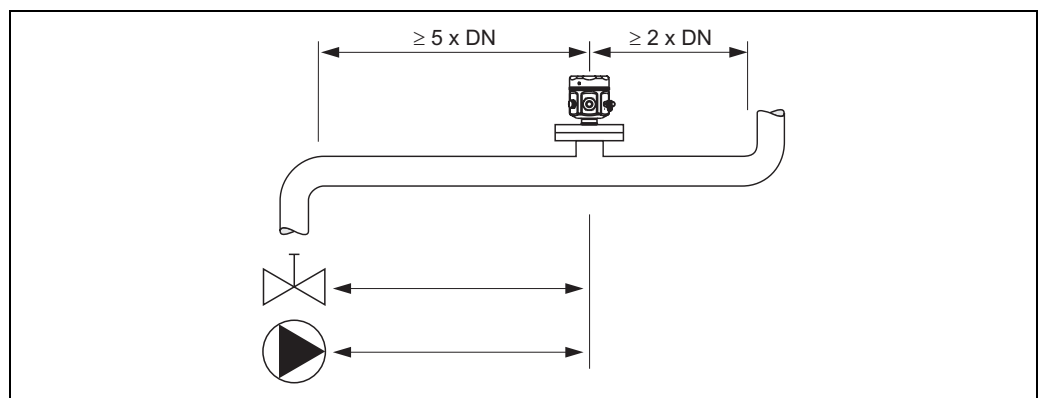
Abb. 4: Ein- und Auslaufstrecken
