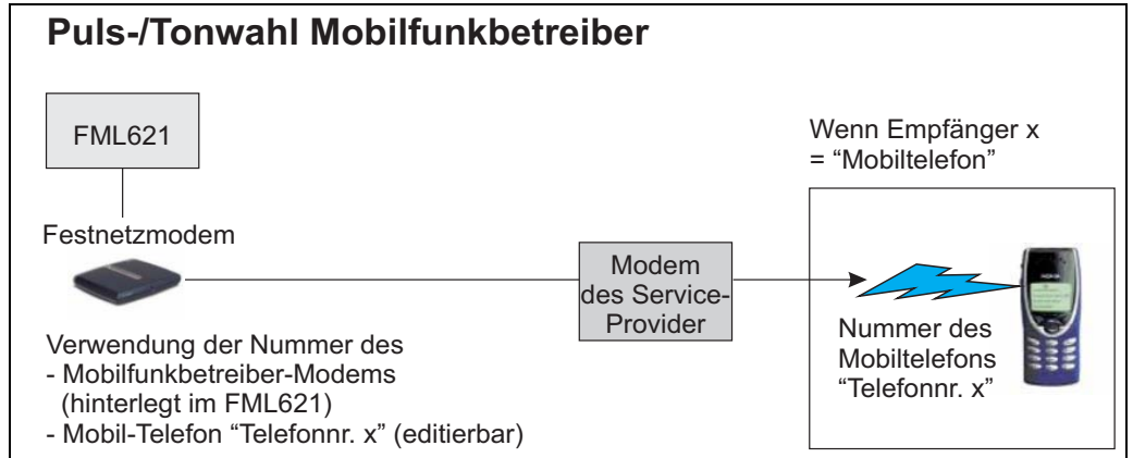
Abb. 56: Kommunikation mit Mobiltelefon (SMS) via Modem des Service-Providers
