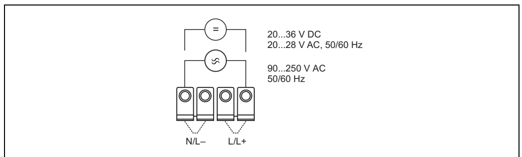
Abb. 14: Anschluss Hilfsenergie
