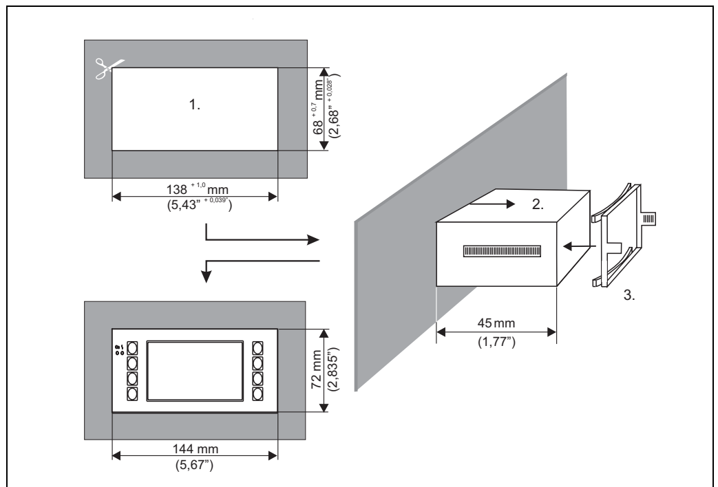
Abb. 22: Schalttafeleinbau
