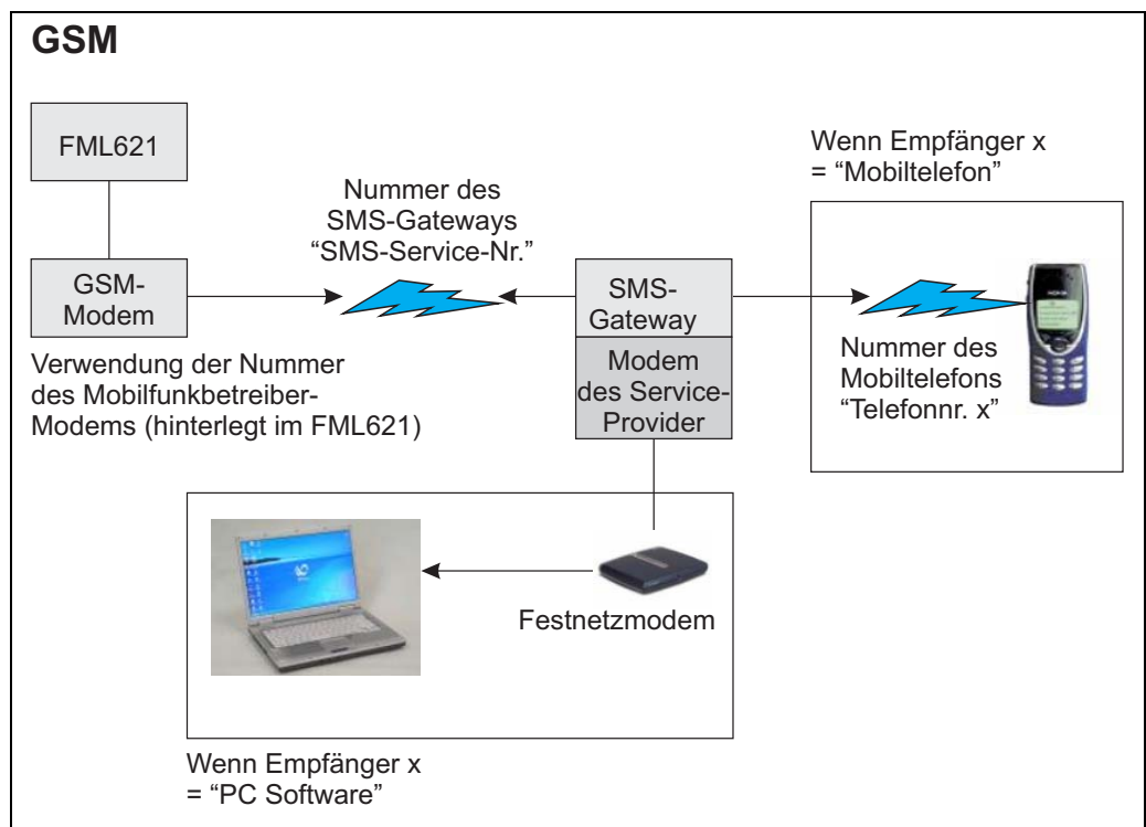
Abb. 55: Kommunikation mit Mobiltelefon (SMS) via GSM-Modem (am FML621) und SMS-Gateway, oder Modem des Service-Providers
