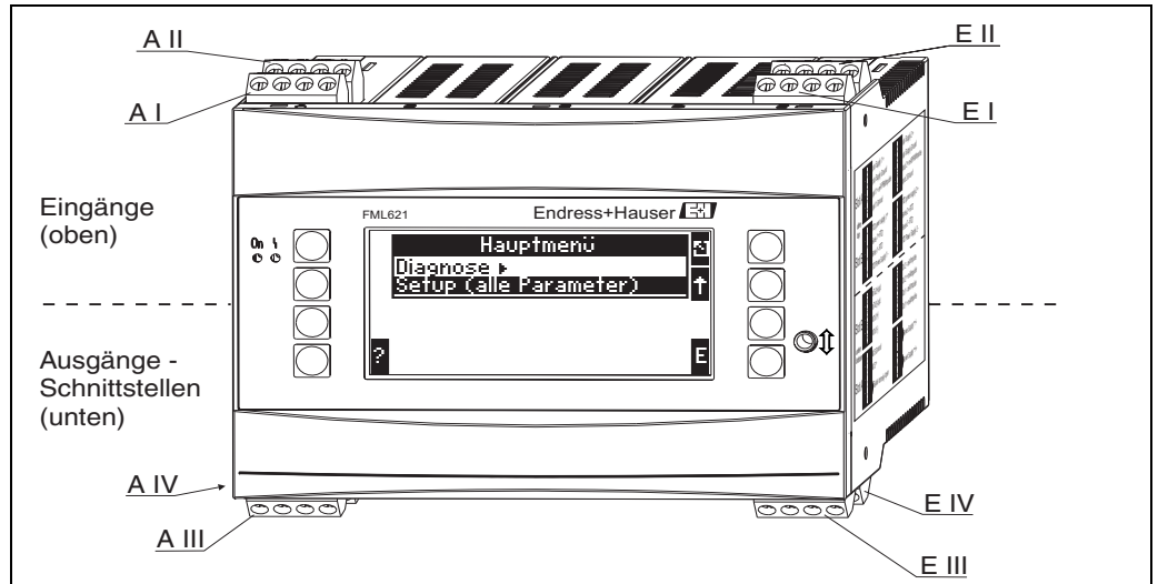
Abb. 13: Slot-Belegung (Grundgerät)
