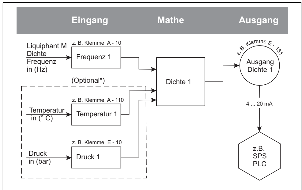
Abb. 32: * wenn die Anwendung es erfordert. Ein Temperatursensor ist erforderlich, wenn eine temperaturkompensierte Dichteinformation benötigt wird. Wenn der Prozessdruck um mehr als +/- 6 bar schwankt, ist ein Drucksensor zur Kompensation notwendig.
