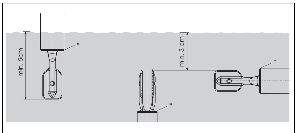
Abb. 11: Gabelzinken und * Membrane müssen vollständig vom Medium bedeckt werden.
