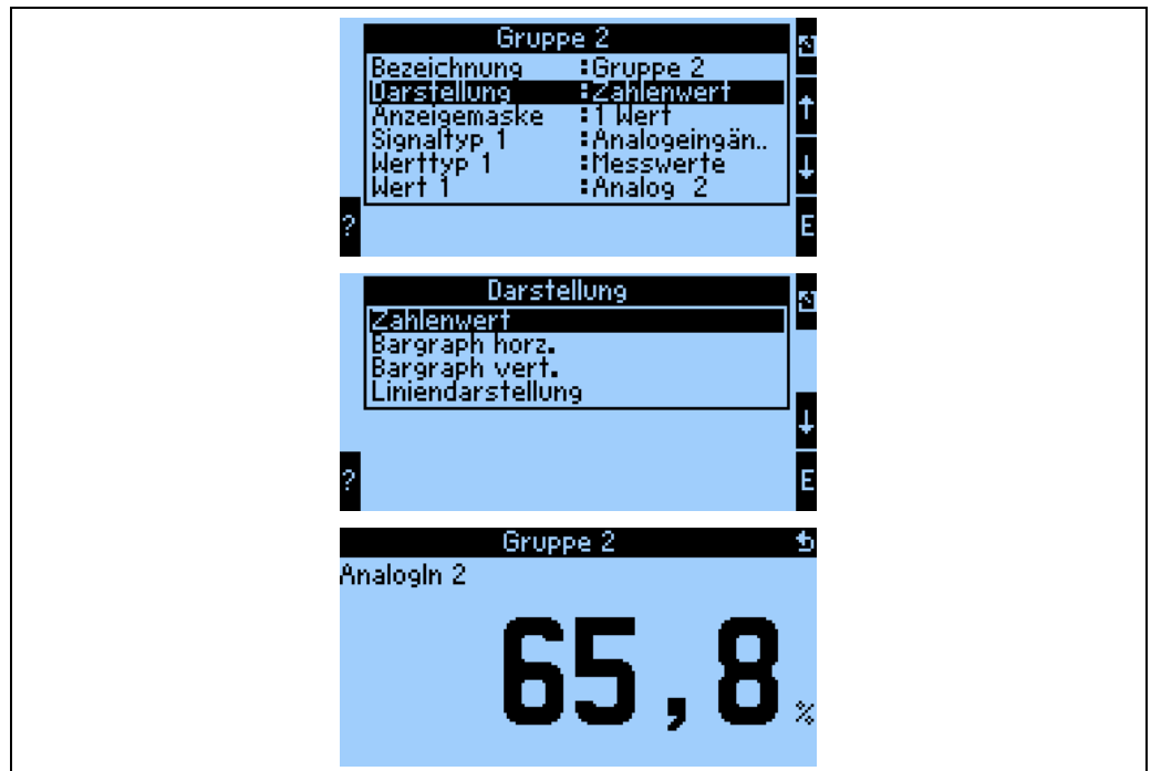
Abb. 38: Darstellung eines Messwertes
