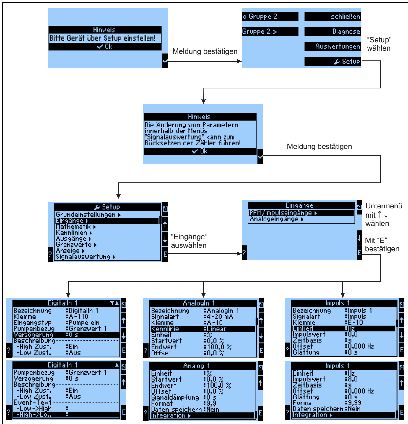
Abb. 44: Parametrierung der Eingänge: Übersicht
