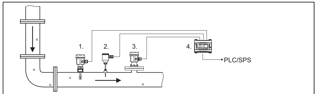
Abb. 31: Szenario für die Messstelle 1
