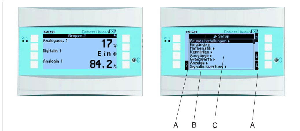
Abb. 25: Anzeigedarstellung des Dichterechners
