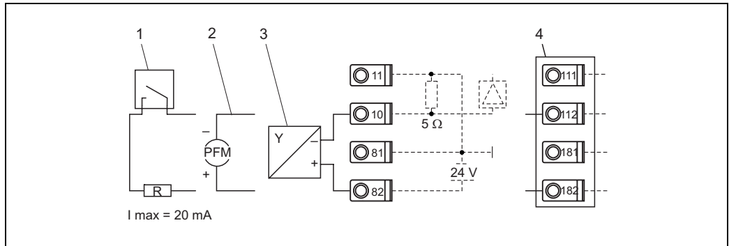
Abb. 15: Anschluss eines passiven Sensors, z.B. am Eingang 1 (Slot A I).
