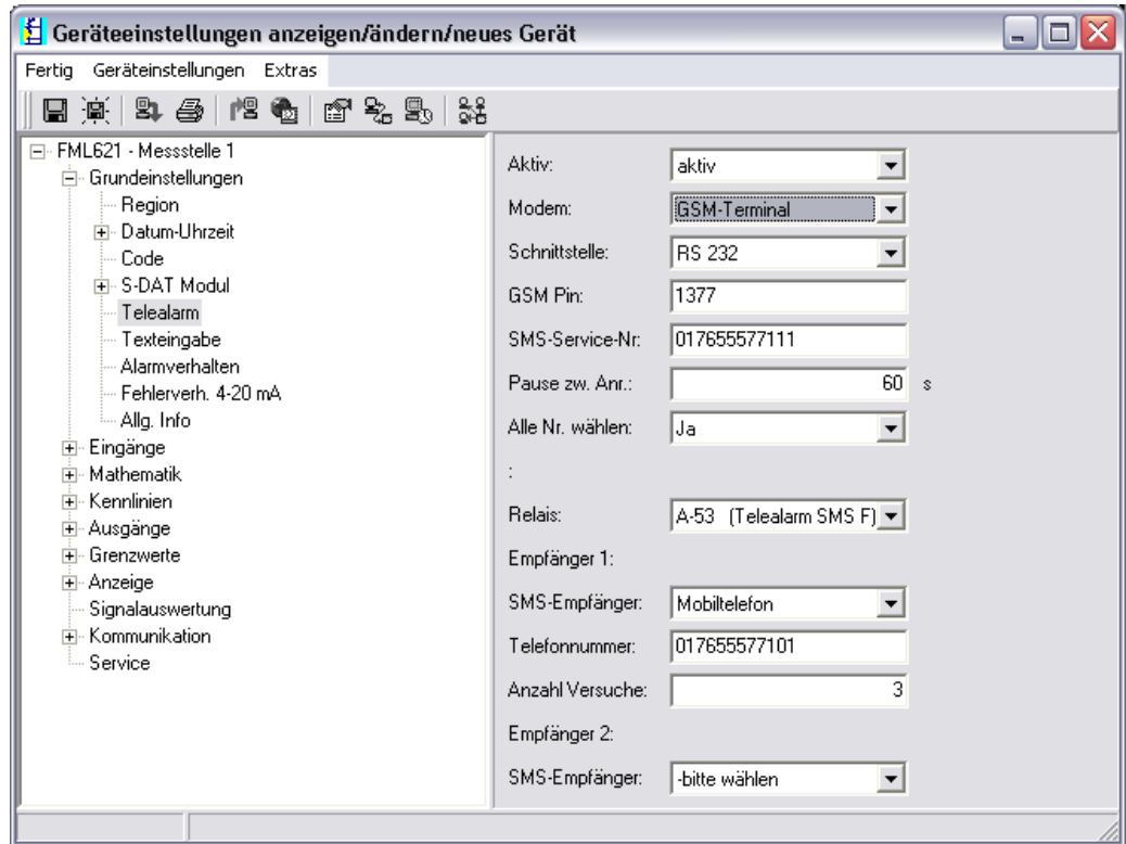
Abb. 54: Parametrierung Telealarm für GSM-Terminal in ReadWin® 2000
