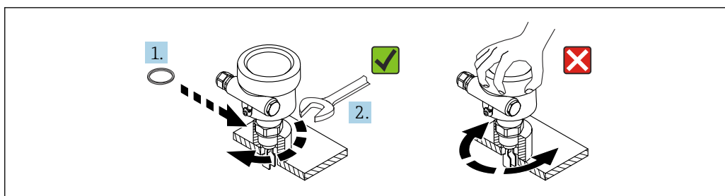
13 Прикручивание прибора
