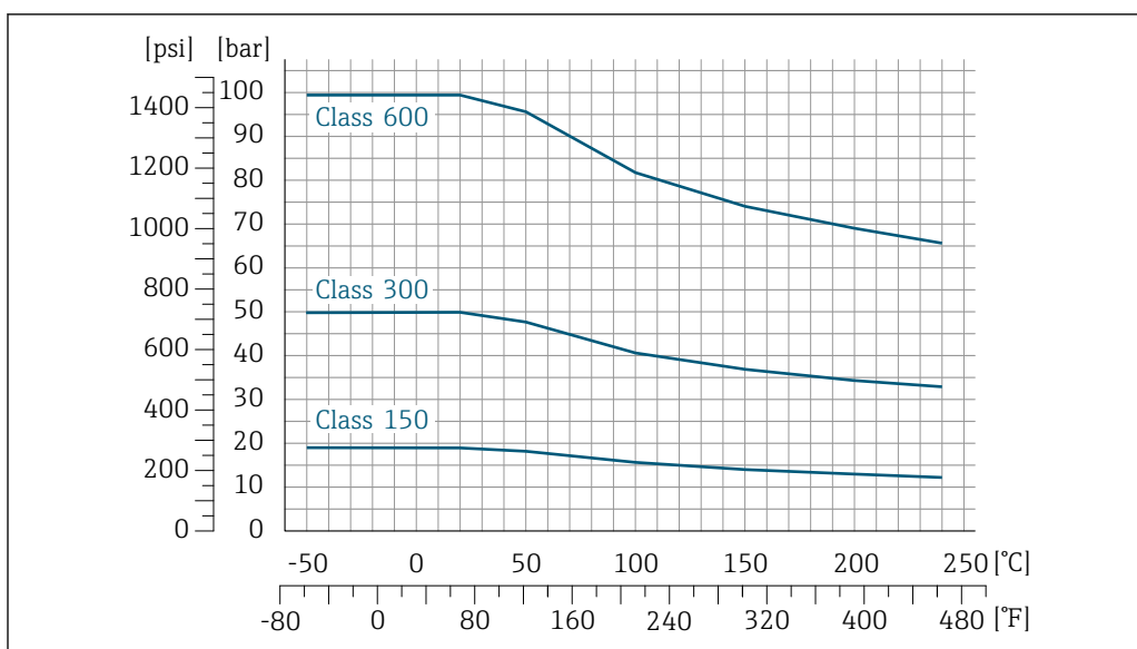
26 Mit Flanschwerkstoff 1.4301 (F304); mediumsberührende Teile Alloy C22
