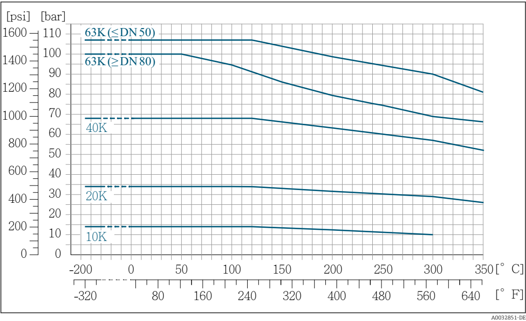
23 Mit Flanschwerkstoff 1.4404 (F316/F316L), Alloy C22
