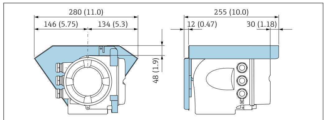
43 Wetterschutzhaube Proline 500; Einheit mm (in)
