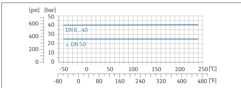
28 Mit Anschlusswerkstoff 1.4404 (316/316L)
