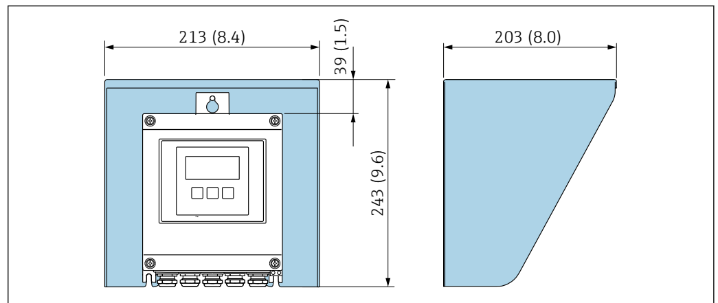
42 Wetterschutzhaube Proline 500 – digital; Einheit mm (in)
