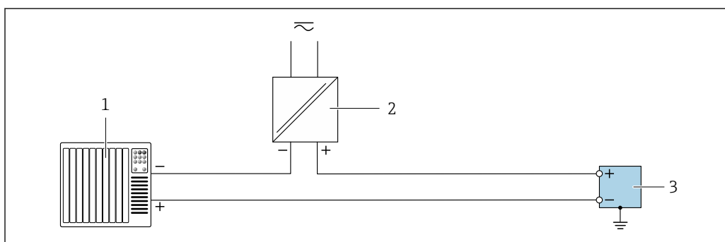
6 Anschlussbeispiel für Impuls-/Frequenz-/Schaltausgang (passiv)
