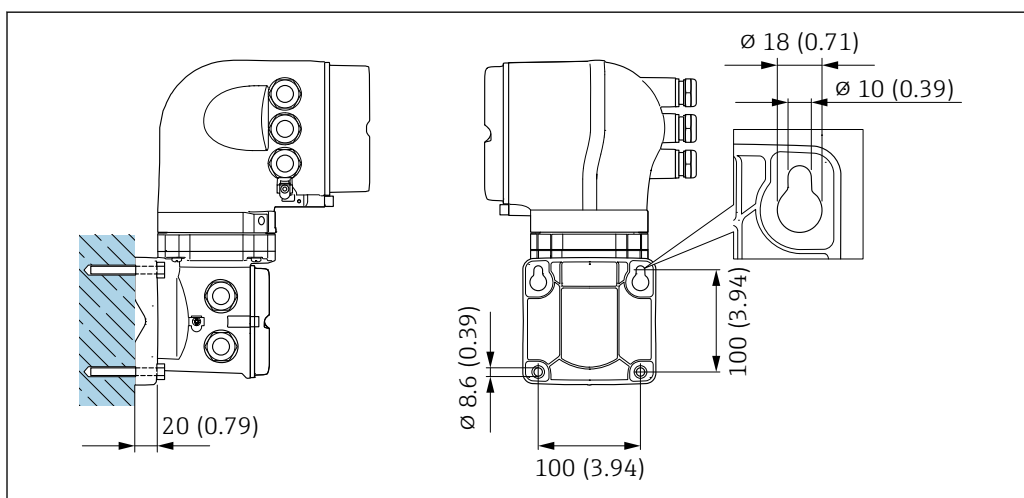
18 Maßeinheit mm (in)
