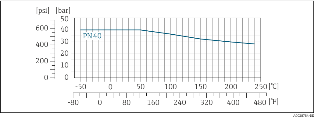
25 Mit Flanschwerkstoff 1.4301 (F304); mediumsberührende Teile Alloy C22
