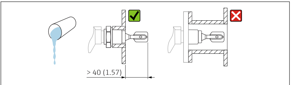
图 7 安装实例：测量高粘度液体介质。测量单位 mm (in)
