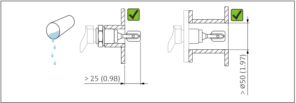
图 6 安装实例：测量低粘度液体介质。测量单位 mm (in)
