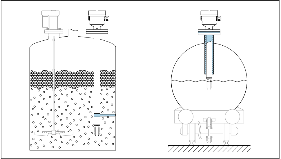
图 10 实例：存在动态负载时，应支撑设备
