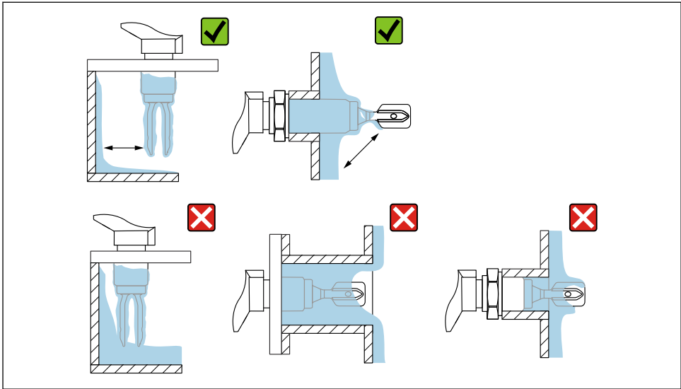
图 8 安装实例：测量高粘度过程介质
