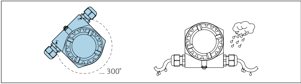
图 15 外壳不带锁紧螺丝；在电缆上建立排水回路
