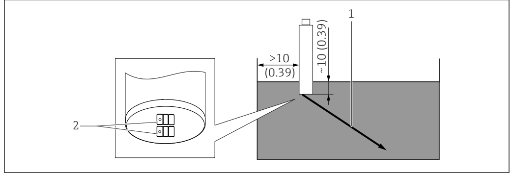
31 Sensörün konumlanması. Boyutlar: mm (inç)
