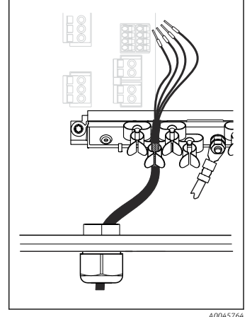
23 Kablunun topraklama kelepçesi içerisine bastırılması
