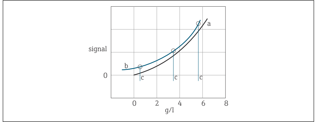
28 Üç noktalı kalibrasyon
