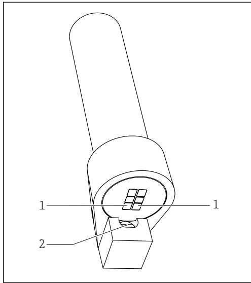
18 Temizlik ünitesinin hizalanması
