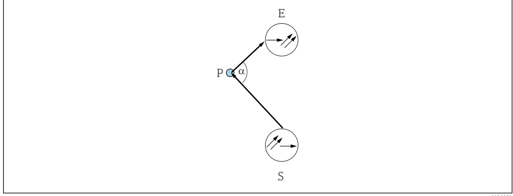
6 90° saçılmış ışık yöntemi
