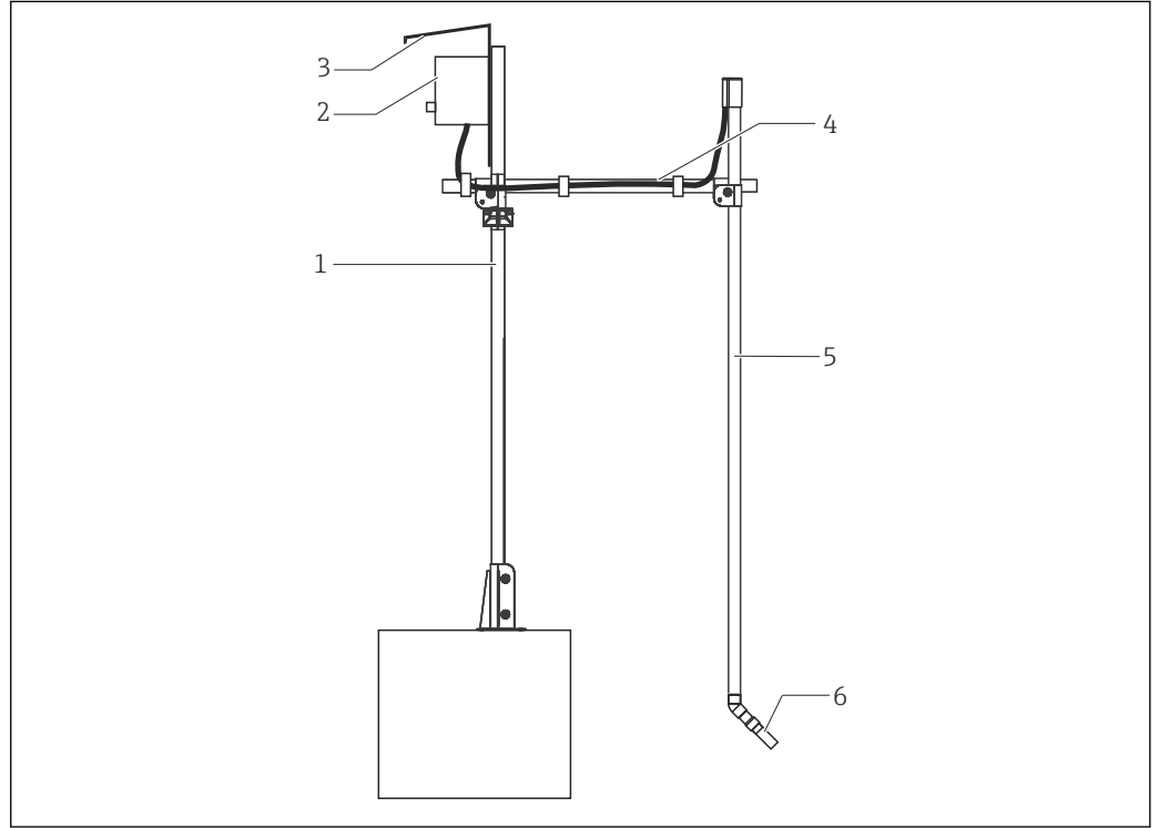
10 Daldırma düzeneğine sahip ölçüm sistemi (örnek)
