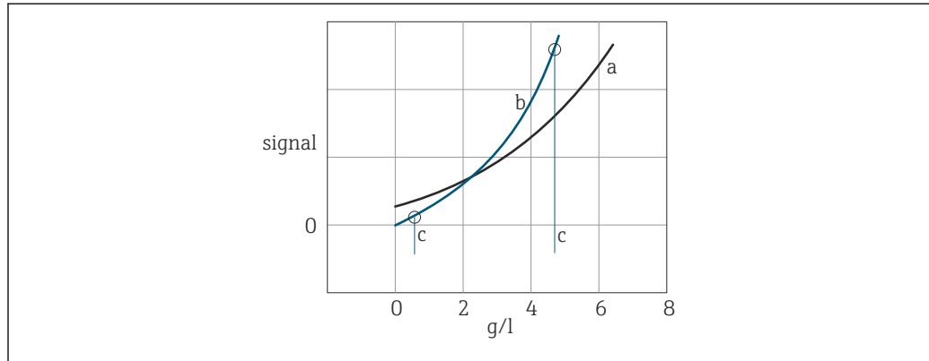
27 İki noktalı kalibrasyon
