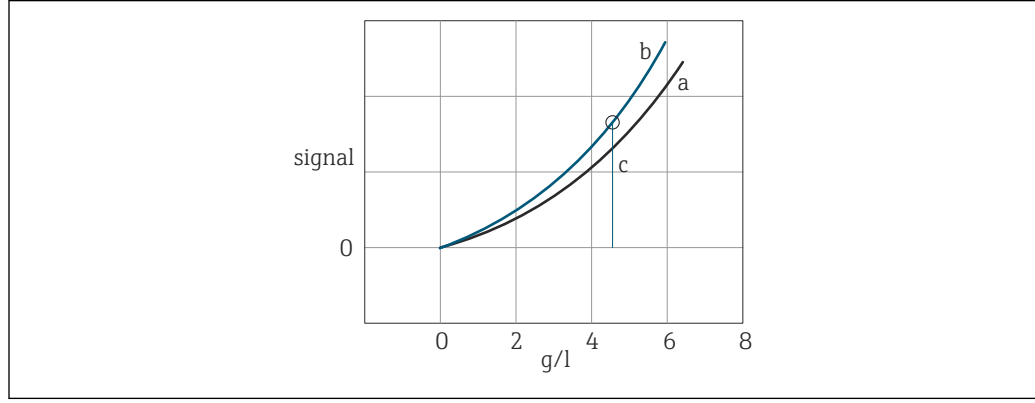
26 Tek noktalı kalibrasyon
