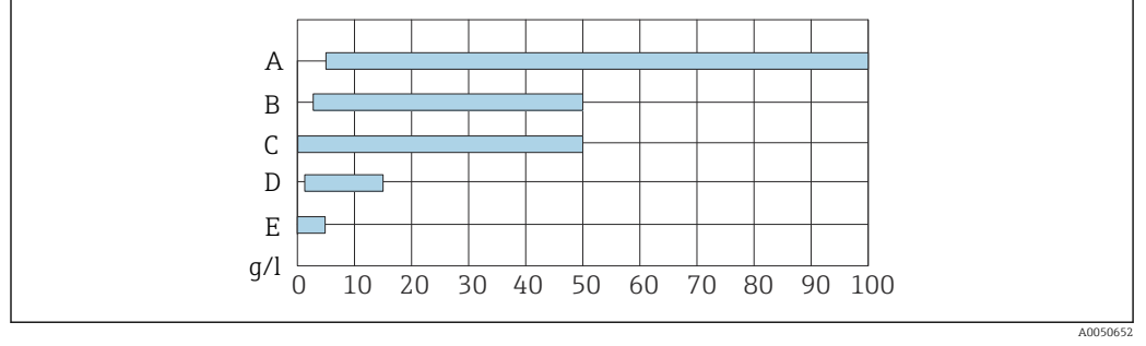
25 Katı uygulama tipi
