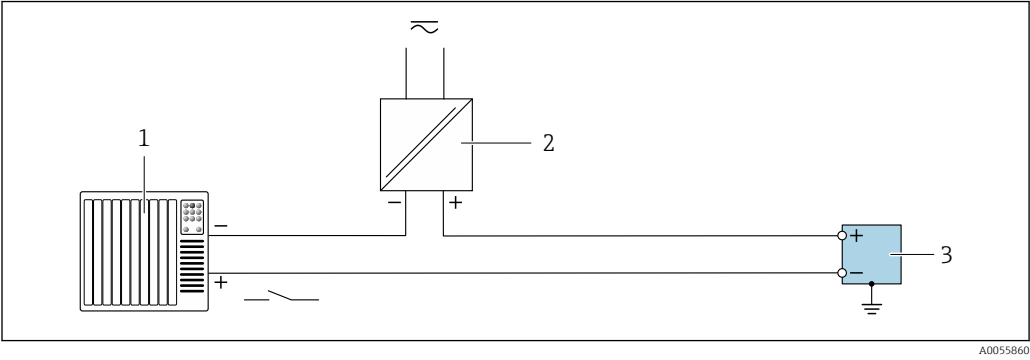
26 Exemple de raccordement pour l'entrée état 1 Système d'automatisation avec sortie tout ou rien passive p. ex. API) 2 Alimentation électrique 3 Transmetteur avec entrée d'état
