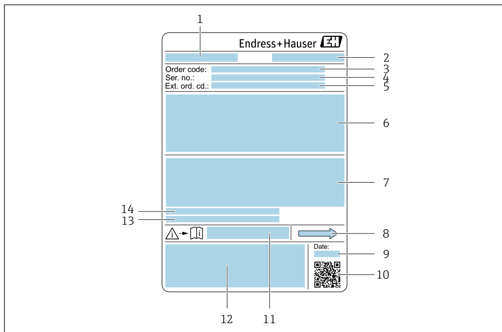
5 センサ銘板の例
