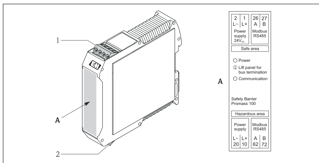
8 Barrière de sécurité Promass 100 avec raccords
