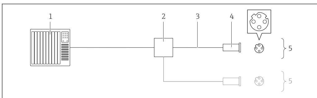
16 Câble de raccordement pour PROFINET
