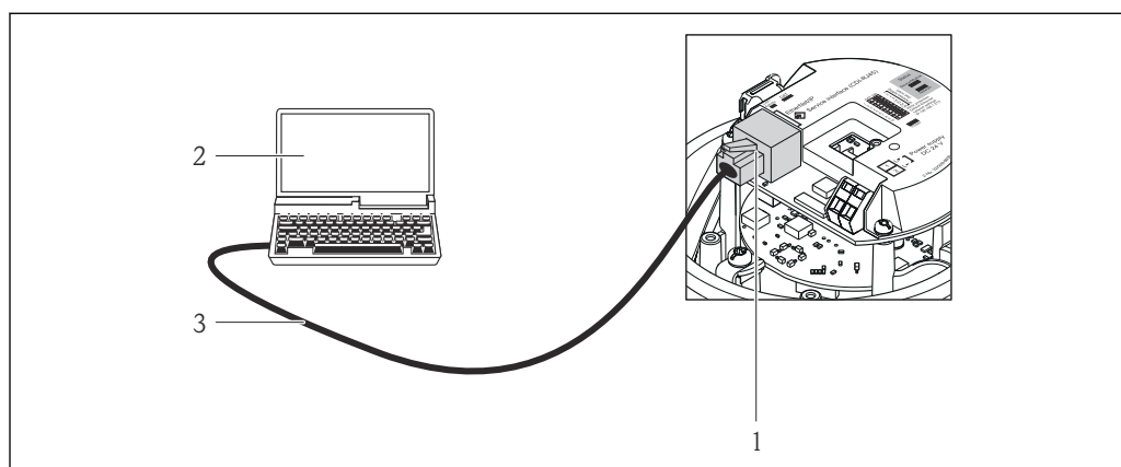
37 Connexion pour la variante de commande "Sortie", option R : PROFINET
