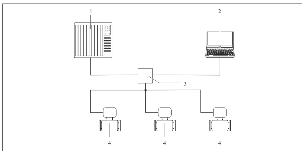
33 Options de configuration à distance via réseau PROFINET
