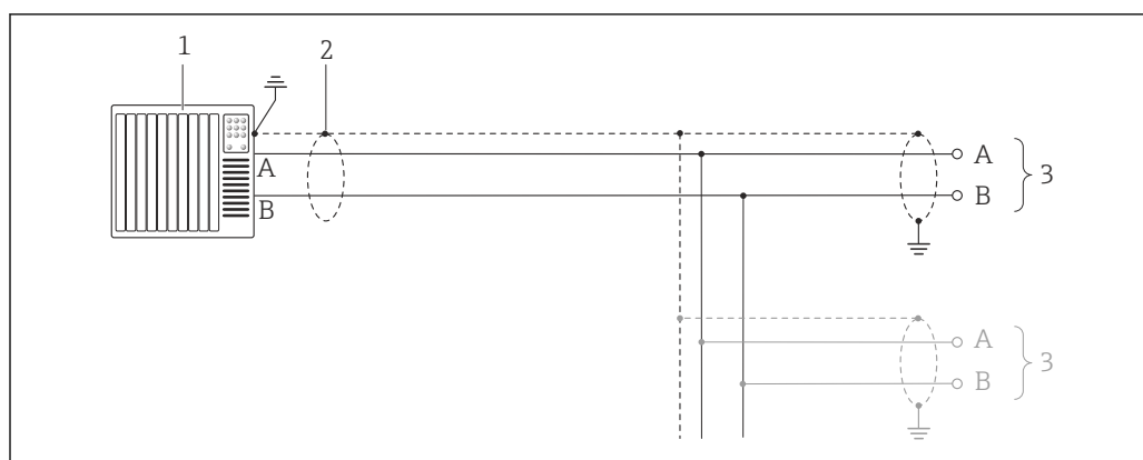
12 Exemple de raccordement pour PROFIBUS DP, zone non explosible et zone 2/Div. 2
