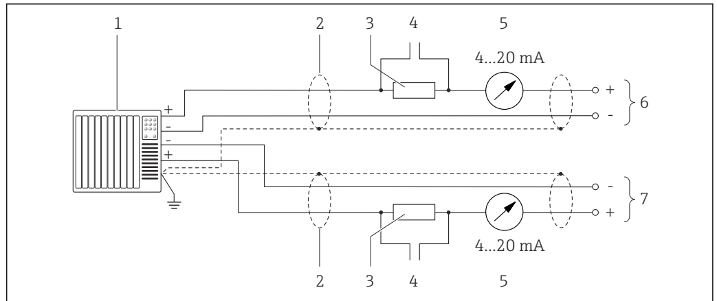
18 Exemple de raccordement pour entrée HART (mode maître) via sortie courant (active)
