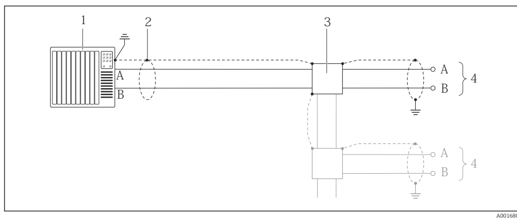
13 Exemple de raccordement pour Modbus RS485, zone non explosible et zone 2/Div. 2
