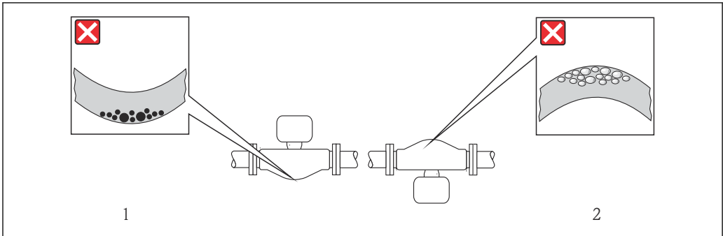
☒ 20 Orientation du capteur avec tube de mesure coudé
