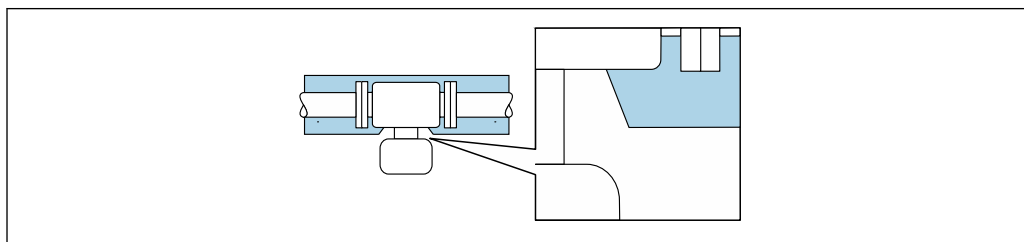
26 Isolation thermique avec tube prolongateur découvert
