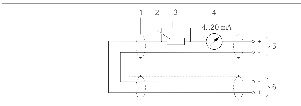
17 Exemple de raccordement pour entrée HART (mode Burst) via sortie courant (active)
