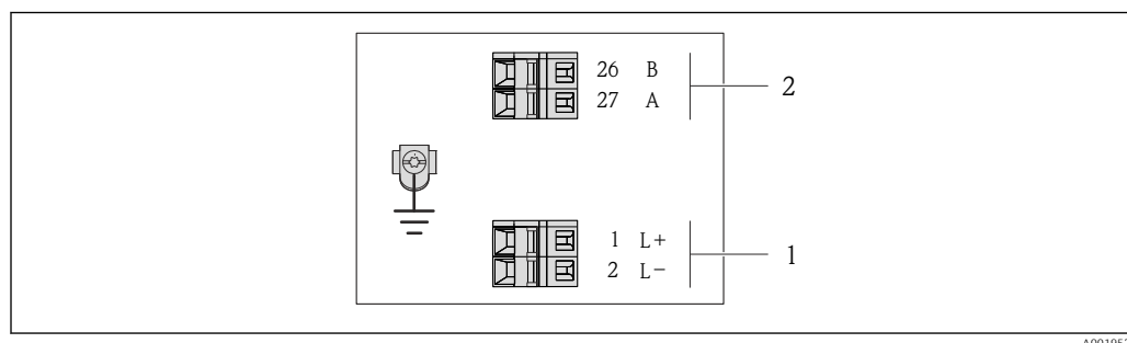
4 Occupation des bornes Modbus RS485, variante de raccordement pour l'utilisation en zone non explosible et en zone 2/Div. 2
