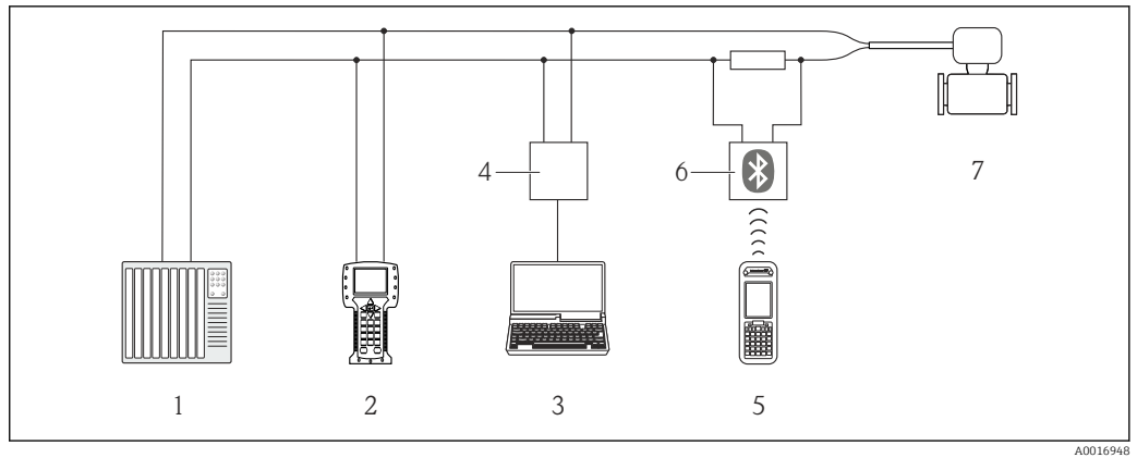
30 Options de configuration à distance via protocole HART
