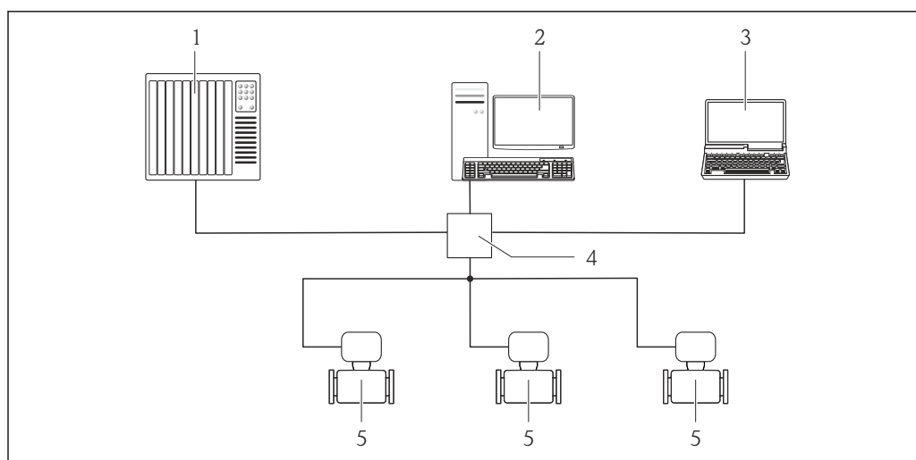
32 Options de configuration à distance via bus de terrain basé sur Ethernet
