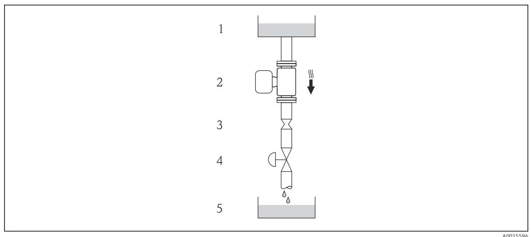
19 Montage dans un écoulement gravitaire (par ex. applications de dosage)
