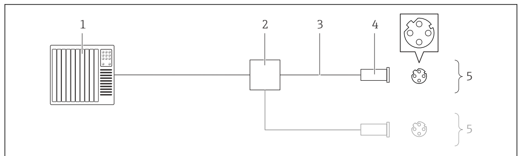
15 Exemple de raccordement pour EtherNet/IP
