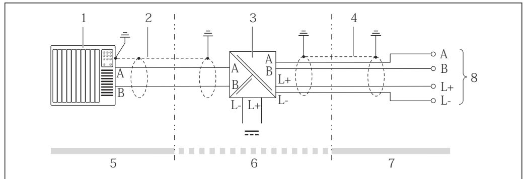
14 Exemple de raccordement pour Modbus RS485 sécurité intrinsèque
