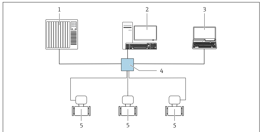
30 Opzioni per il funzionamento a distanza mediante rete EtherNet/IP: topologia a stella
