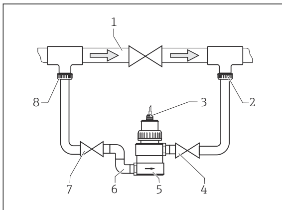
8 Installation en bypass avec des vannes manuelles ou des électrovannes
