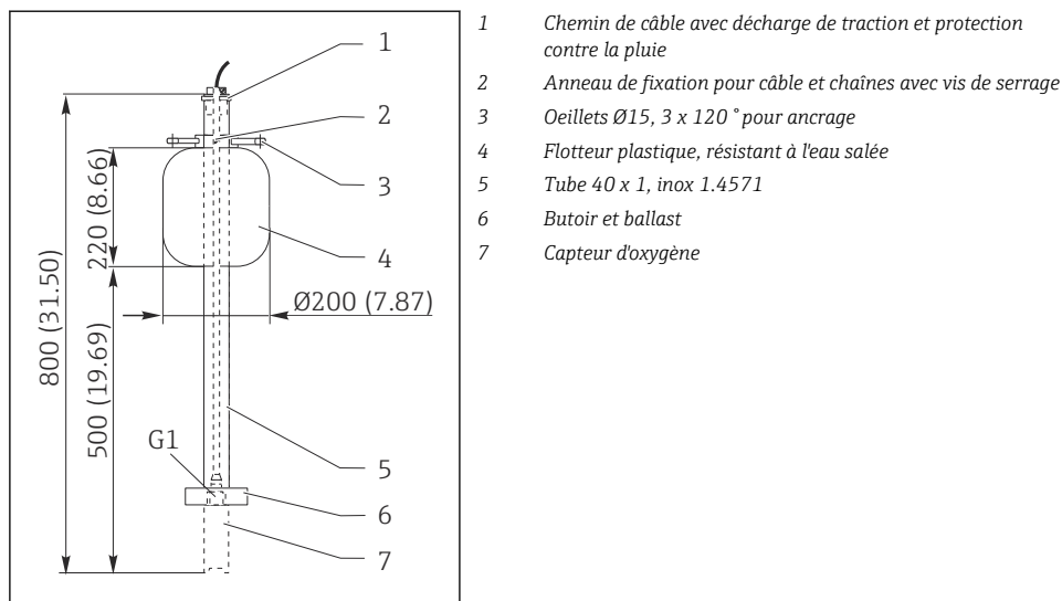
6 Dimensions en mm (inch)
