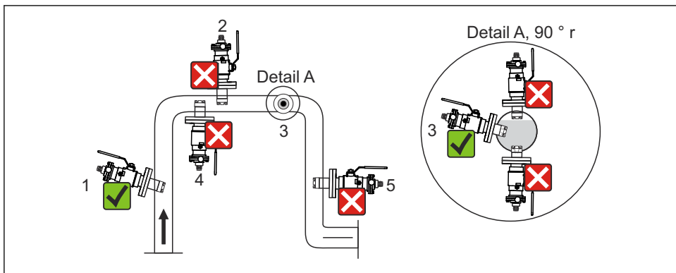
9 Positions de montage adaptées et inadaptées avec la sonde rétractable COA451
