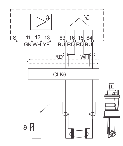
7 Anslutning av induktiva sensorer
