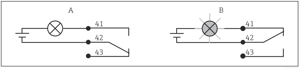
9 Commutation de sécurité recommandée pour le contact d'alarme
