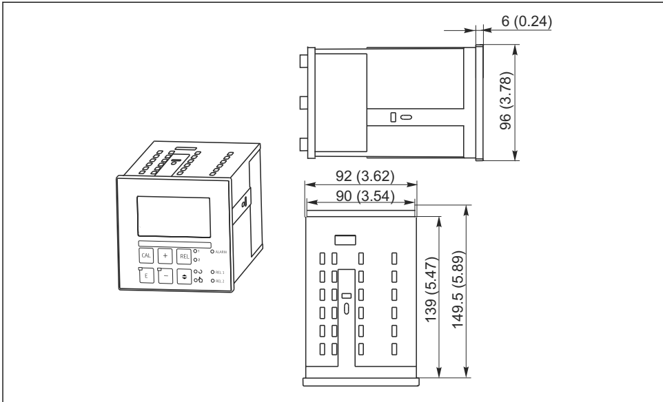
1 Appareil encastrable, dimensions en mm (in)
