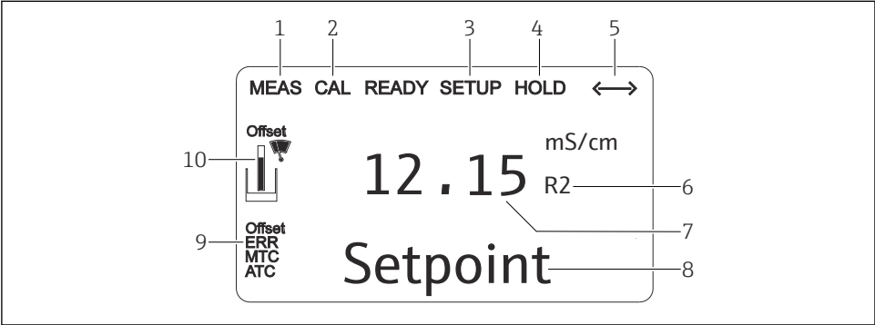
10 Afficheur LCD du transmetteur
