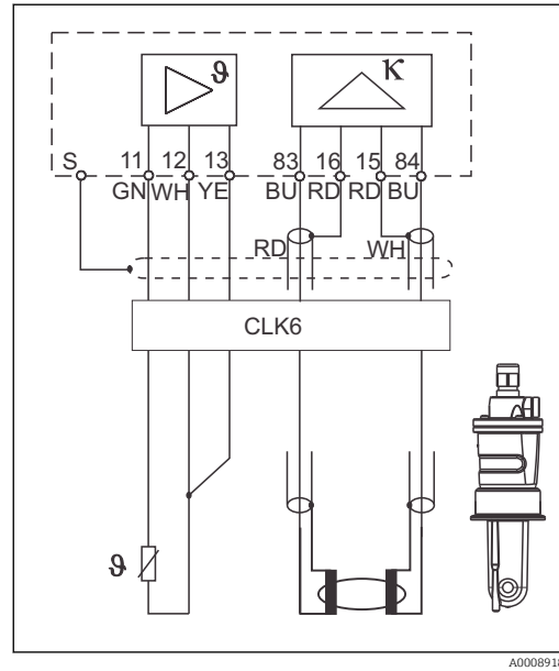
8 Raccordement de capteurs inductifs
