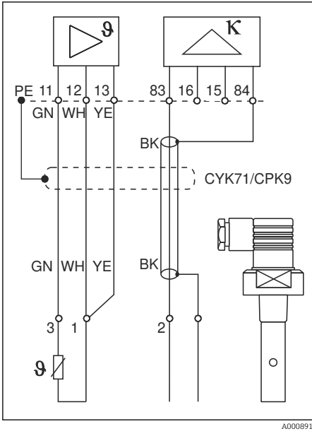
7 Raccordement de capteurs conductifs
