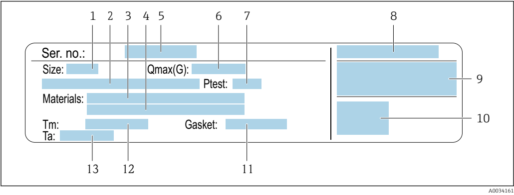
4 Esempio di targhetta del sensore
