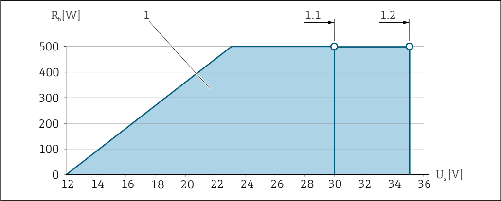
14 Carico per versione compatta senza display locale
