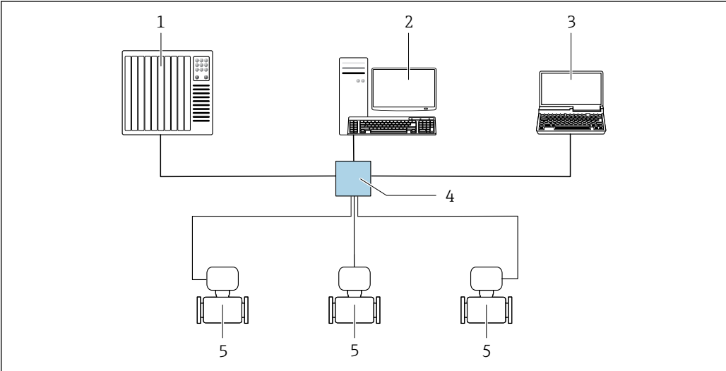
图 23 通过 Modbus TCP + Ethernet 进行远程操作 - 100 Mbit/s: 星形拓扑结构
