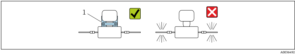
1 传感器安装架（订购选项“安装附件”，选型代号 PR）
