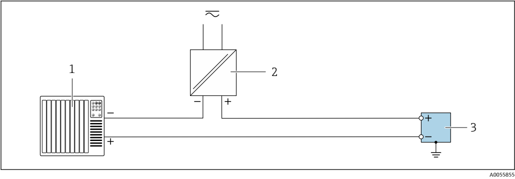
14 接线实例：脉冲输出/频率输出/开关量输出（无源）
