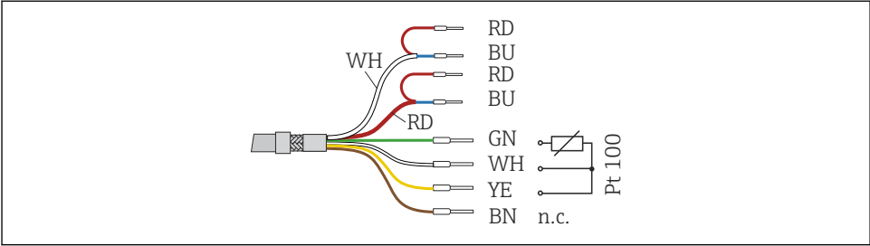
8 整体电缆或 CLK6 测量电缆
