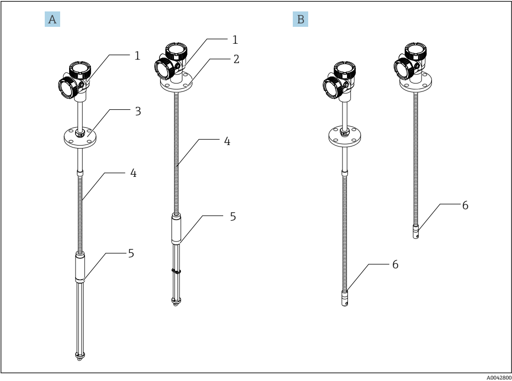
1 Prothermo NMT81 的结构设计 A NMT81，带油水界面测量探头（WB） B NMT81，不带油水界面测量探头（WB） 1 转换器 2 焊接法兰 3 活动法兰 4 柔性温度探头 5 油水界面测量探头（WB） 6 柔性温度探头，不带油水界面测量探头（WB）
