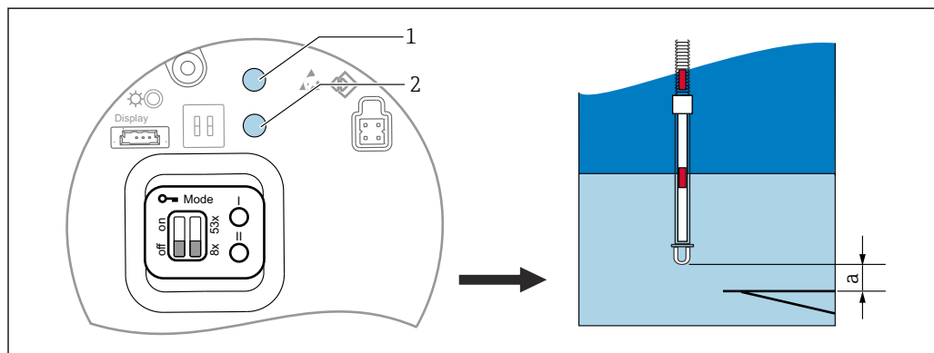
图 50 液位设置
