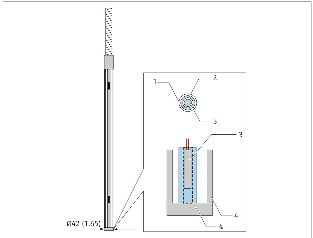
图 12 油水界面测量探头结构。测量单位 mm (in)
