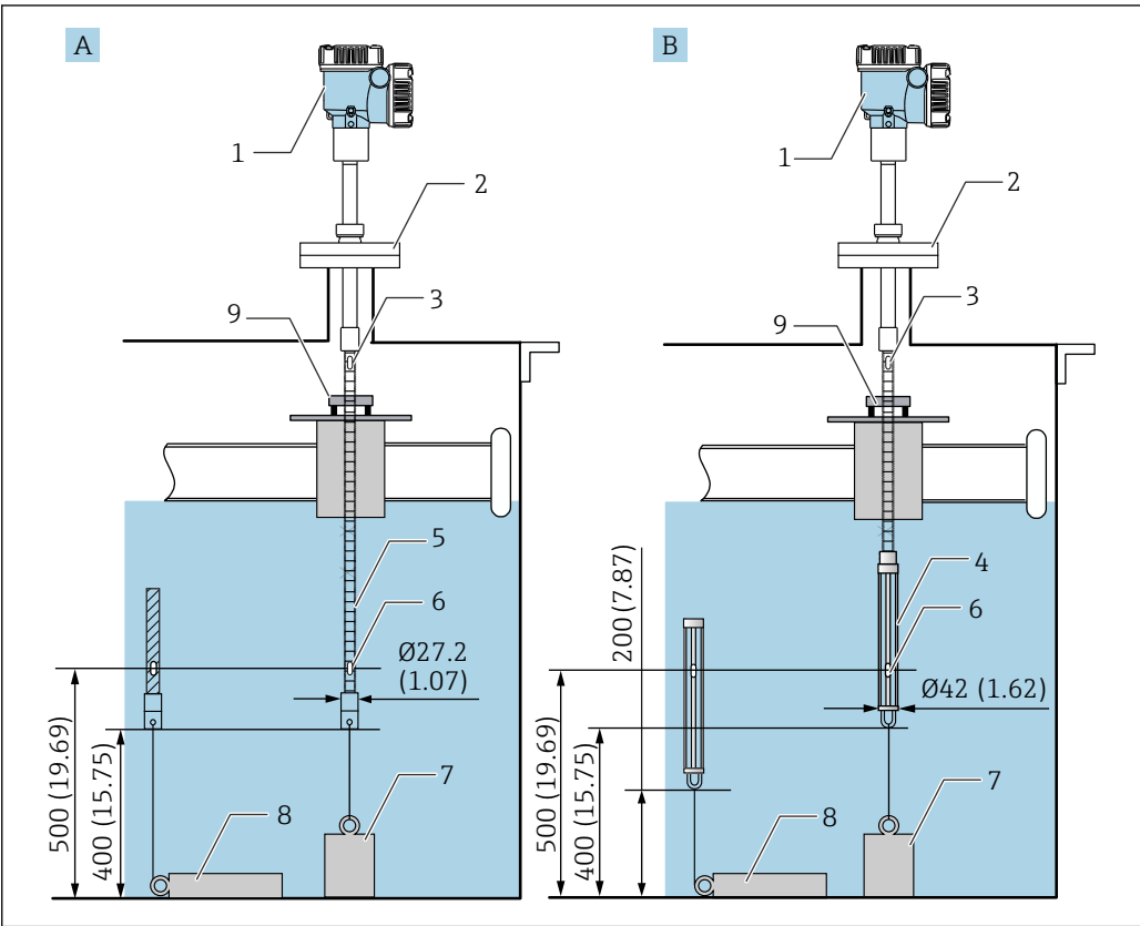
图 32 使用导向环和锚固配重。测量单位 mm (in)
