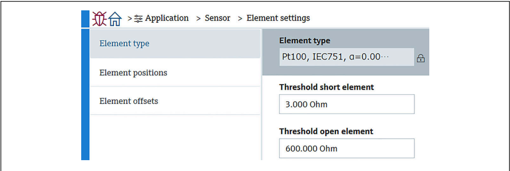
87 测温元件设置子菜单界面
