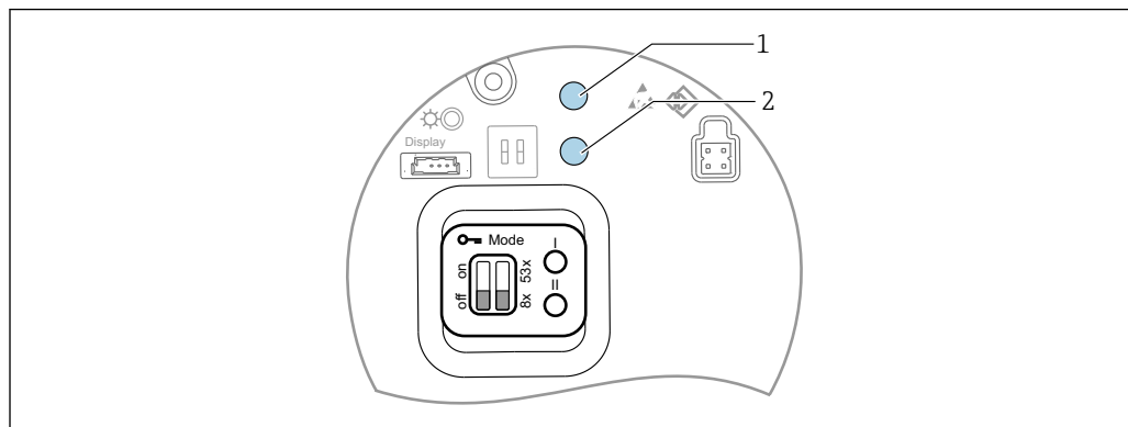
图 49 恢复出厂设置
