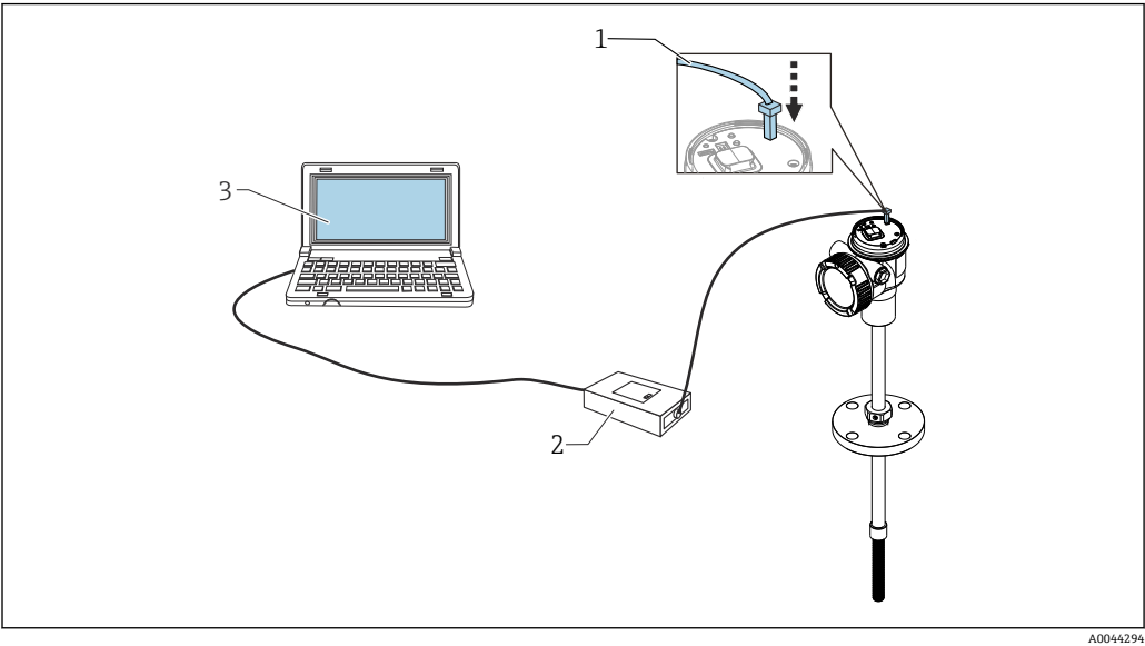
图 53 通过服务接口操作
