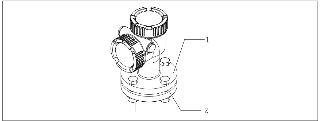
图 20 无高度调整装置的仪表
