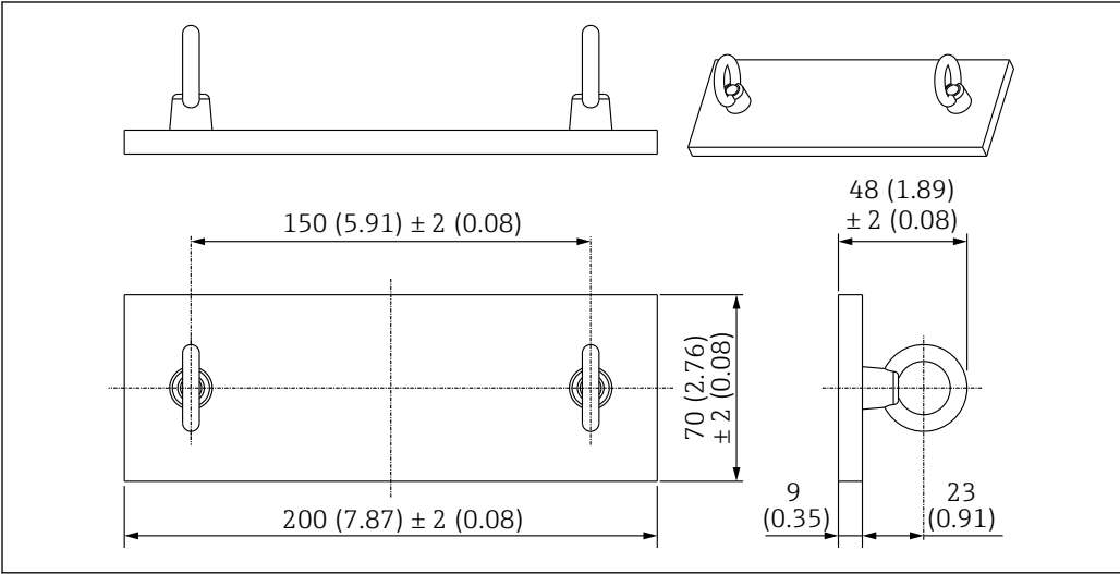
图 118 绞线连接孔。测量单位 mm (in)
