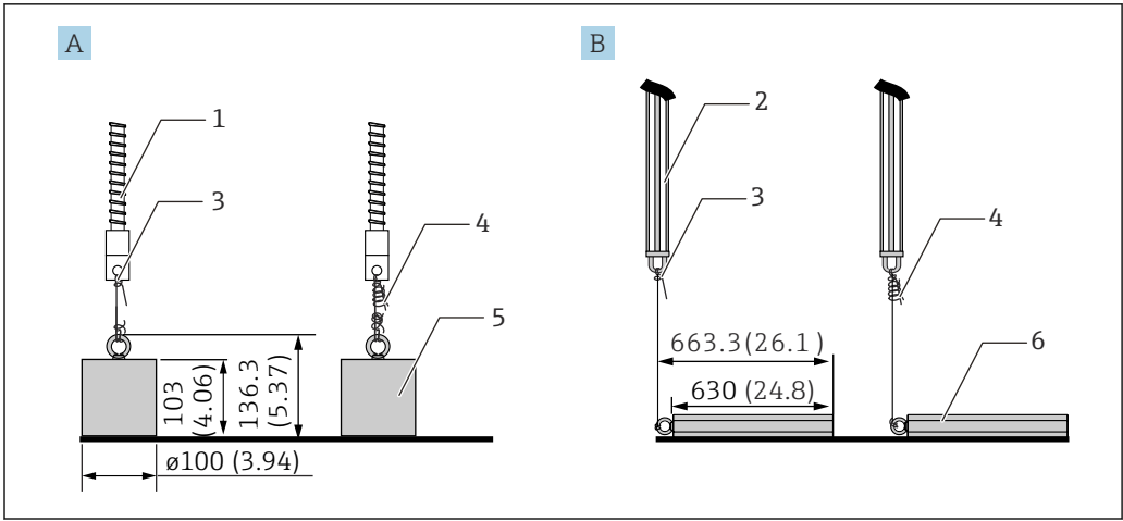
29 安装锚固配重
