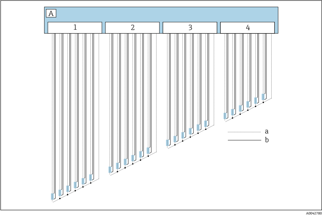
36 四线制接线图
