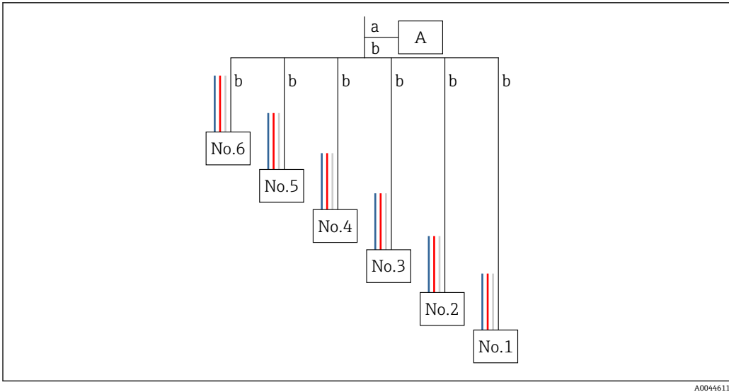
43 四线制结构
