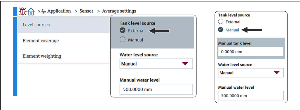
81 储罐液位源/水位源子菜单界面
