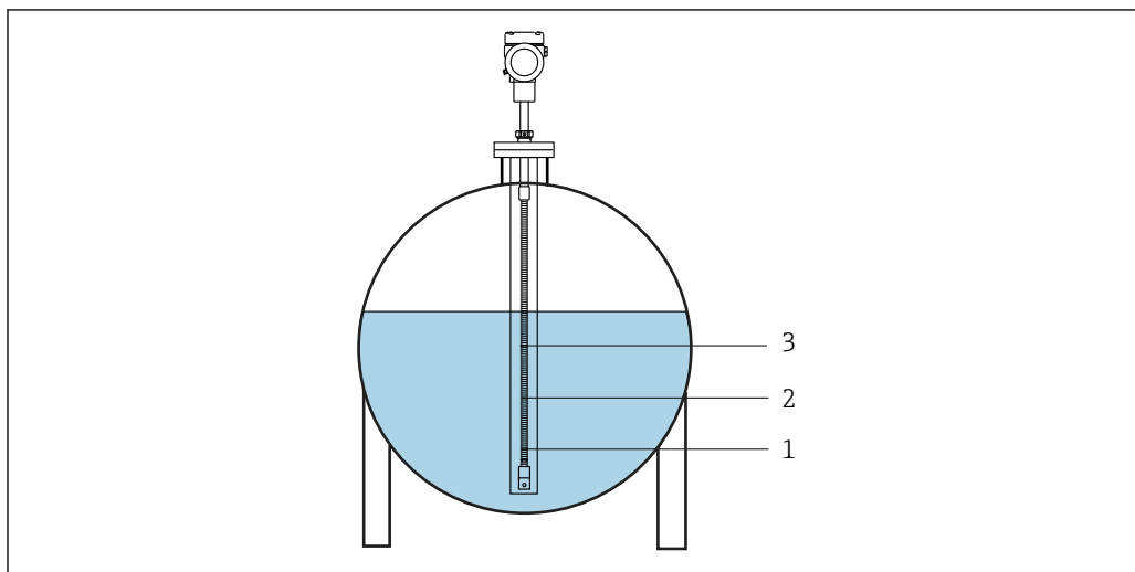
图 85 液体温度的标准计算法
