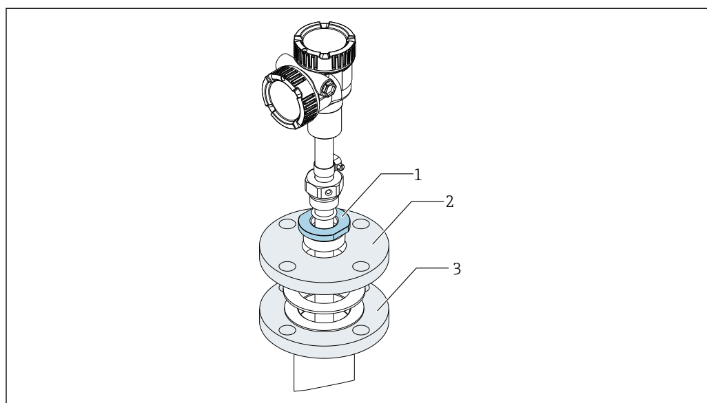
图 22 螺纹调整
