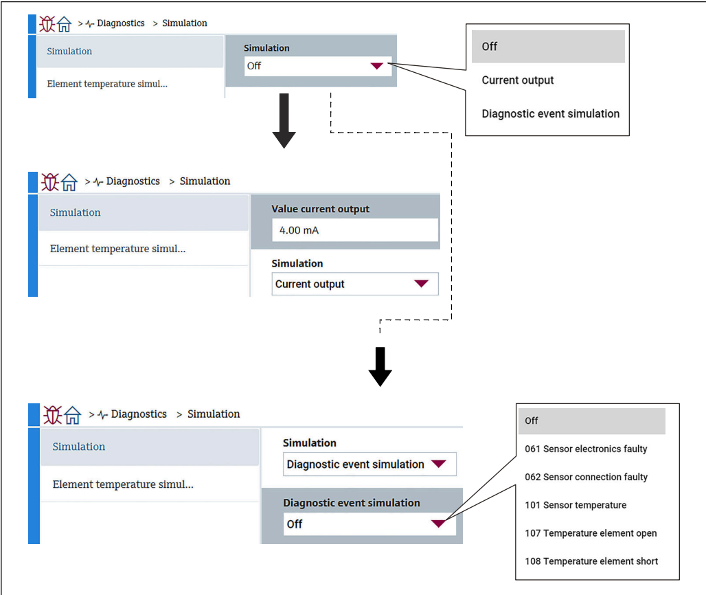
108 仿真子菜单界面
