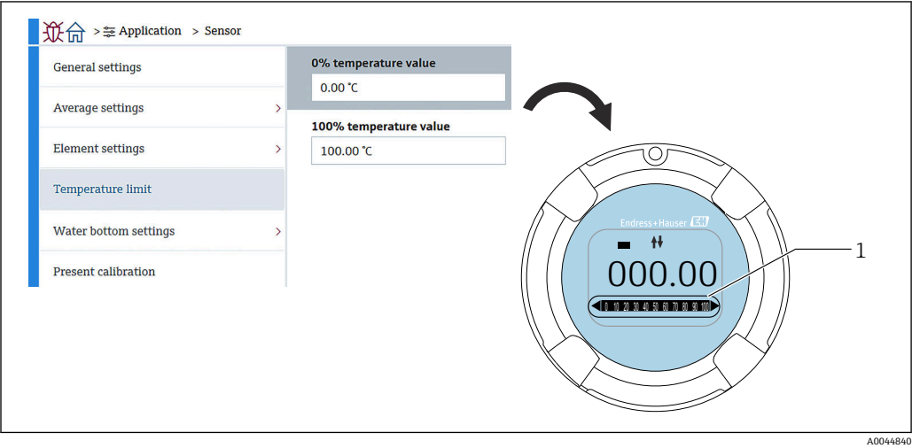
91 温度限值
