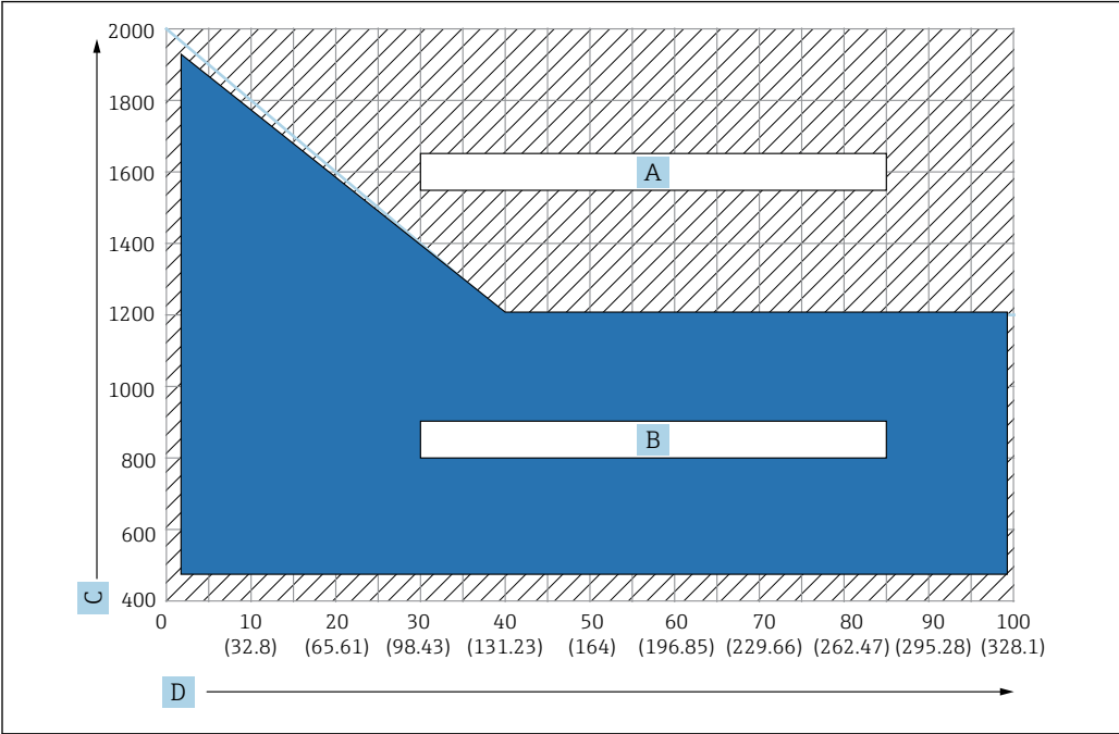
图 117 锚固配重选型图 C: 密度单位[kg/m3], D: 长度单位 m/(ft)
