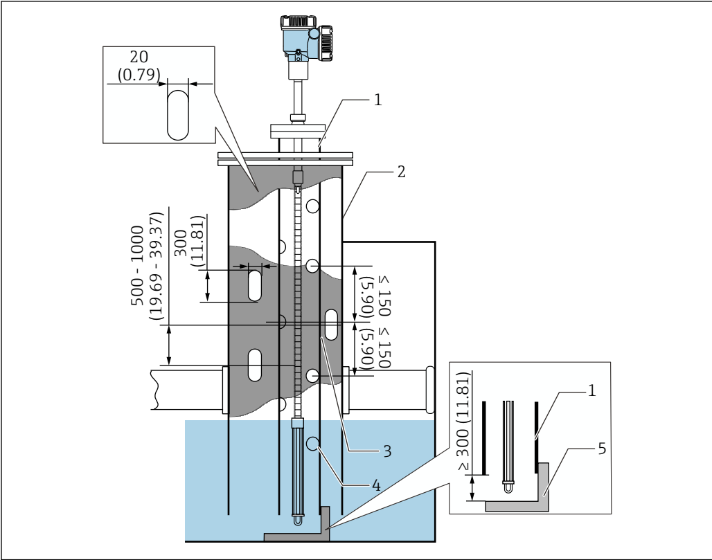
图 31 安装在导波管中。测量单位 mm (in)
