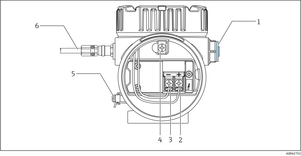
图 35 NMT81 的接线端子 (ATEX 本安防爆)
