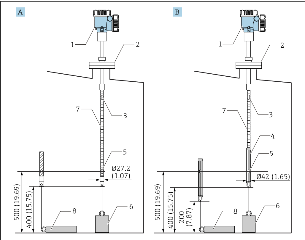
图 28 使用锚固配重。测量单位 mm (in)
