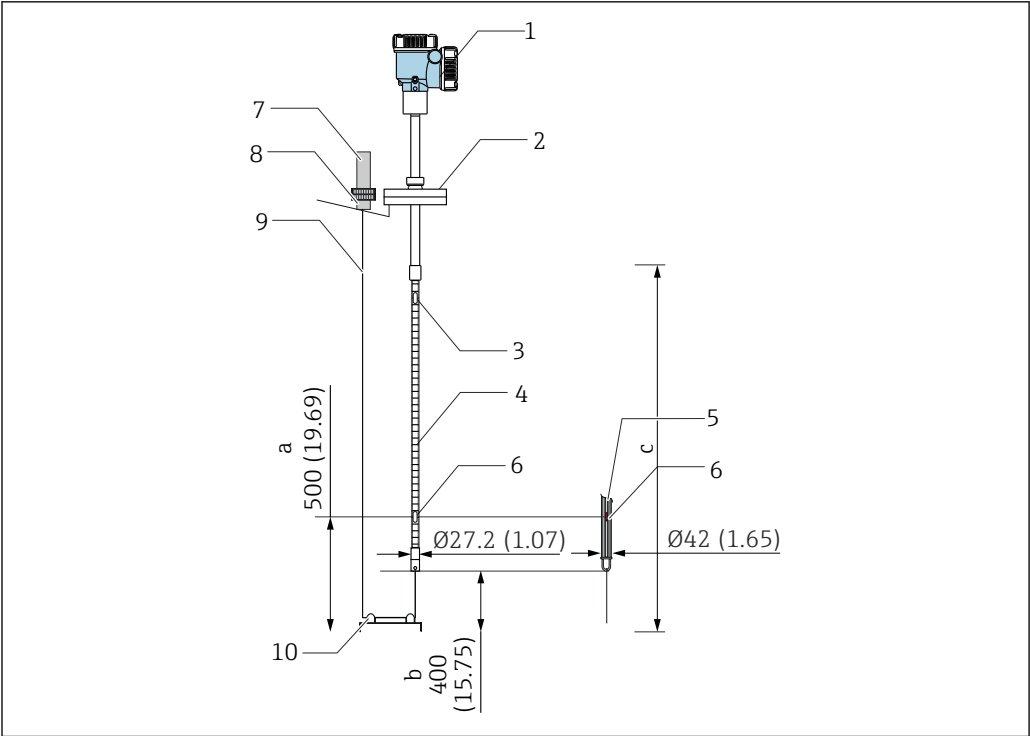
图 24 使用顶部锚固装置。测量单位 mm (in)
