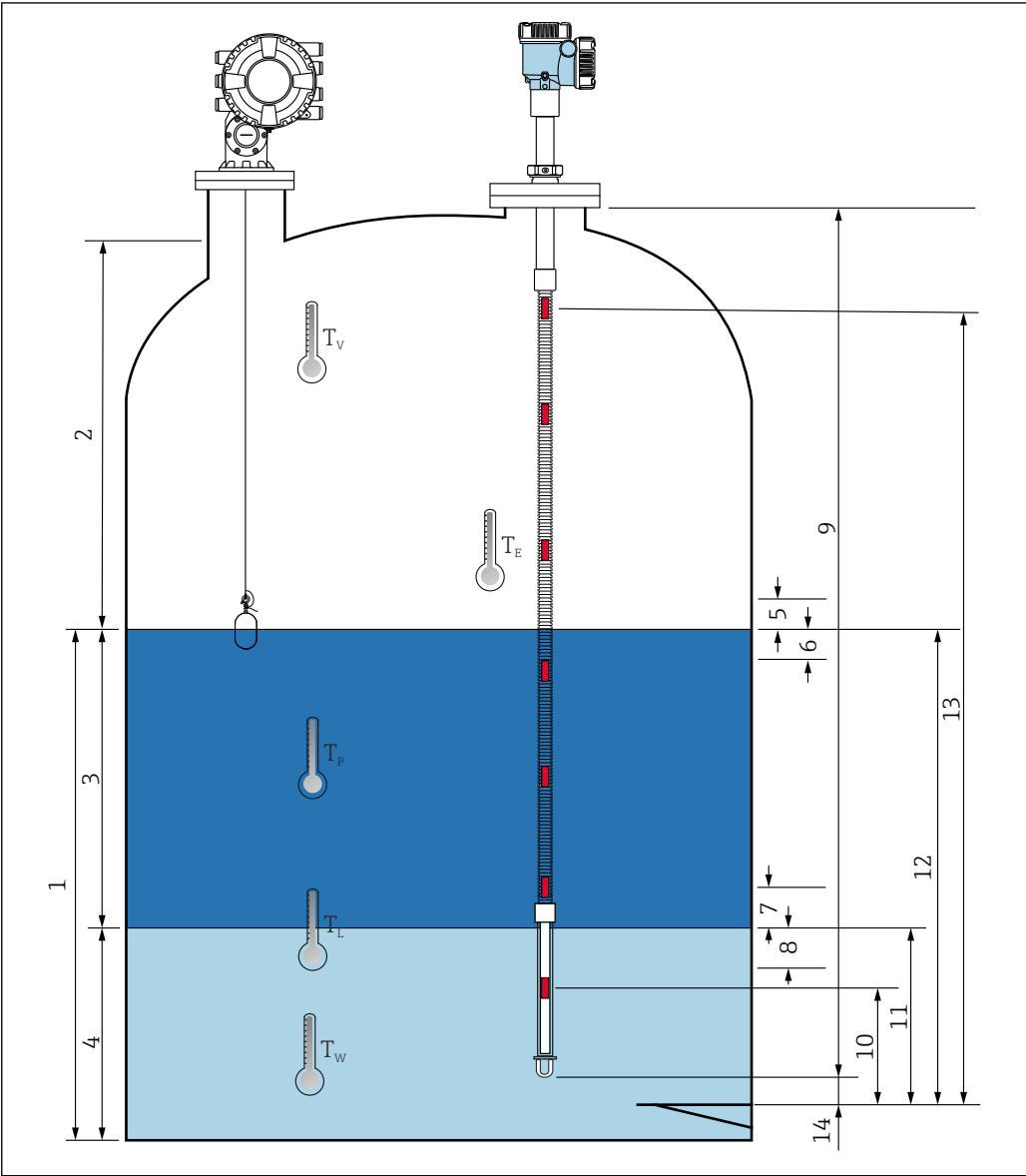
55 与 NMT81 安装相关的术语
