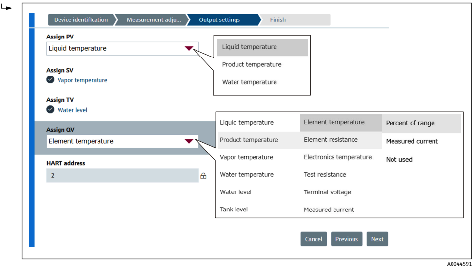
63 输出设置界面
