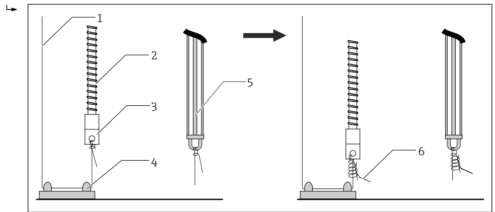
25 安装顶部锚固装置 (第 1 部分)
