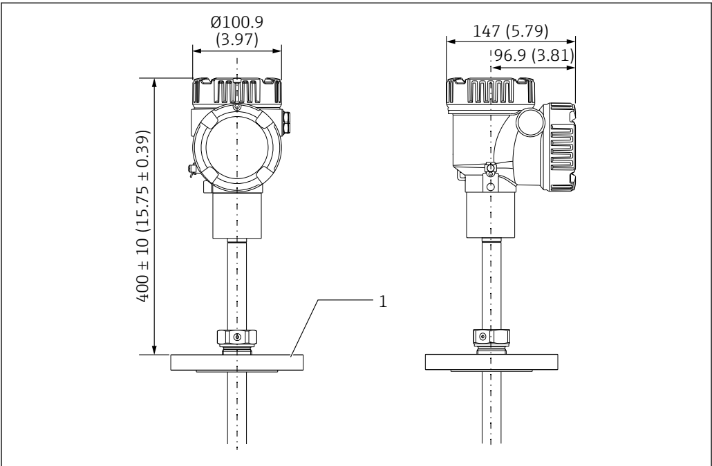
9 活动法兰。测量单位 mm (in)
