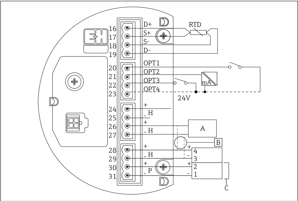
39 NRF590 的本安接线端子
