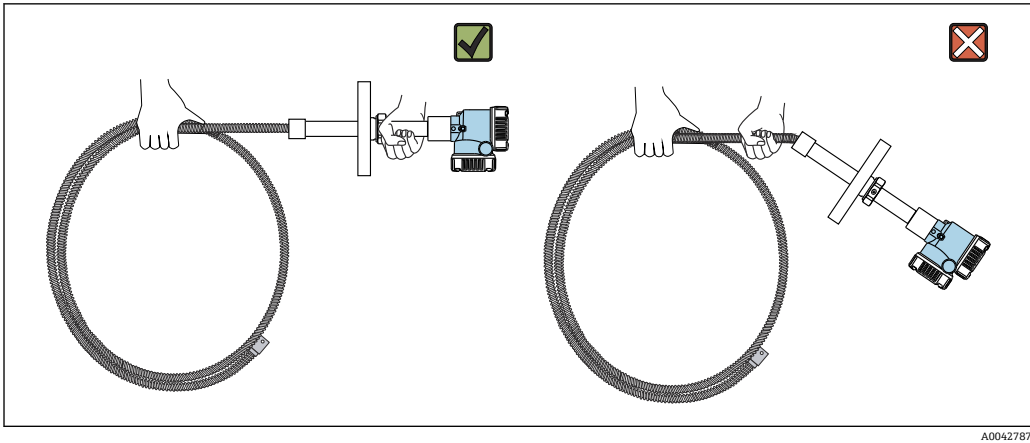
图 15 拆除 NMT81 包装
