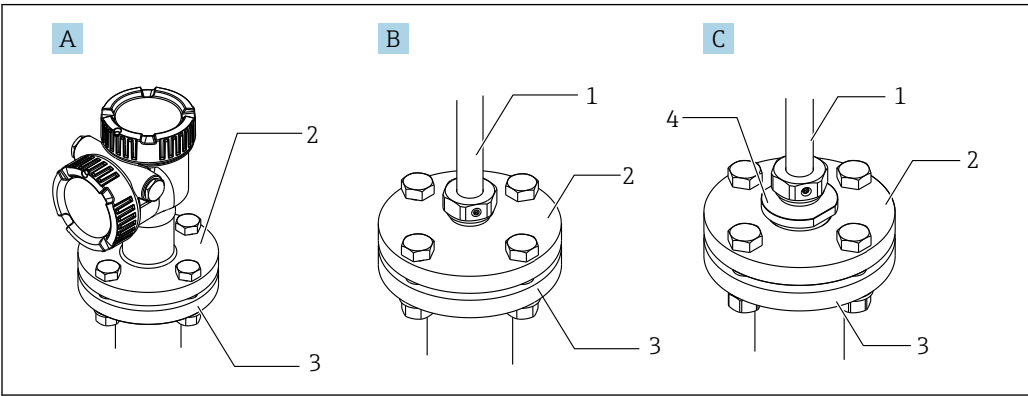
图 19 法兰
