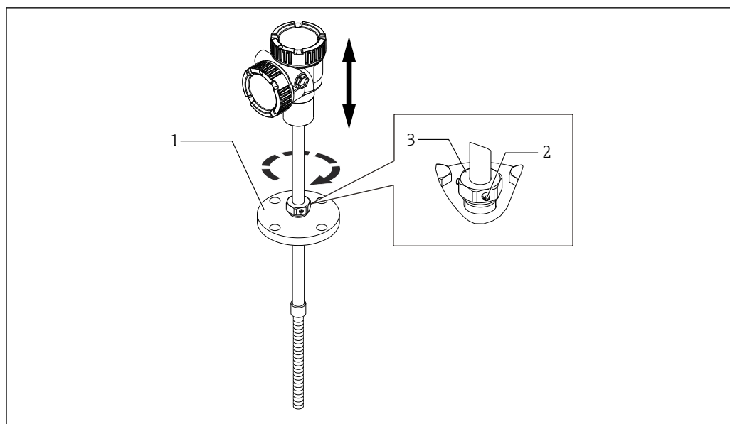
图 21 带高度调整装置的 NMT81 示意图
