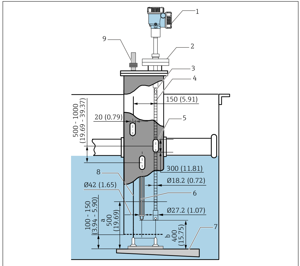
图 30 使用顶部锚固装置。测量单位 mm (in)
