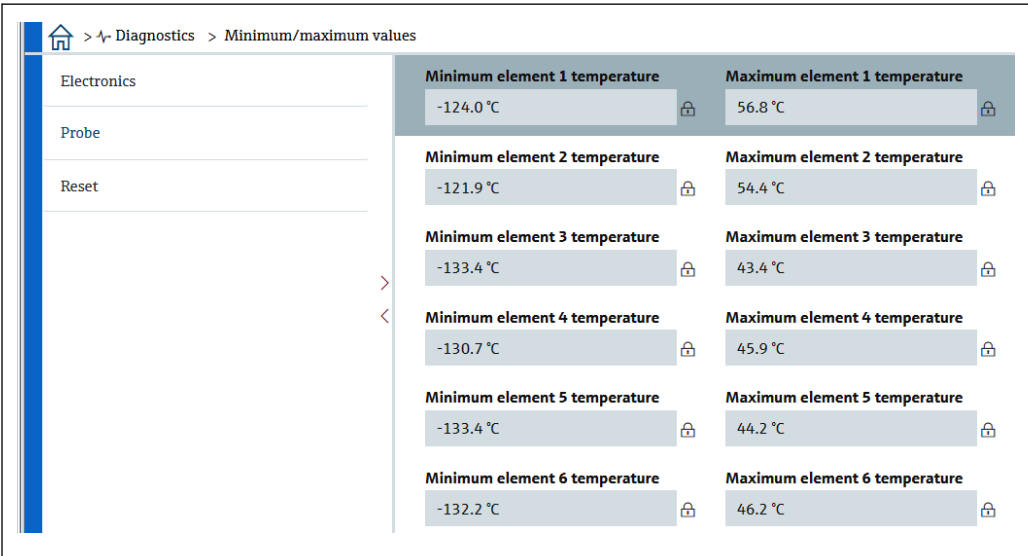
107 Probe 界面
