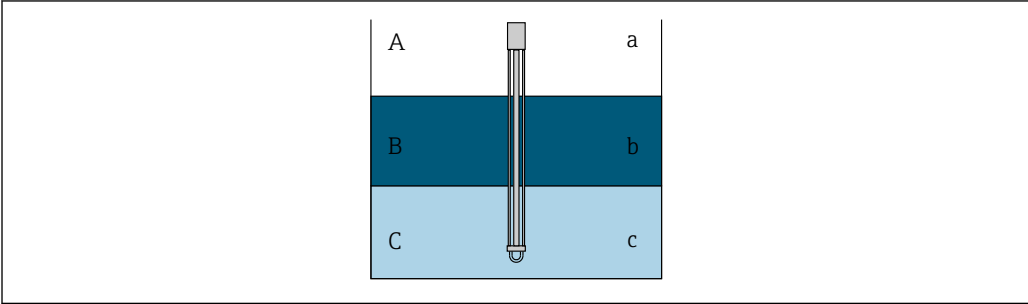
图 13 三层介质工况中的水层厚度测量
