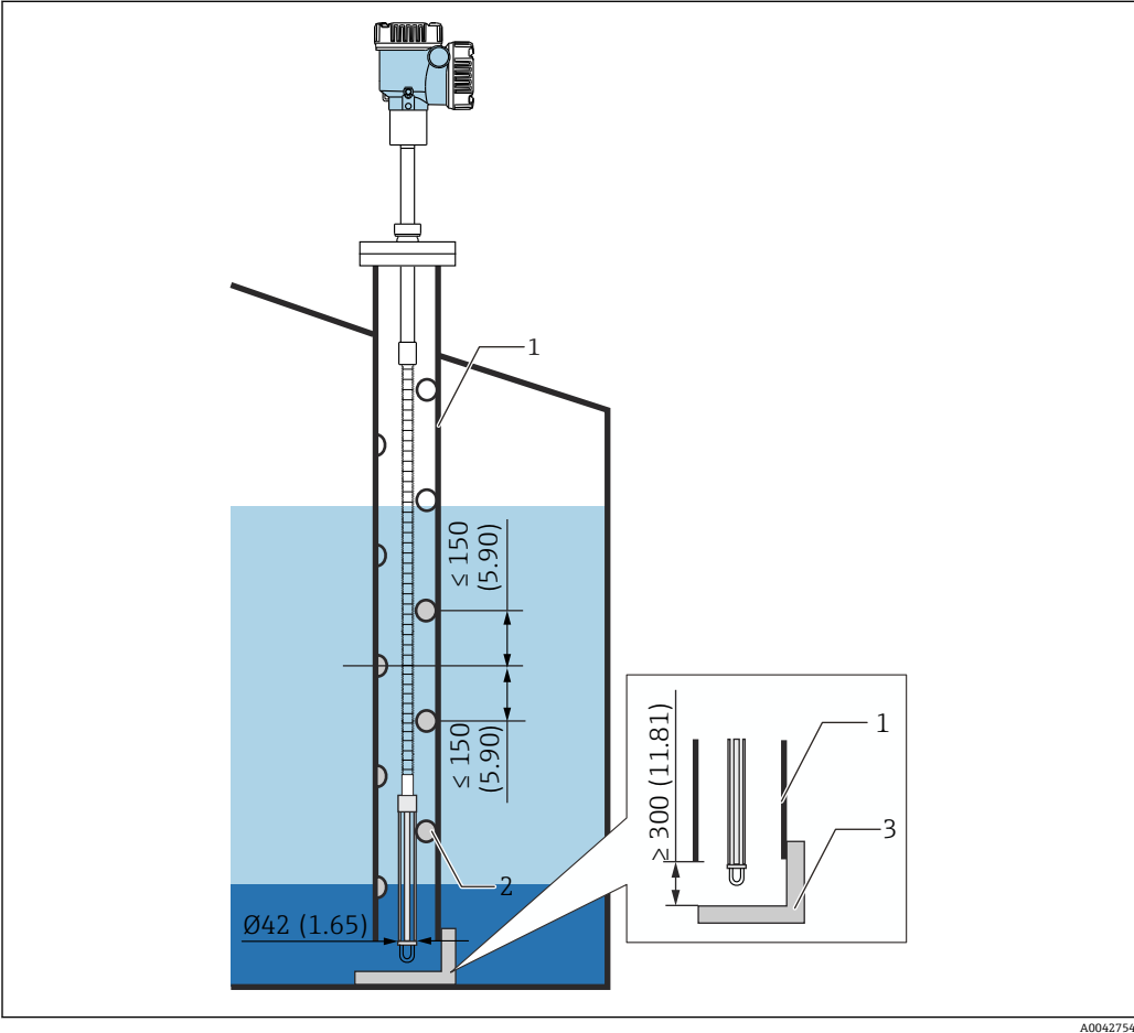
图 27 导波管。测量单位 mm (in)
