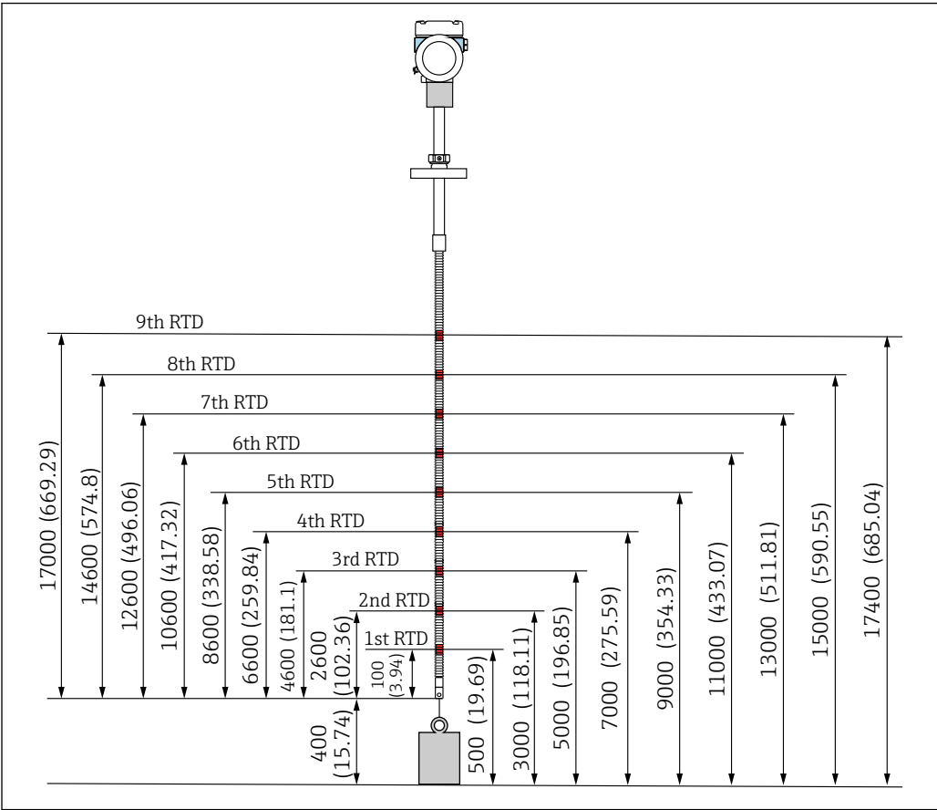
11 元件位置。测量单位 mm (in)
