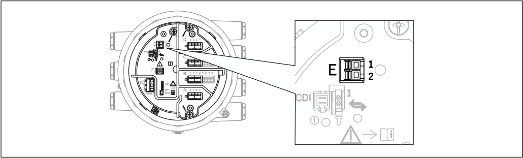
37 NMS8x 的接线端子，用于连接 NMT81
