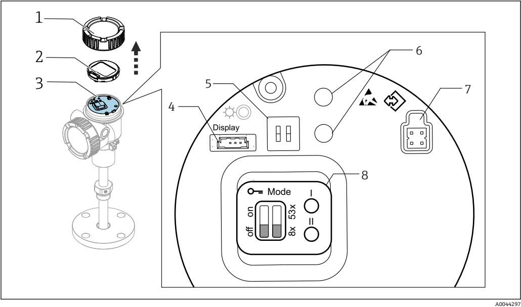
图 47 电子模块 1 外壳盖 2 显示单元（可选） 3 主仪表 4 显示单元接口 5 DIP 开关 6 操作按键 7 FieldCare 接口 8 接口和开关信息标签
