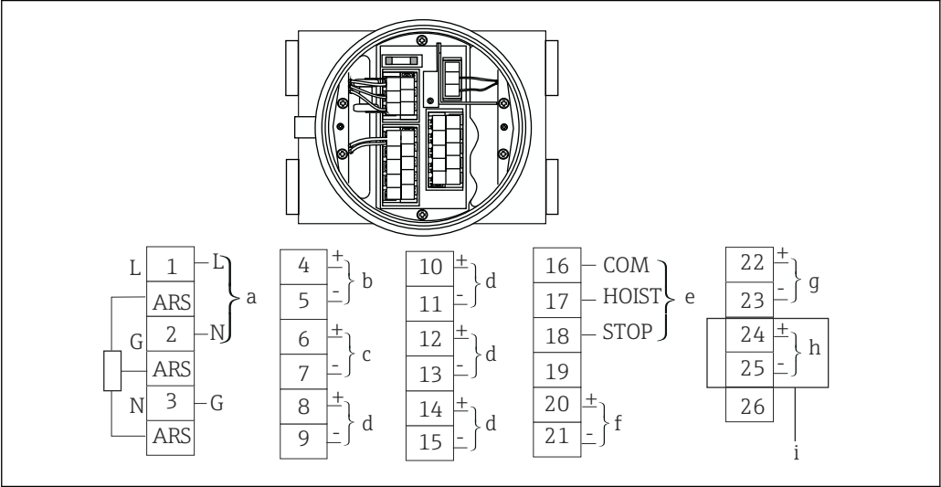
图 38 NMS5 的接线端子
