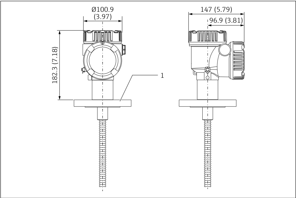
8 焊接法兰。测量单位 mm (in)
