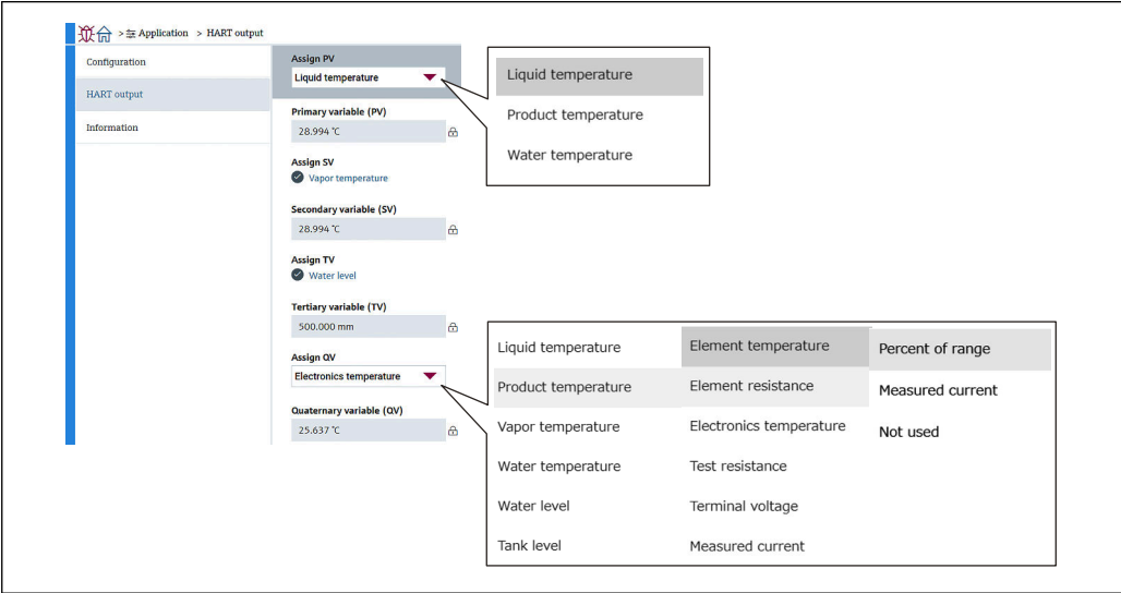
95 HART 输出子菜单界面
