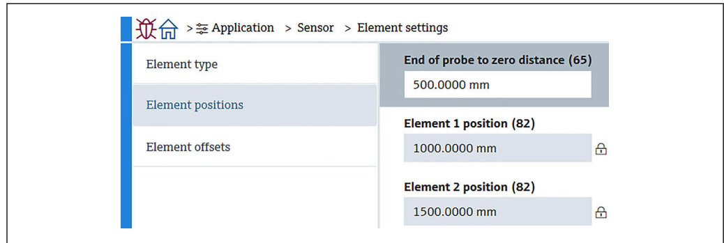
88 Element positions 子菜单界面
