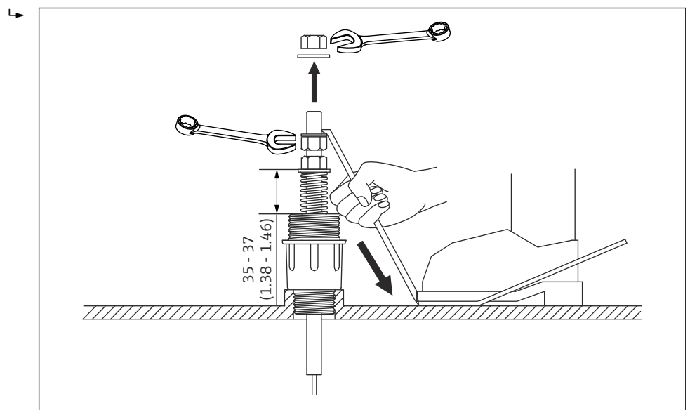
26 安装顶部锚固装置 (第 2 部分)。测量单位 mm (in)
