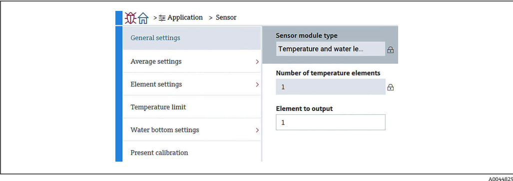
79 常规设置子菜单界面
