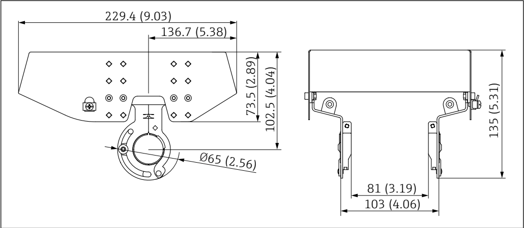
114 防护罩。测量单位 mm (in)
