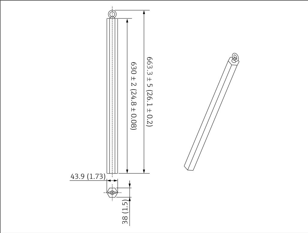
116 安装附件。测量单位 mm (in)
