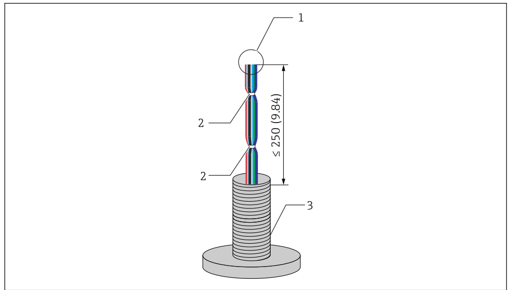
图 40 电缆处理
