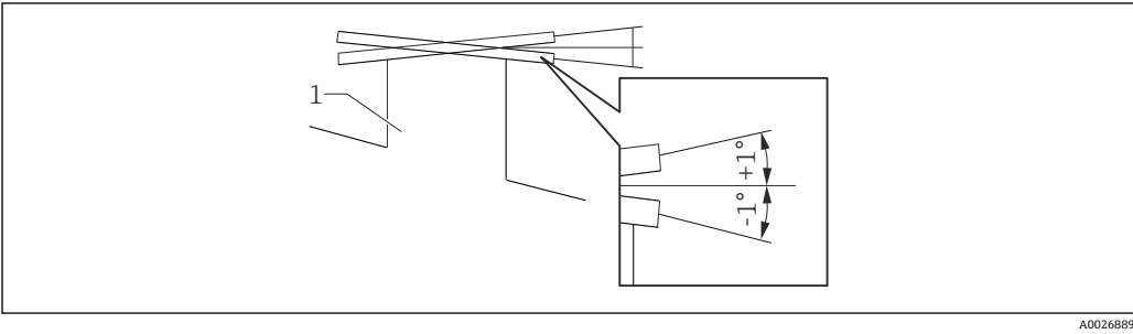
图 18 安装法兰的允许偏差角度范围
