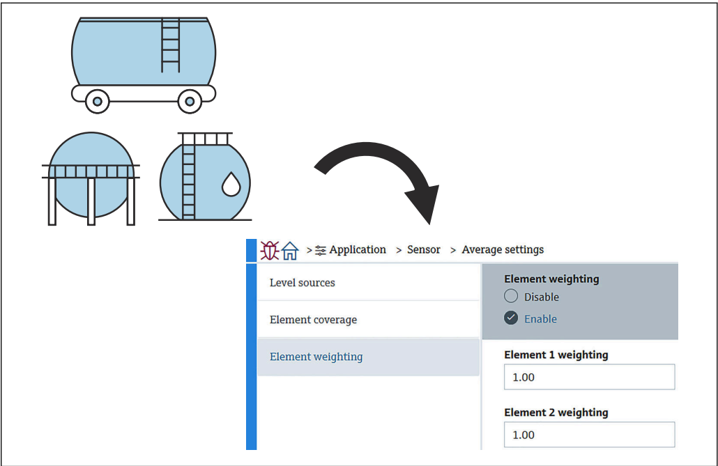
图 84 测温元件权重子菜单界面
