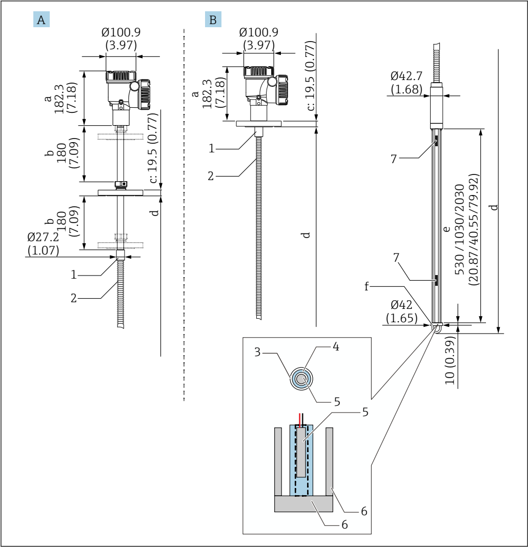
图 7 “转换器+平均温度探头+油水界面测量探头”型仪表。测量单位 mm (in)
