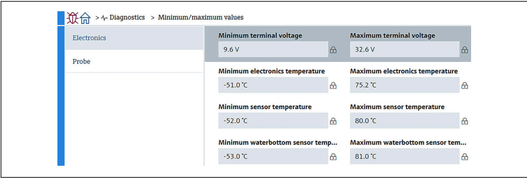
106 Electronics 界面
