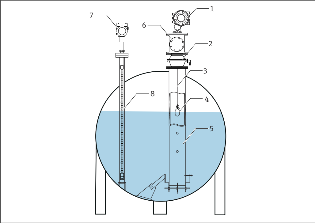
33 在高压罐中安装保护套管
