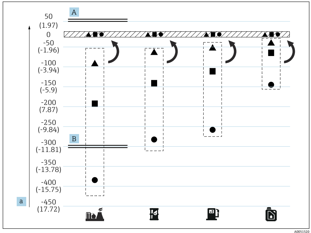
14 针对三层介质工况的补偿功能
