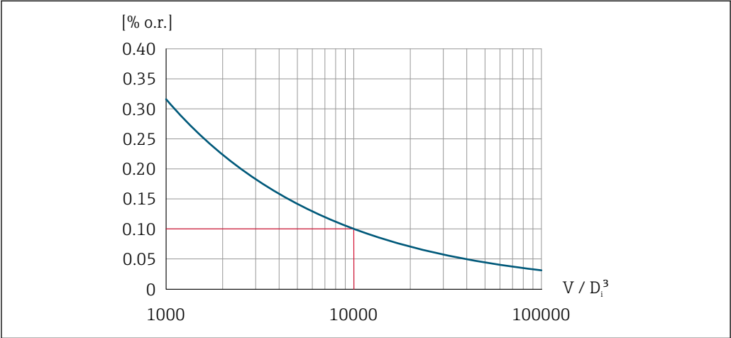
22 Repetibilidade = 0,1 % o.r. com um volume medido [m³] de V = 10\,000 \cdot D_i^3
