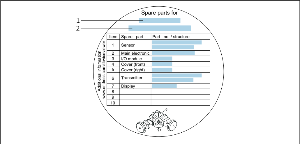
21 Exemplo para "Etiqueta de descrição da peça de reposição" na tampa do compartimento de conexão
