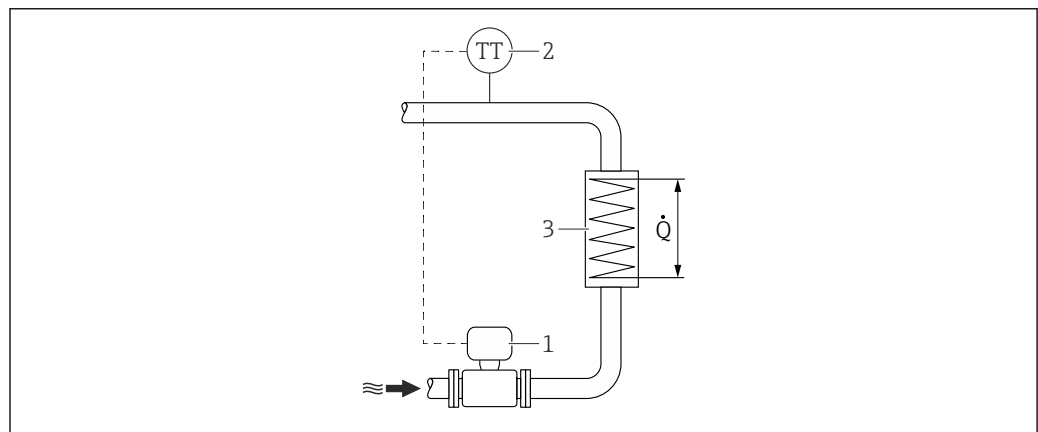
5 Layout para a medição de delta de calor de água e vapor saturado
