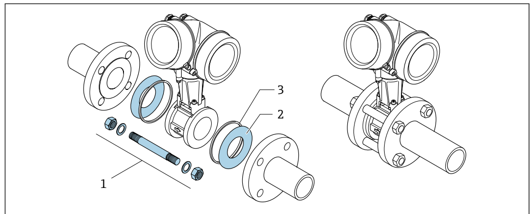
6 Conjunto de montagem para versão wafer
