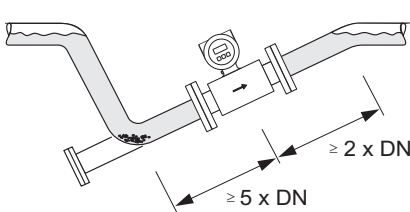
Instalación en una tubería parcialmente llena
