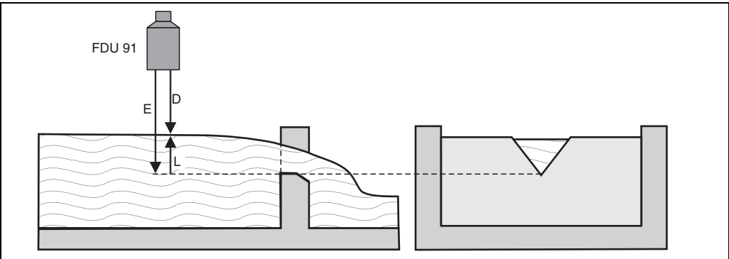
Beispiel: Dreieckswehr E: Leerabgleich; D: gemessene Distanz; L: Füllstand (Pegel)
