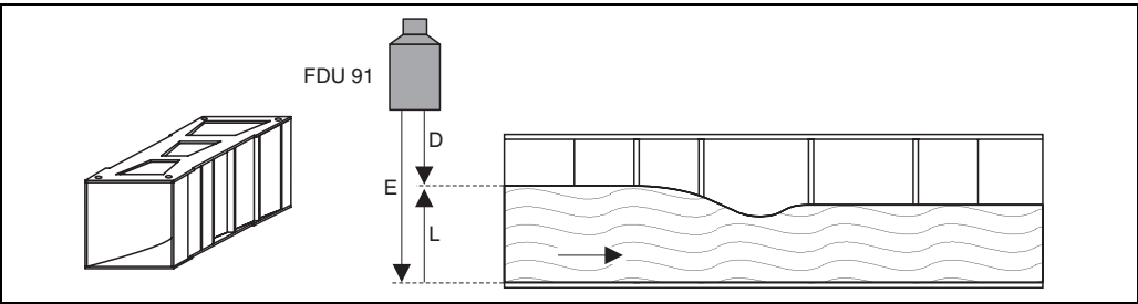
Beispiel: Khafagi-Venturi-Rinne E: Leerabgleich; D: gemessene Distanz; L: Füllstand (Pegel)
