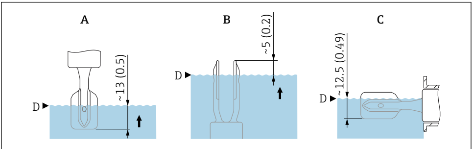
☐ 4 일반적인 스위치 포인트. 측정 단위 mm (in)
