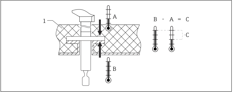
☐ 3 플랜지의 바깥쪽과 안쪽의 온도 차이
