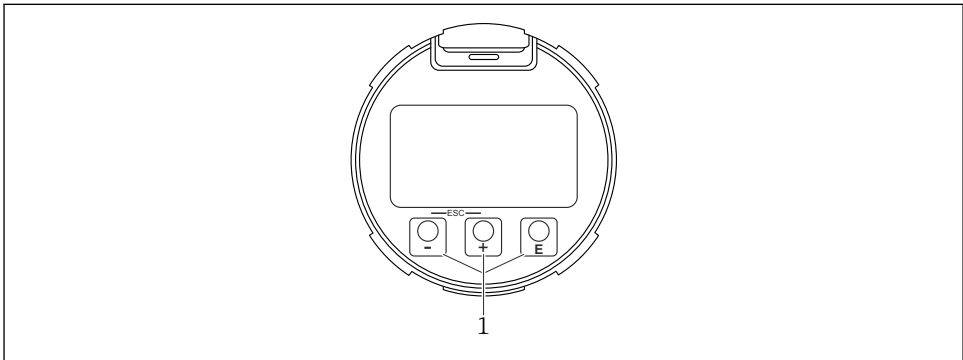
☒ 22 광학 작동 키(1)가 있는 그래픽 디스플레이
