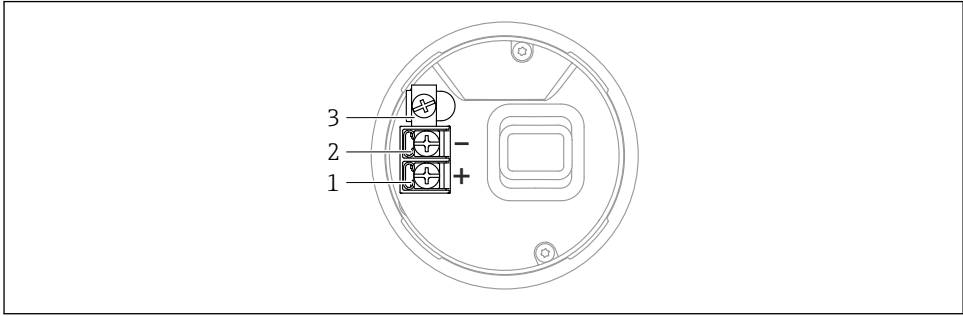
☐ 17 연결부의 연결 단자 및 접지 단자, 단일 격벽 하우징
