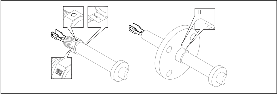
☞ 10 마킹을 사용하여 용기에 수직으로 설치할 때 진동 포크의 위치
