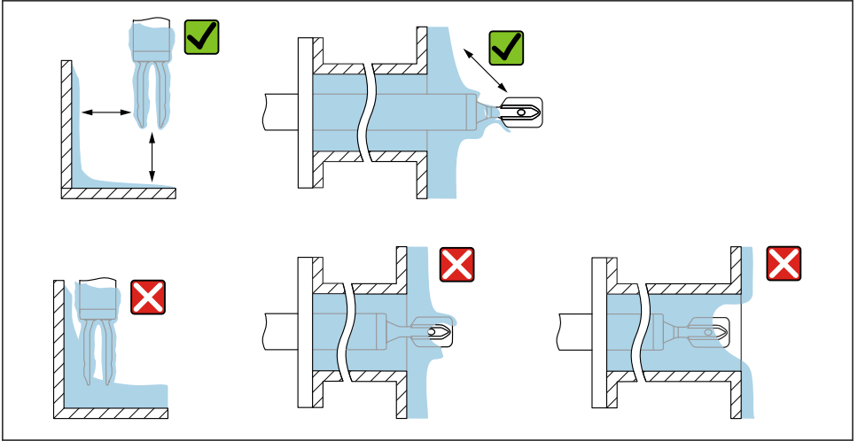
☞ 7 고점성 프로세스 유체용 설치 예
