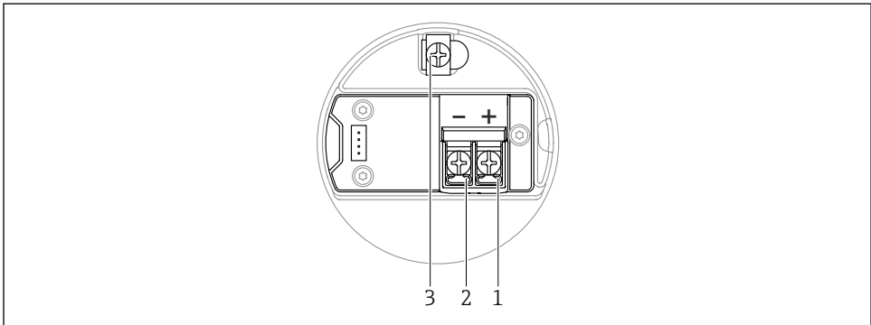
☐ 18 연결부의 연결 단자 및 접지 단자, 이중 격벽 하우징, L자형
