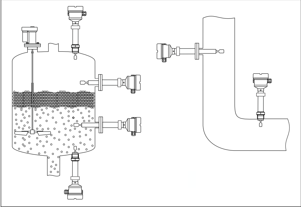
☞ 2 용기, 탱크 또는 배관에 설치 예
