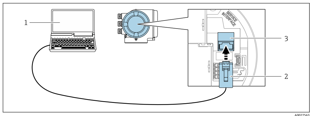
图 31 通过服务接口 (CDI-RJ45) 连接
