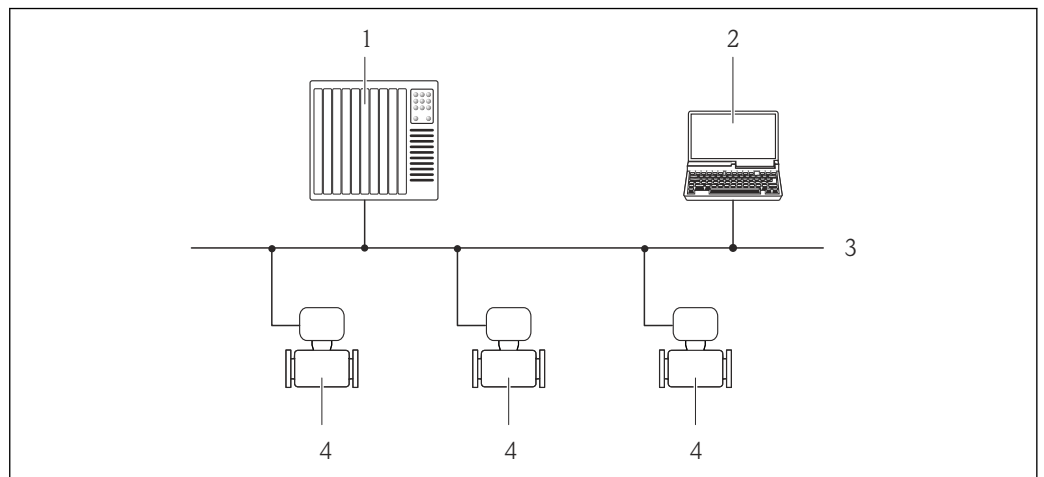
图 29 通过 PROFIBUS DP 网络进行远程操作
