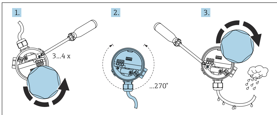
14 Hus med låseskruer; dann en dryppsløyfe på kabelen
