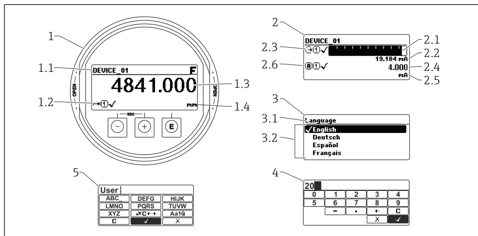
18 Formato de indicación en el módulo indicador y de configuración
