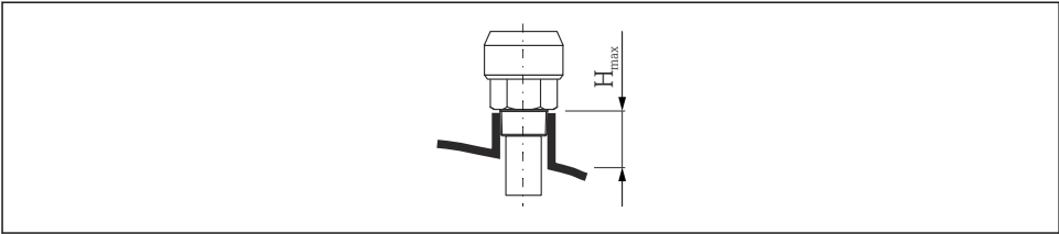
2 Altura de la tubuladura con antena de bocina encapsulada (FMR50); H_{m\acute{a}x} = 60\text{ mm} (2,36 in)
