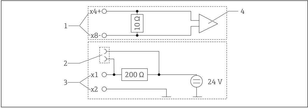
3 Circuiterie interne des douilles de raccordement HART® 1 Entrée courant 2 Douilles de raccordement HART® 3 Alimentation par boucle 4 Convertisseur A/N
