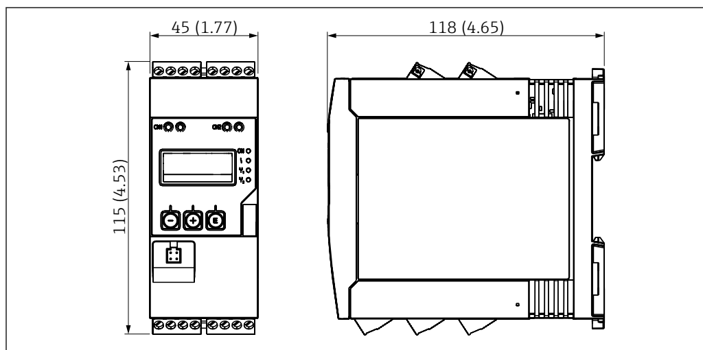
16 Dimensions du transmetteur de process en mm (in)
