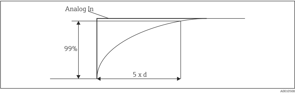
13 Amortissement du signal Analog In : Signal d'entrée analogique d : Réglage de l'amortissement
