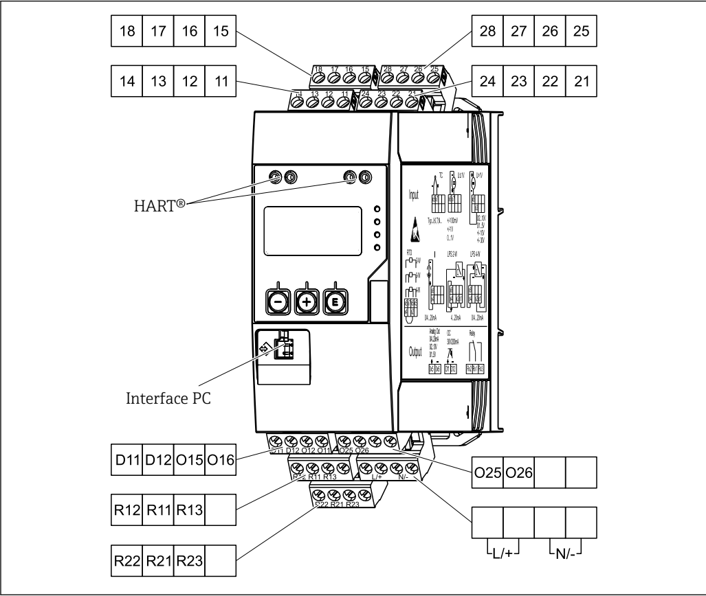
2 Affectation des bornes du transmetteur de process (voie 2 et relais en option)
