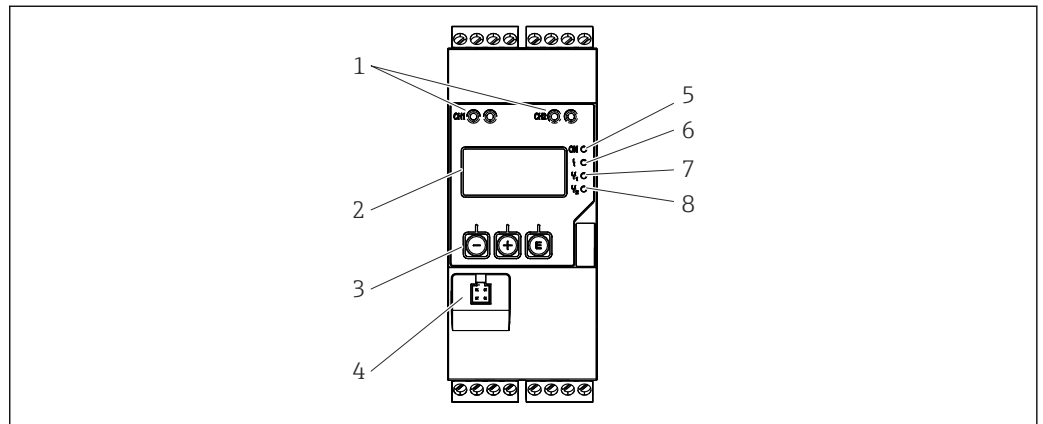
■ 17 Éléments d'affichage et de configuration du transmetteur de process
