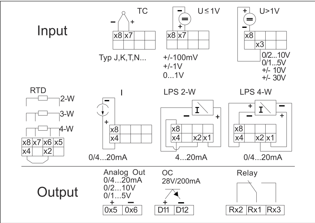
15 Affectation des bornes du transmetteur de process (relais (bornes Rx1-Rx3) et voie 2 (bornes 21-28 et 025/026) en option). Remarque : Position de contact illustrée des relais en cas de panne de l'alimentation électrique.
