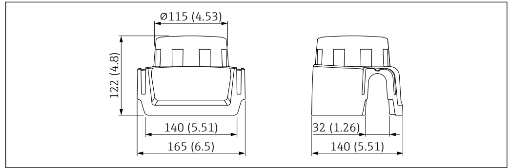
图 24 防护罩，适用单腔体铝外壳。测量单位 mm (in)
