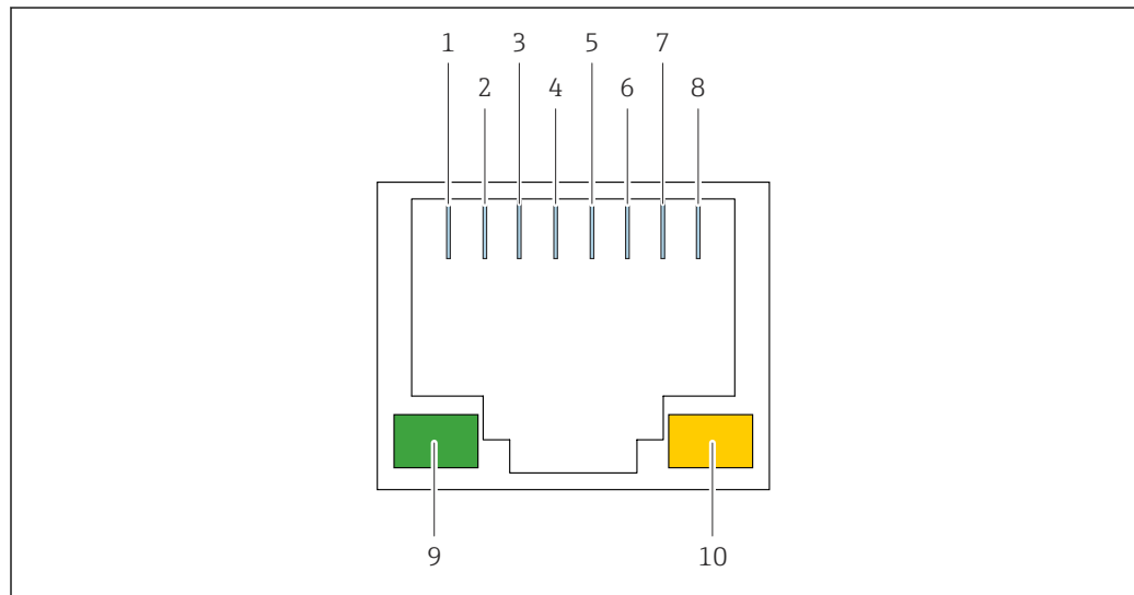
4 Affectation des broches des prises RJ45 et description des LED
