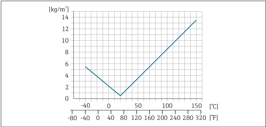
36 Ajuste da densidade de campo, por exemplo, a +20 °C (+68 °F)
