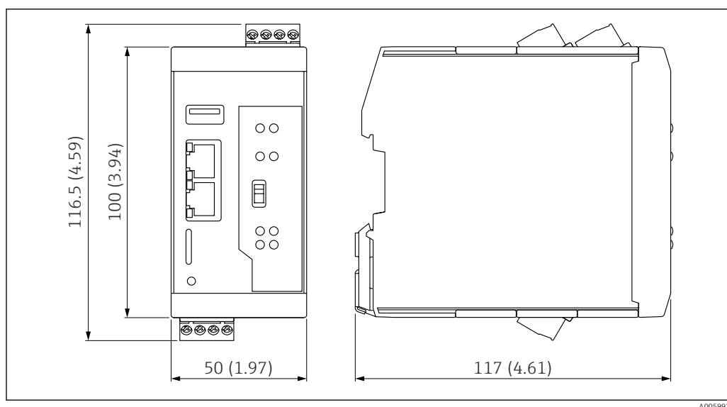
35 Dimensions. Unité de mesure mm (in)
