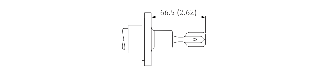
29 DRD. Unité de mesure mm (in)
