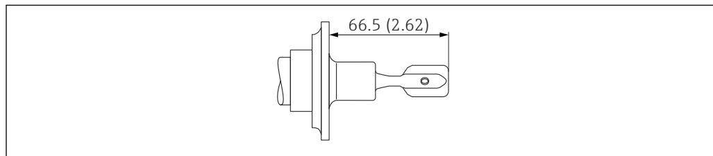
30 Raccord de conduite SMS 1145. Unité de mesure mm (in)
