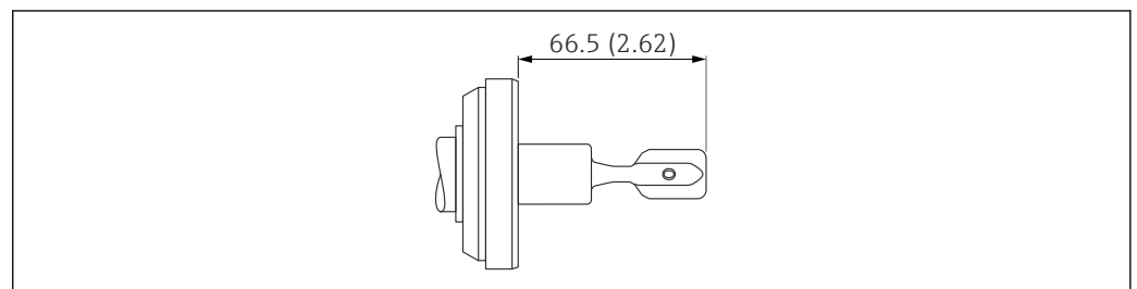
28 Raccord de conduite DIN 11864-1. Unité de mesure mm (in)
