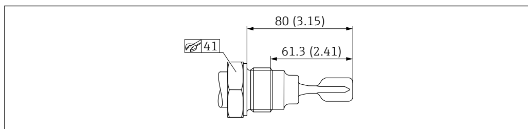
24 Filetage ISO228 G 1. Unité de mesure mm (in)
