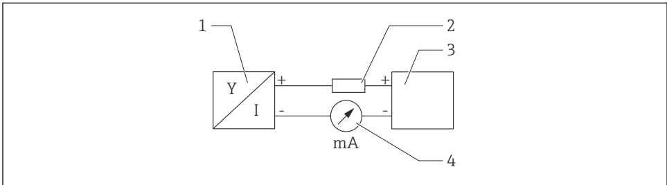
1 HART 接続のブロック図
