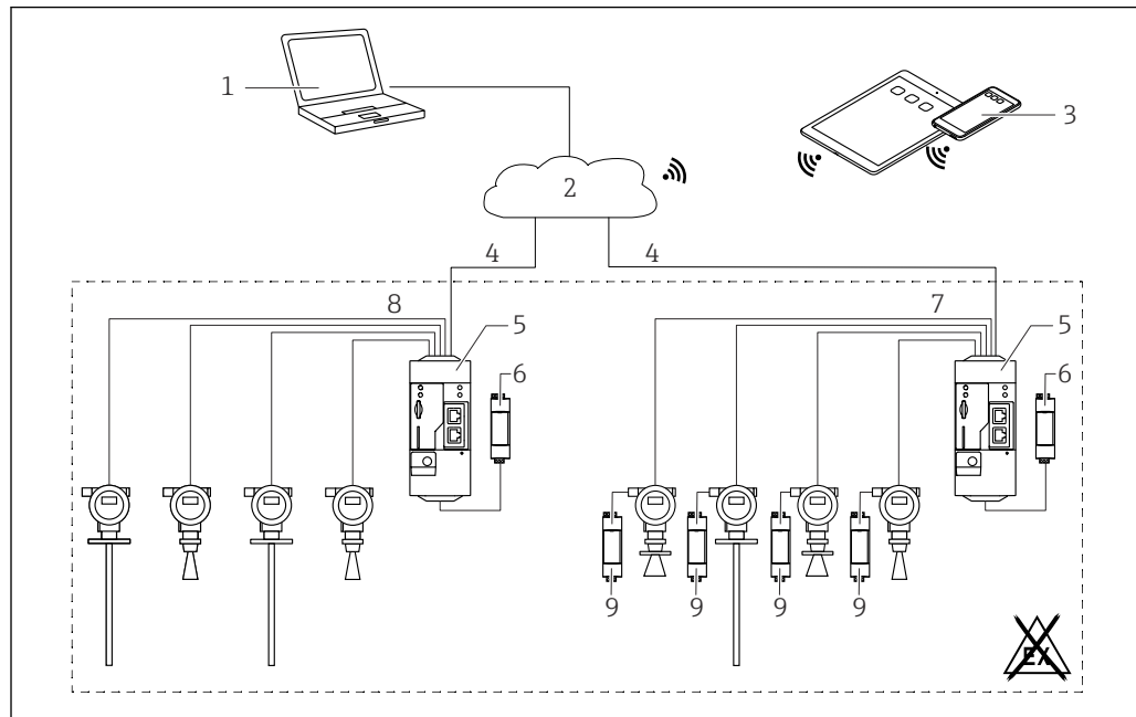
3 Arquitetura de sistema de um Fieldgate FXA42 com entrada analógica 4 para 20 mA
