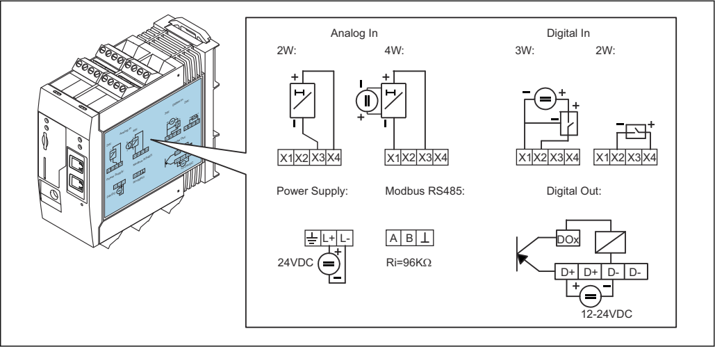
8 Identificação do invólucro para esquema de ligação elétrica
