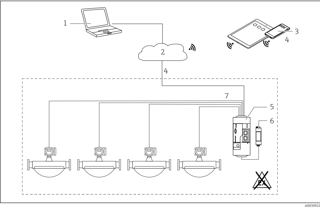
5 Arquitetura de sistema de um Fieldgate FXA42 com um contador de pulsos
