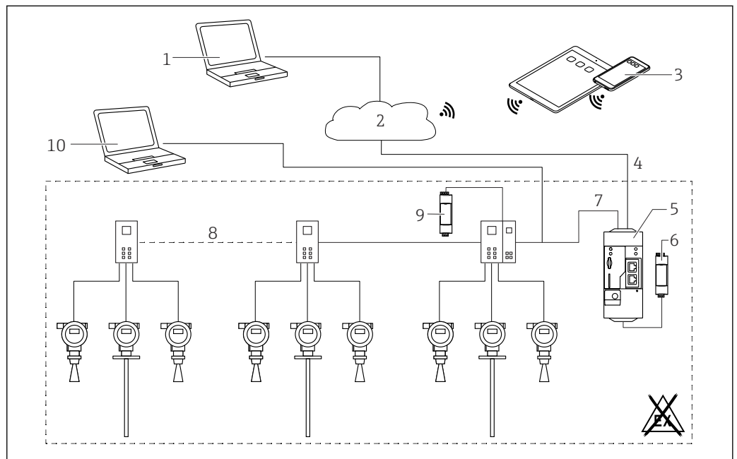
6 Arquitetura de sistema de um Fieldgate FXA42 com multiplexador HART ponto-a-ponto
