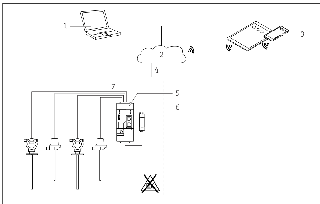
4 Arquitetura de sistema de um Fieldgate FXA42 com uma entrada digital
