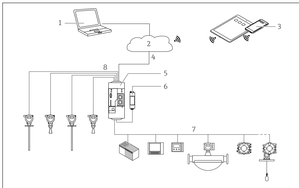
7 Arquitetura do sistema de um Fieldgate FXA42 com Modbus RS485
