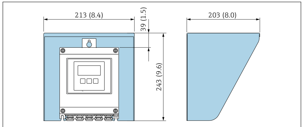
19 Cubierta protectora para Proline 500, digital; unidad: mm (in)
