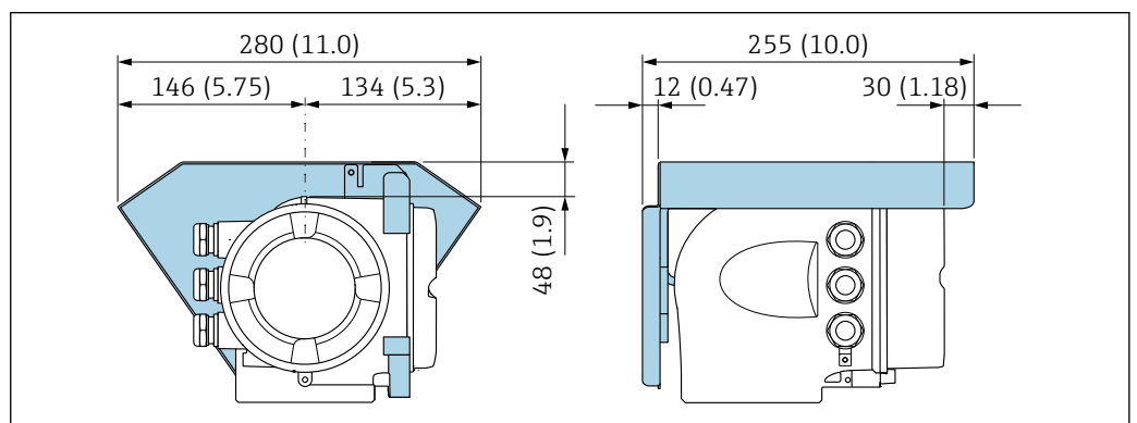
20 Cubierta protectora para Proline 500; unidad: mm (in)
