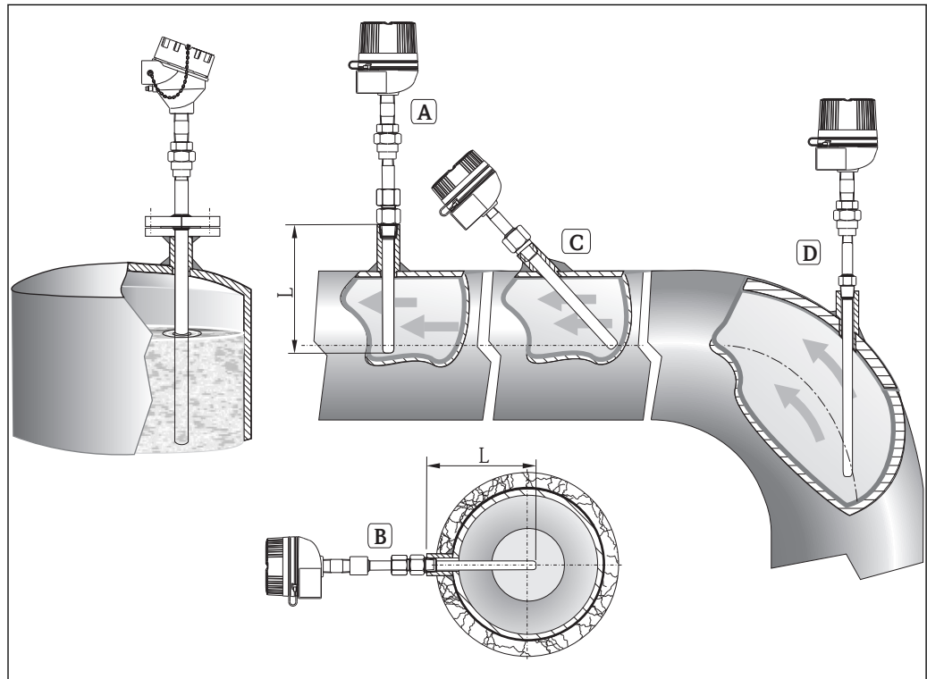
5 Installationsbeispiele
