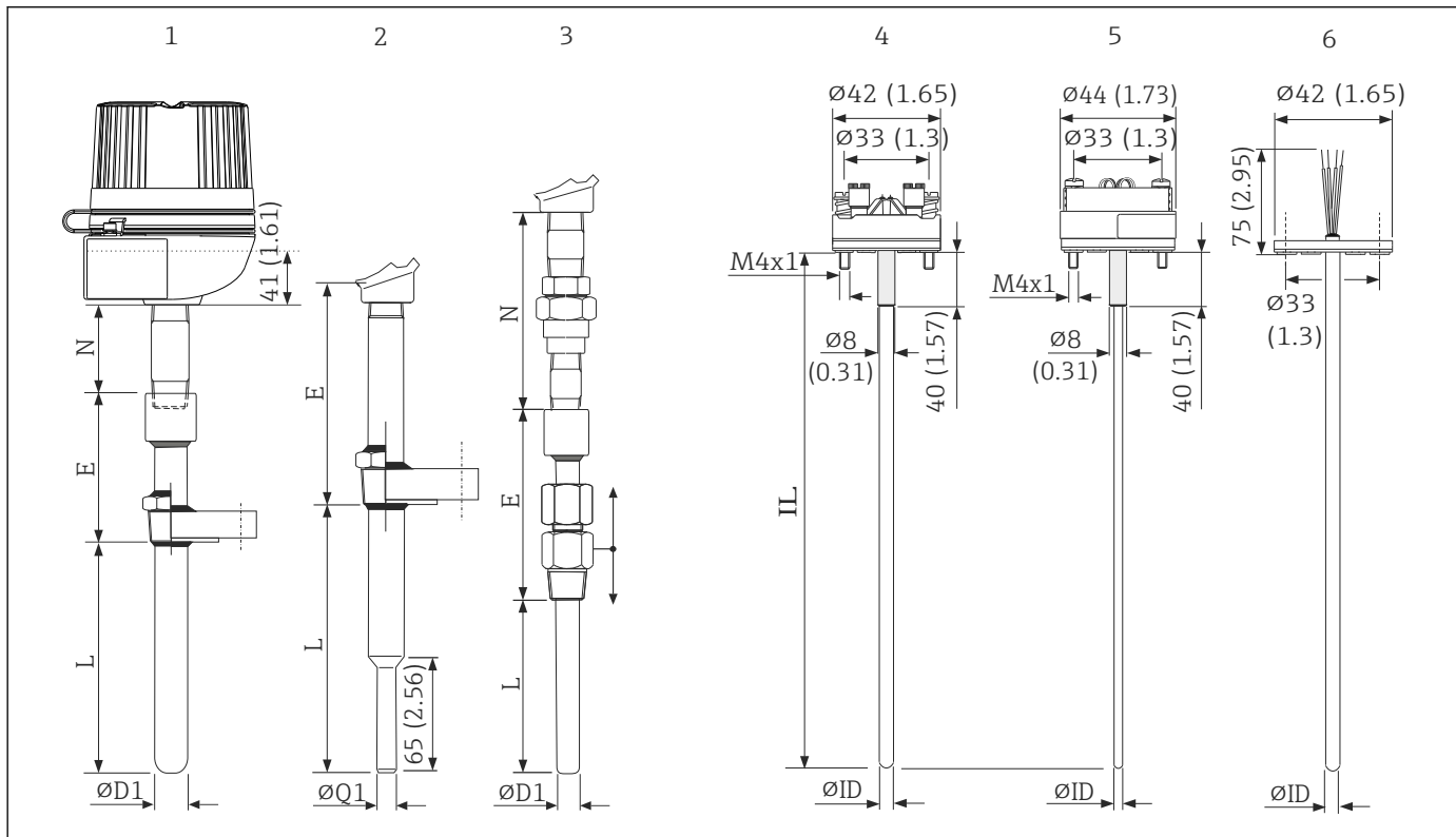
4 Abmessungen Omnigrad S TR63 und TC63
