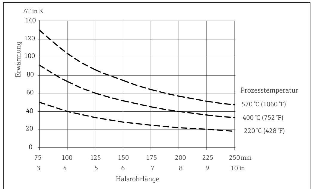
6 Erwärmung des Anschlusskopfes in Abhängigkeit von der Prozesstemperatur. Temperatur im Anschlusskopf = Umgebungstemperatur 20 °C (68 °F) + ΔT
