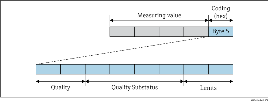
30 Estrutura do byte de codificação
