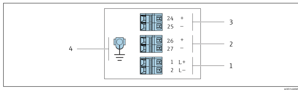
2 Klemmenbelegung 4-20 mA HART mit Impuls-/Frequenz-/Schaltausgang
