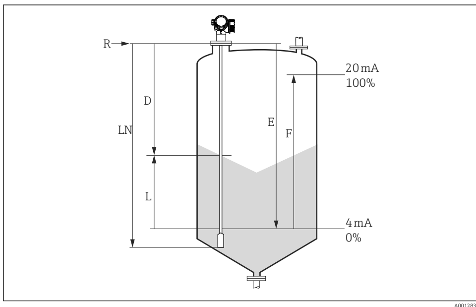
10 Parâmetros de configuração para as medições de nível em sólidos a granel
