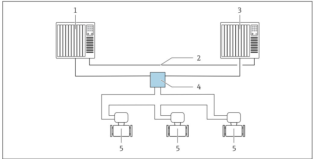
33 Пример компоновки резервируемой системы (S2): кольцевая топология
