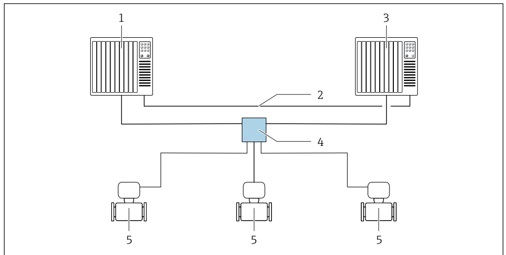
34 Пример компоновки резервируемой системы (S2): топология «звезда»
