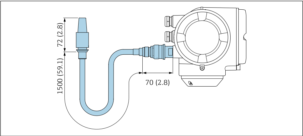
36 単位 mm (in)
