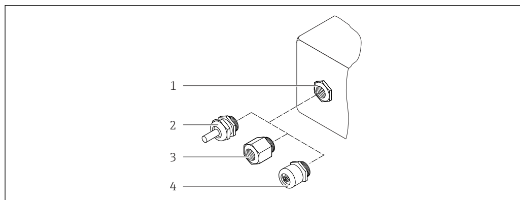
図 37 可能な電線口/ケーブルグランド
