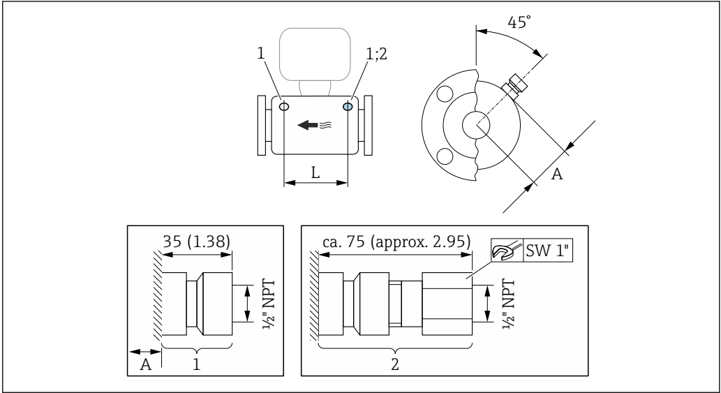
27 単位 mm (in)
