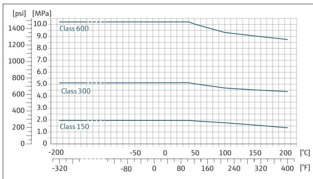
図 19 フランジ材質 1.4404 (SUS F316 相当または SUS F316L 相当)
