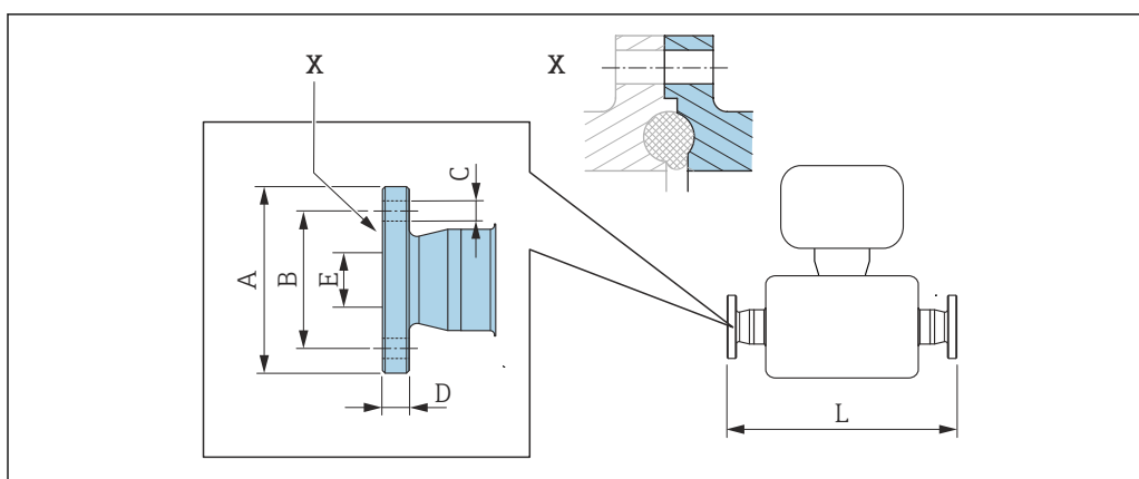
図 26 X の詳細：非対称型プロセス接続；青色部分が供給されます。
