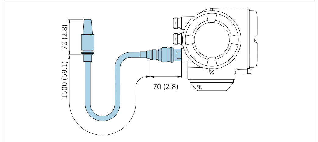
31 単位 mm (in)
