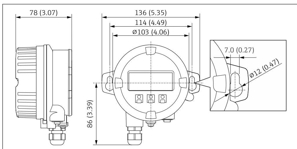
図 29 単位 mm (in)
