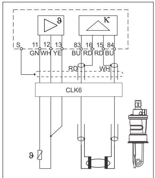
11 Connessione dei sensori induttivi
