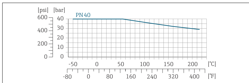
18 Flange da junta de lapela com material do flange: 1.4301 (F304), partes úmidas Liga C22: 2.4602 (UNS N06022)
