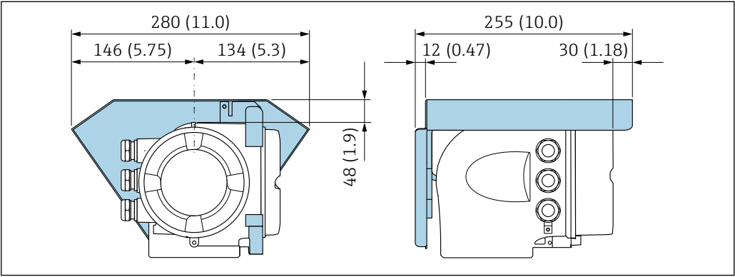
14 Unidade em mm (pol.)
