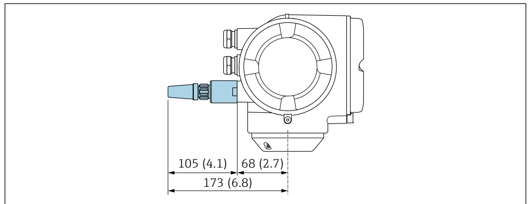
30 Unidade em mm (pol.)
