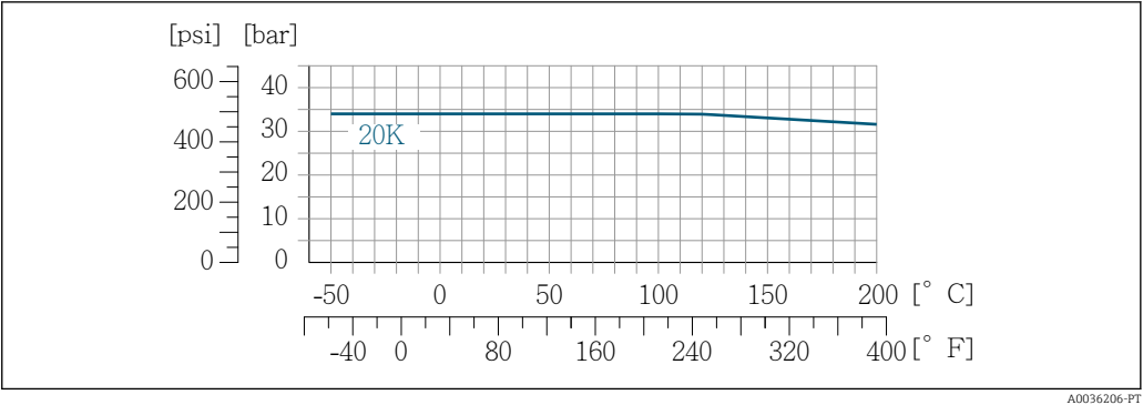
23 Flange da junta de lapela com material do flange: 1.4301 (F304), partes úmidas Liga C22: 2.4602 (UNS N06022)
