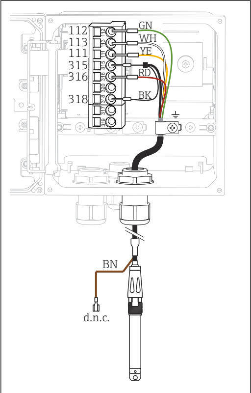
32 变送器的内部结构示意图（传感器模块）
