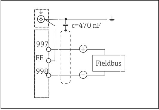
图 19 接线图
