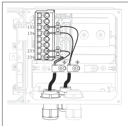
图 14 变送器的内部结构示意图 (CPU 模块)
