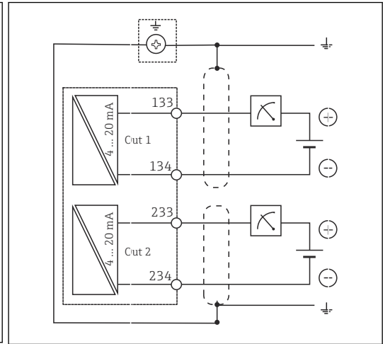
图 13 接线图
