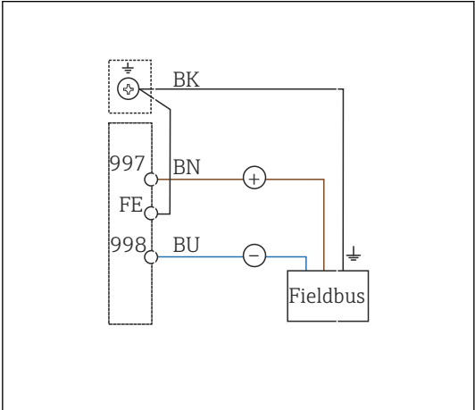
图 21 接线图
