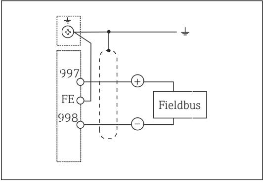
图 17 接线图
