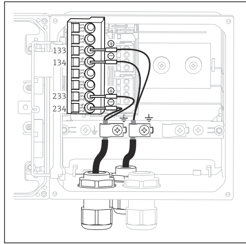
图 12 变送器的内部结构示意图 (CPU 模块)
