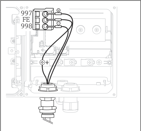
图 20 变送器的内部结构示意图 (CPU 模块)
