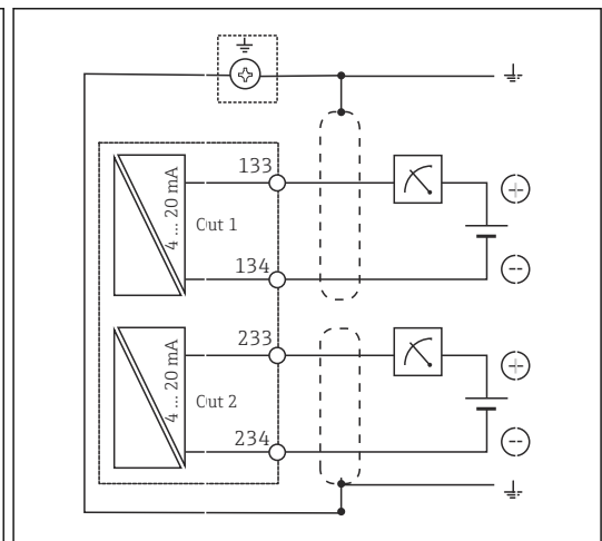
图 15 接线图
