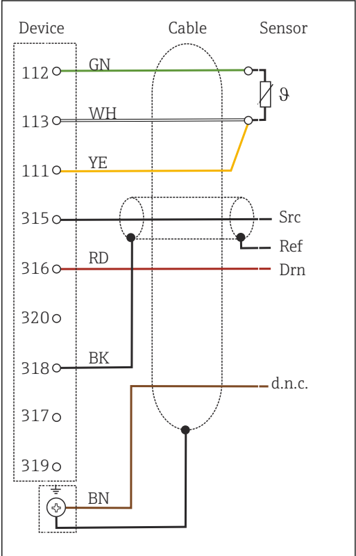
33 接线图
