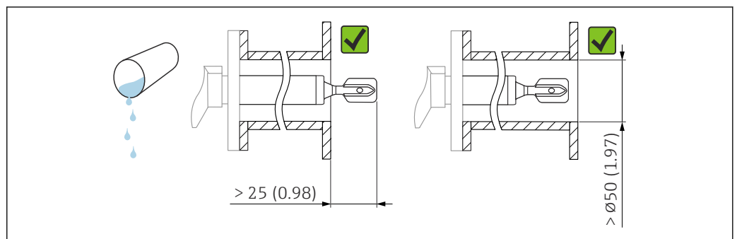
图 7 安装实例：测量低粘度液体。测量单位 mm (in)
