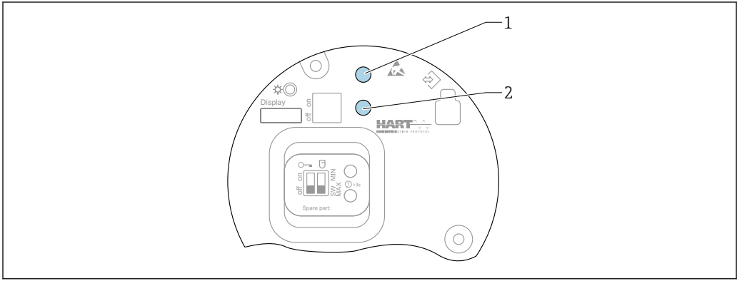
📖 30 FEL60H 电子插件上的操作按键 1+2 同时按下：复位设备的操作按键（恢复出厂状态）
