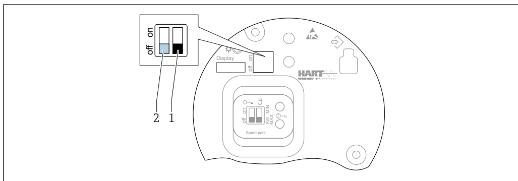
图 29 FEL60H 电子插件上的 DIP 开关的功能
