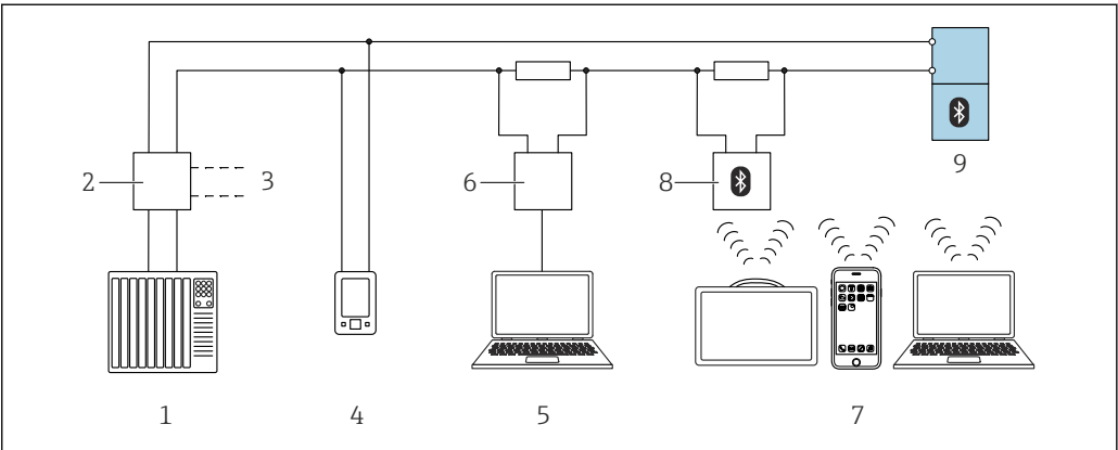
图 27 通过 HART 通信实现远程操作
