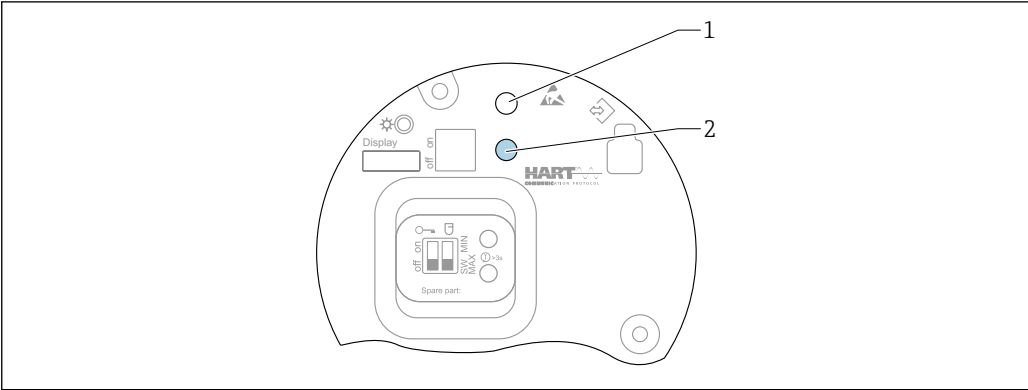
图 23 FEL60H 电子插件上的操作按键 1 操作按键，用于重置密码 2 操作按键，用于执行功能安全测试 (> 3 s)
