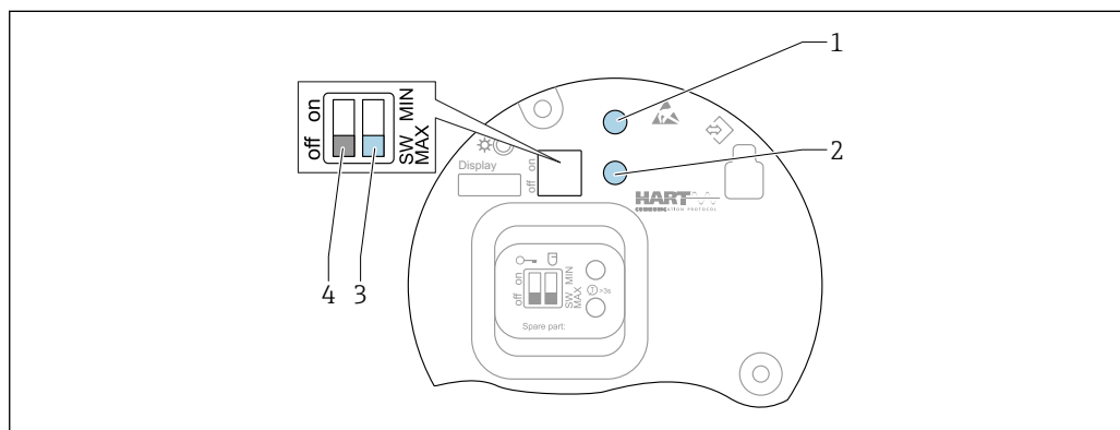
图 28 FEL60H 电子插件上的操作按键和 DIP 开关
