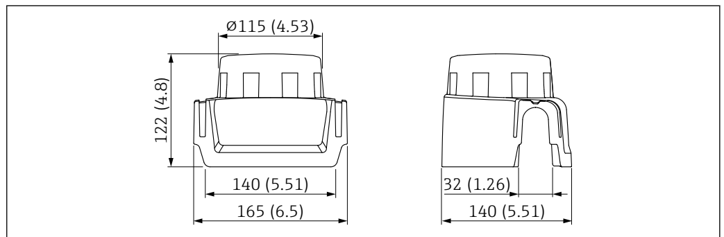
图 32 塑料防护罩 XW111 的外形尺寸示意图。测量单位 mm (in)
