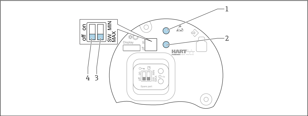
图 22 FEL60H 电子插件上的操作按钮和 DIP 开关
