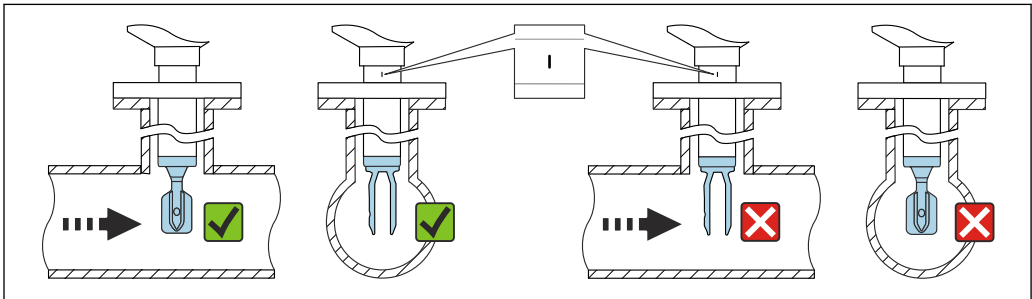
13 安装在管道中（注意叉体安装位置和标记）
