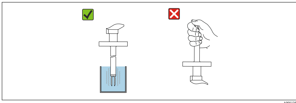
图 26 音叉的功能测试
