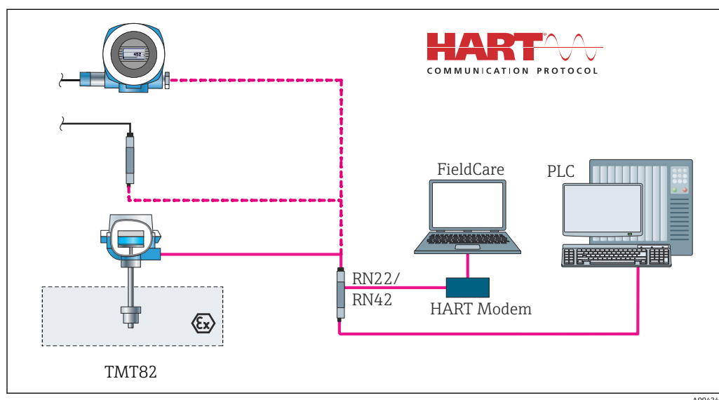
図 2 HART 通信用の機器構成
