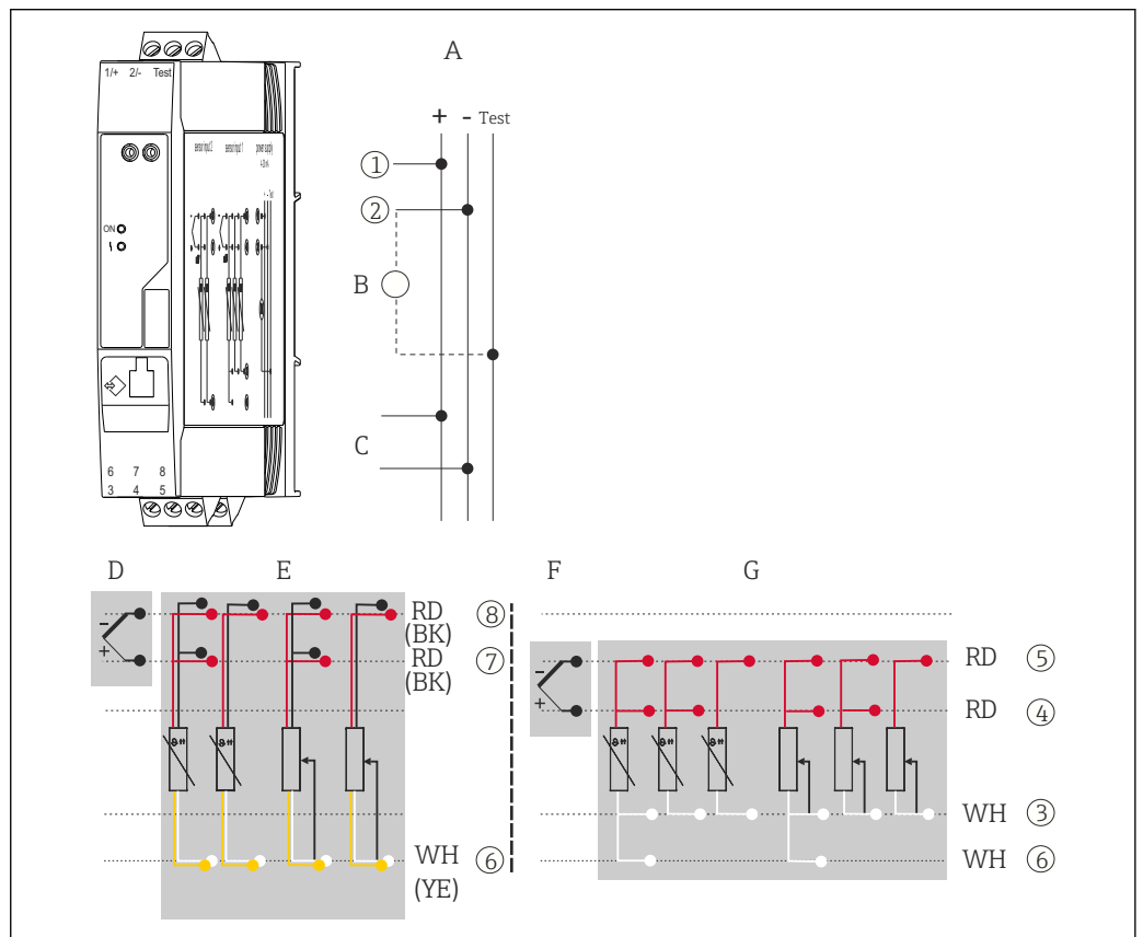
図 4 DIN レール用伝送器の接続端子の割当て
