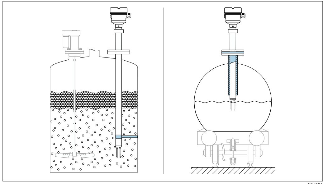
图 16 实例：存在动态负载时，应支撑设备
