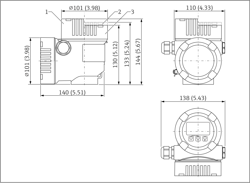
图 22 L 型双腔室铝外壳（带涂层）的外形尺寸示意图；包括 M20 接头和塑料插头。测量单位 mm (in) 1 带玻璃观察窗的盖板高度（适用 Ex d/XP 和粉尘防爆仪表） 2 带塑料观察窗的盖板高度 3 不带观察窗的盖板高度
