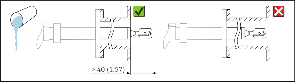
8 安装实例：测量高粘度液体。测量单位 mm (in)
