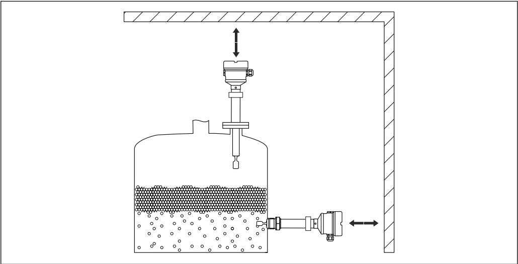
10 预留安装间隙
