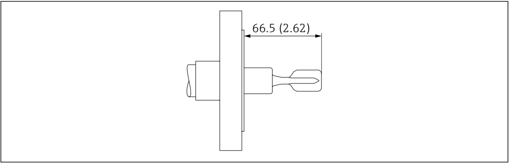
35 法兰连接型传感器示意图。测量单位 mm (in)
