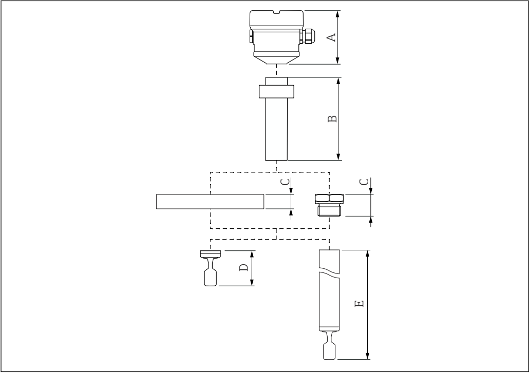
图 18 计算设备高度所需考虑的部件 A 外壳，含外壳盖 B 隔热管（带玻璃气密锁通）→可选 2 种长度，取决于过程温度 C 过程连接 D 探头类型：一体式，带音叉 E 探头类型：延长管型，带音叉
