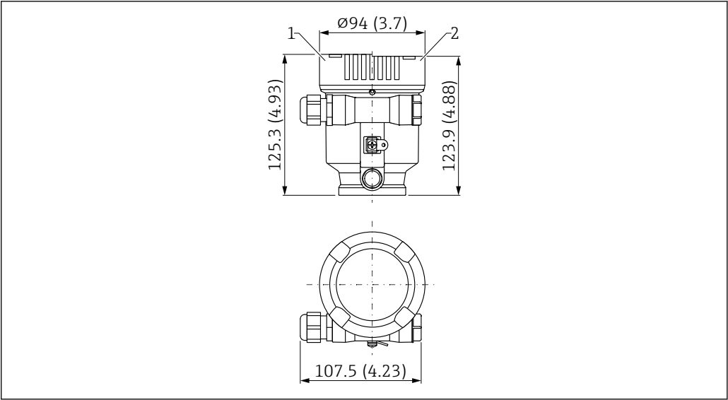
19 单腔室塑料外壳的外形尺寸示意图；包括 M20 接头和塑料插头。测量单位 mm (in)
