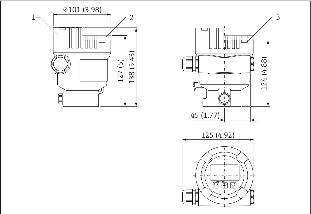
20 单腔体铝外壳（带涂层）的外形尺寸示意图。测量单位 mm (in)
