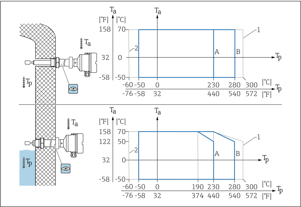
图 17 外壳允许环境温度 T_a 与罐体内部过程温度 T_p 的关系
