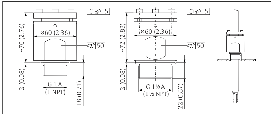
图 41 高压滑动套管。测量单位 mm (in)
