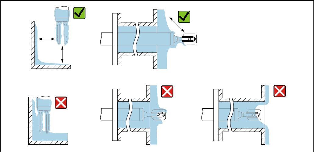
9 安装实例：测量高粘度过程介质
