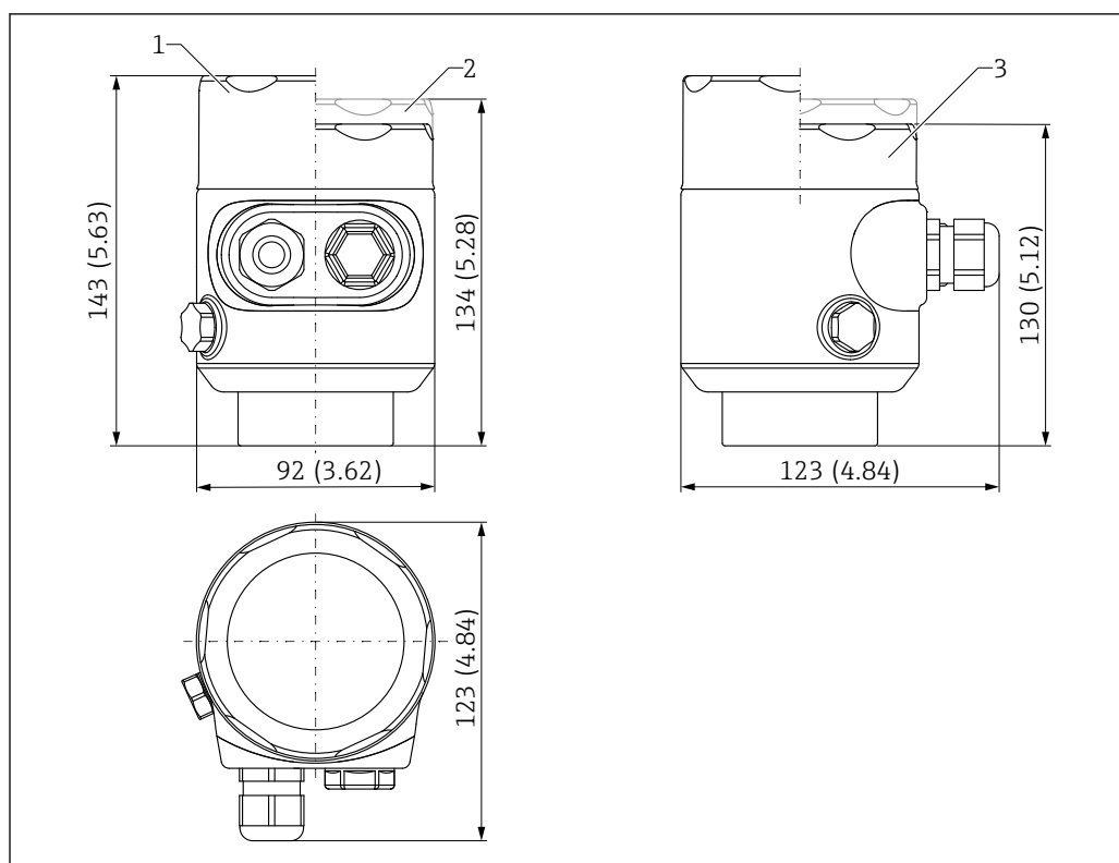
图 21 单腔体 316L 外壳（卫生型）的外形尺寸示意图。测量单位 mm (in)
