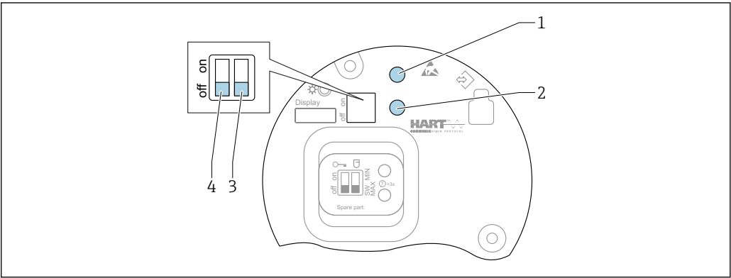
图 36 FEL60H 电子插件上的操作按键和 DIP 开关
