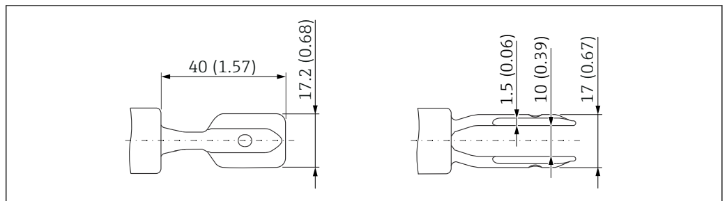
图 27 叉体。测量单位 mm (in)
