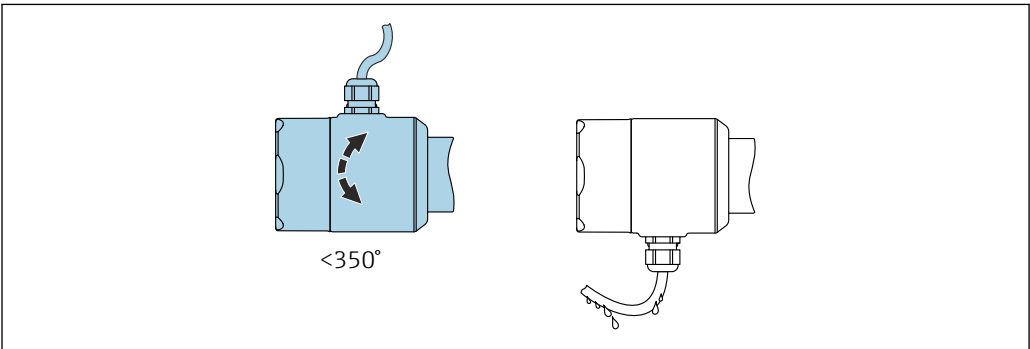
图 13 外壳不带锁紧螺丝，带排水回路
