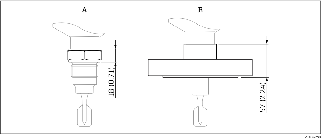
图 28 过程连接的最大高度规格
