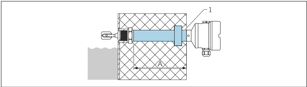
图 24 隔热管（带玻璃气密锁通）
