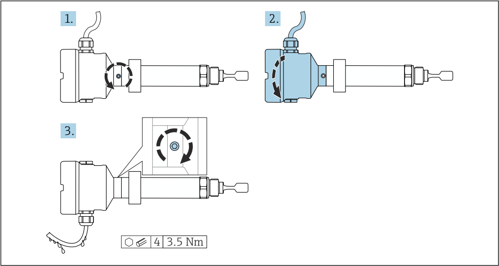
14 外壳带外部锁紧螺丝和排水回路
