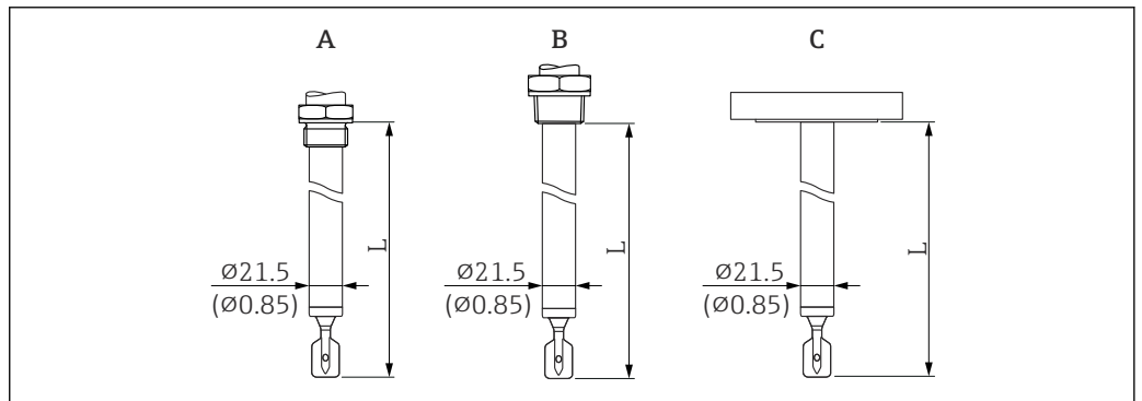
图 26 延长管型（传感器长度 L）。测量单位 mm (in)
