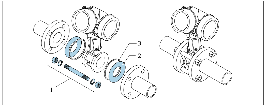
7 Kit di montaggio per versione wafer
