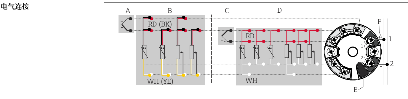
图 3 模块化温度变送器的接线端子分配
