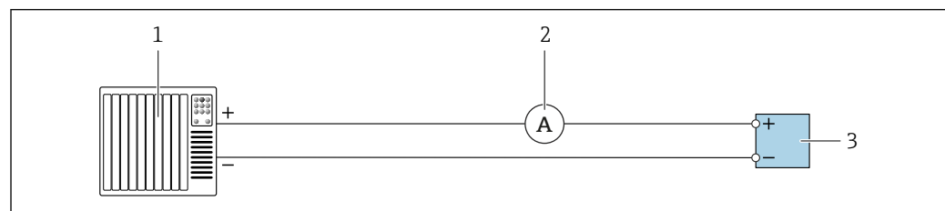
图 29 有源电流输出扩展校验
