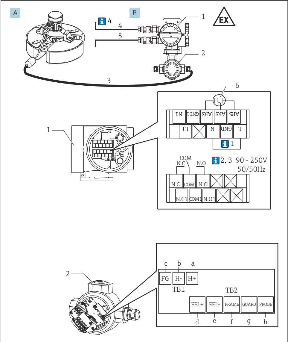
14 Ex d [ia] -muuntimen NRR261-4/A/B/C johdotus
