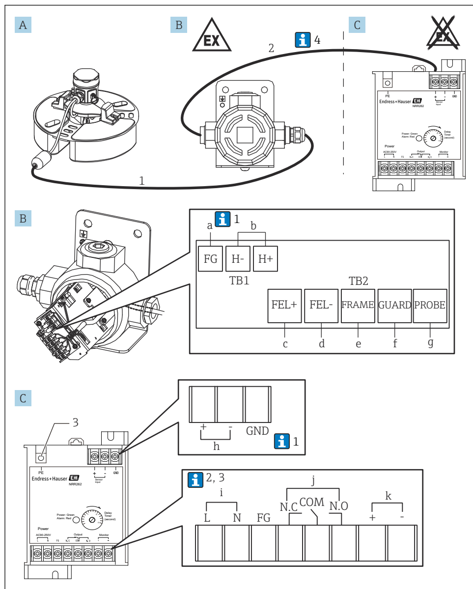
15 Ex [ia] -muuntimen NRR262-4/A/B/C johdotus
