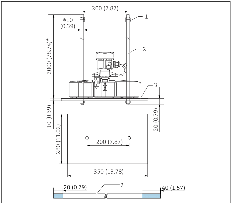
9 NAR300, uimuriohjain. Mittausyksikkö mm (in)
