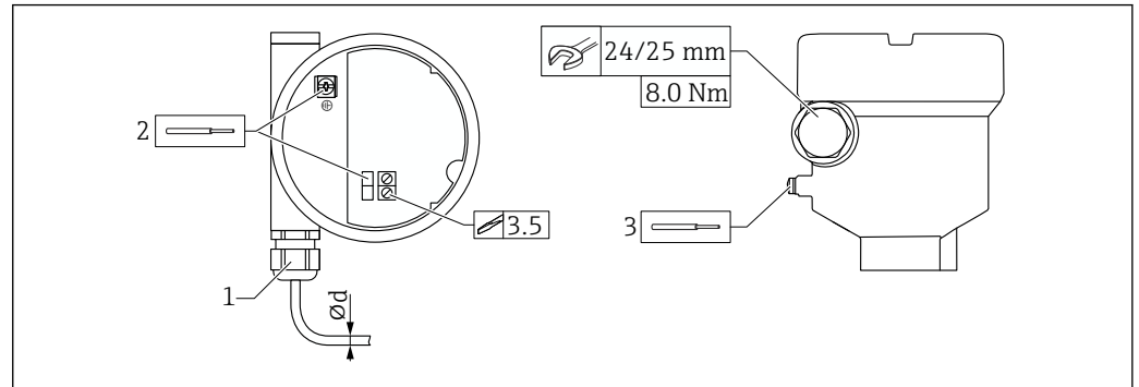
20 Exemple de presse-étoupe avec entrée de câble, électronique avec bornes
