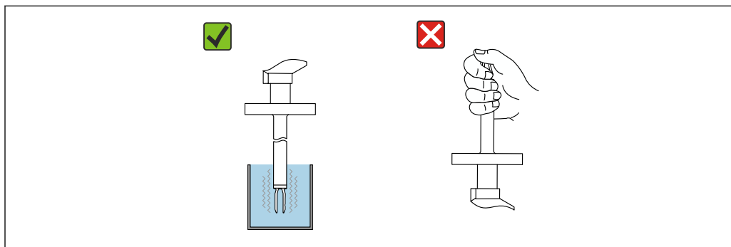
22 Test de fonctionnement de la fourche vibrante
