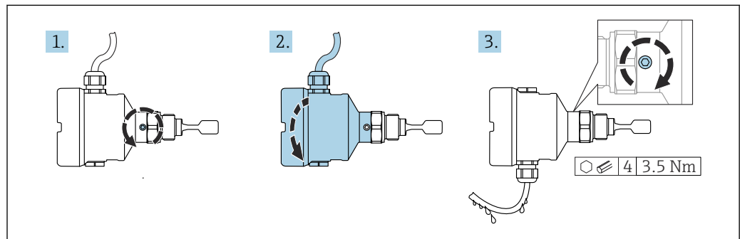
17 Boîtier avec vis de verrouillage externe ; former une boucle de drainage sur le câble
