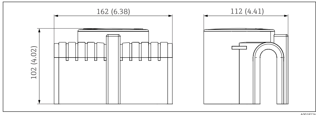
45 Dimensions du capot de protection climatique PA6. Unité de mesure mm (in)
