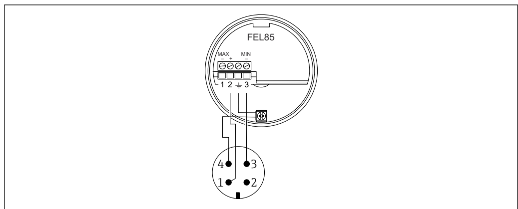
19 Affectation des bornes avec connecteur M12, mode de fonctionnement détection de minimum
