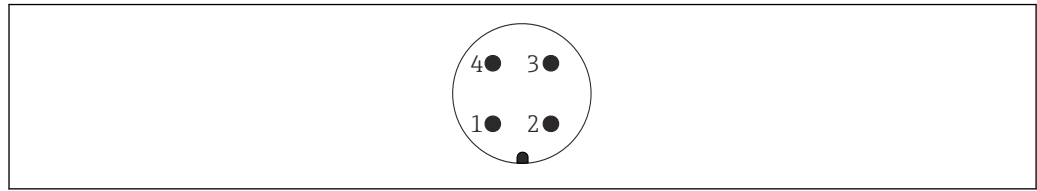
17 Connecteur M12, affectation des broches
