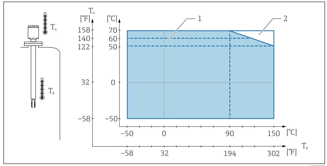
47 Température ambiante autorisée T_a au boîtier en fonction de la température de process T_p dans la cuve ; température maximale du process 150 °C (302 °F)
