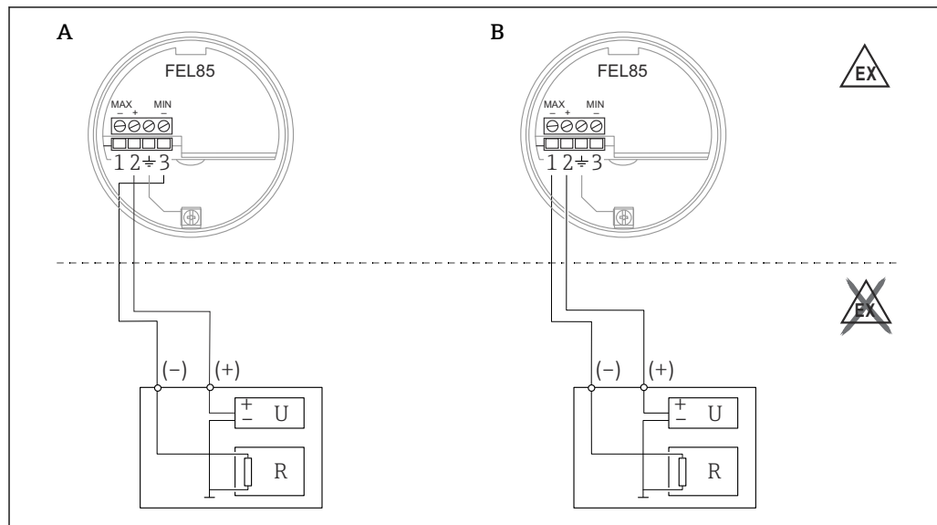
21 Raccordement à un API
