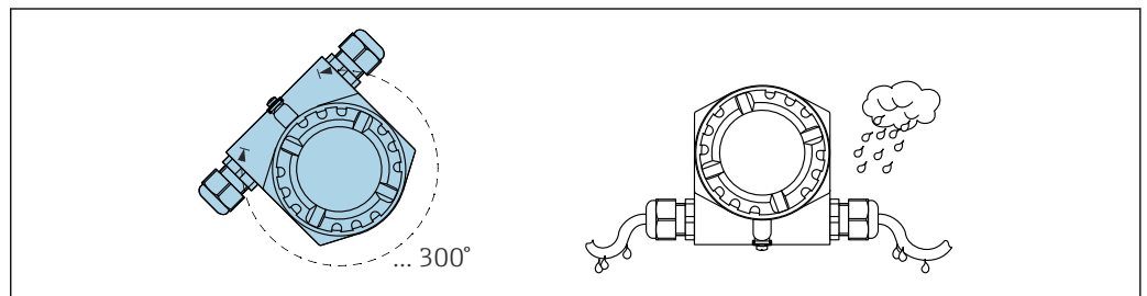
16 Boîtier sans vis de réglage ; former une boucle de drainage sur le câble
