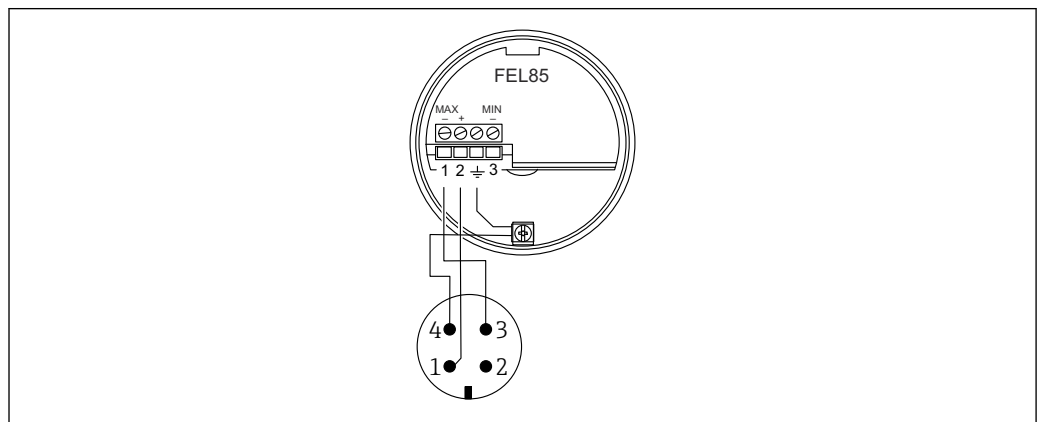
18 Affectation des bornes avec connecteur M12, mode de fonctionnement détection de maximum
