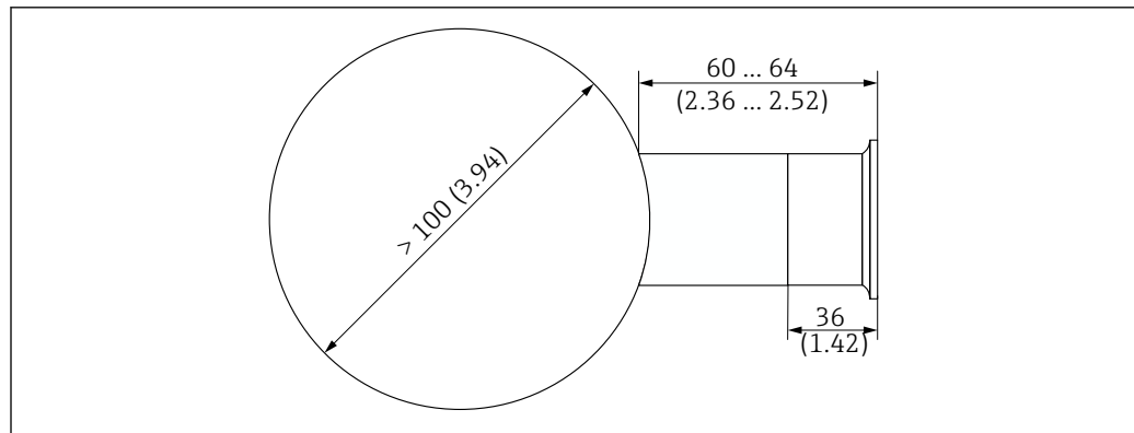
19 Connessione al tubo con adattatore a saldare. Unità: mm (in)
