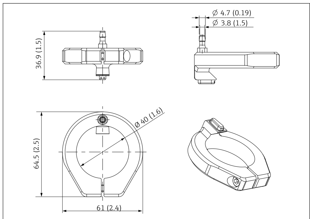
17 Dimensioni per la pulizia con aria compressa. Dimensioni: mm (in)
