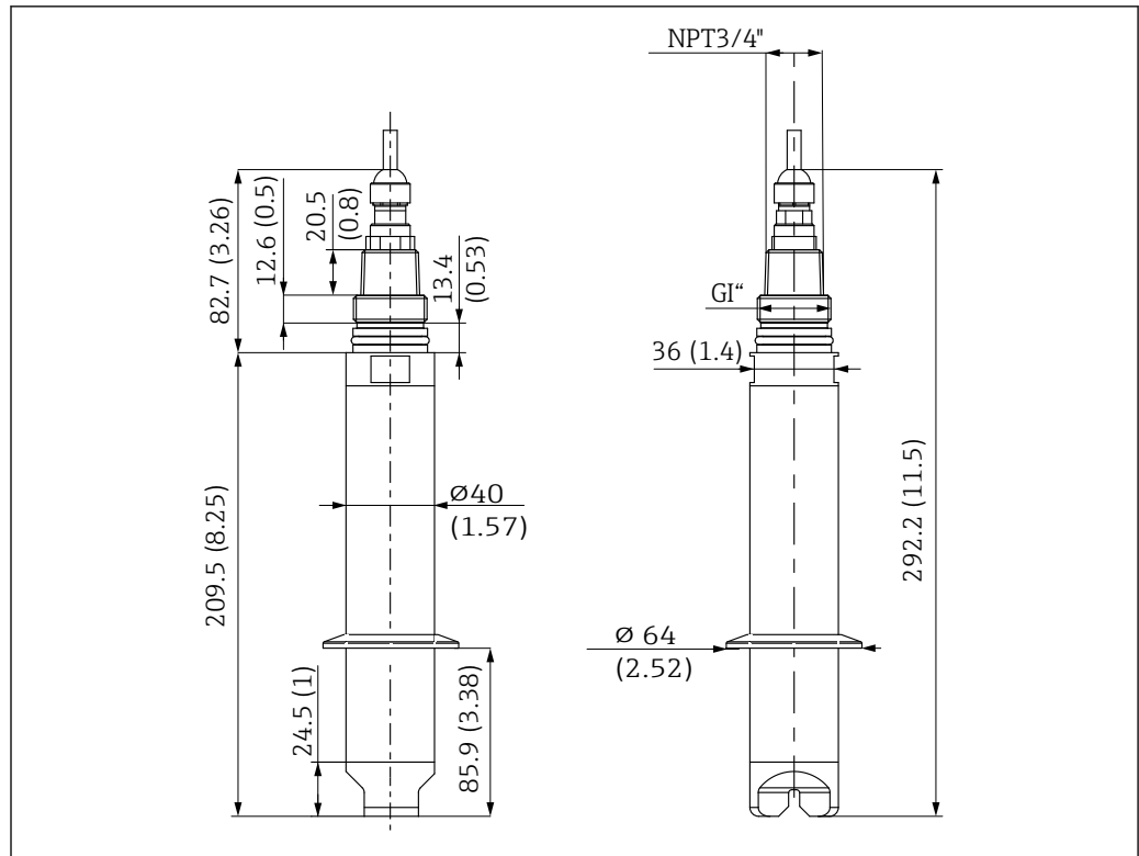
16 Dimensioni con clamp. Dimensioni: mm (in)
